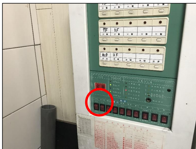
圖 3-48 受信總機如有異常燈號亮起（紅圈部分），應立即予以檢查並修正，圖為地區警鈴被關閉之狀態
