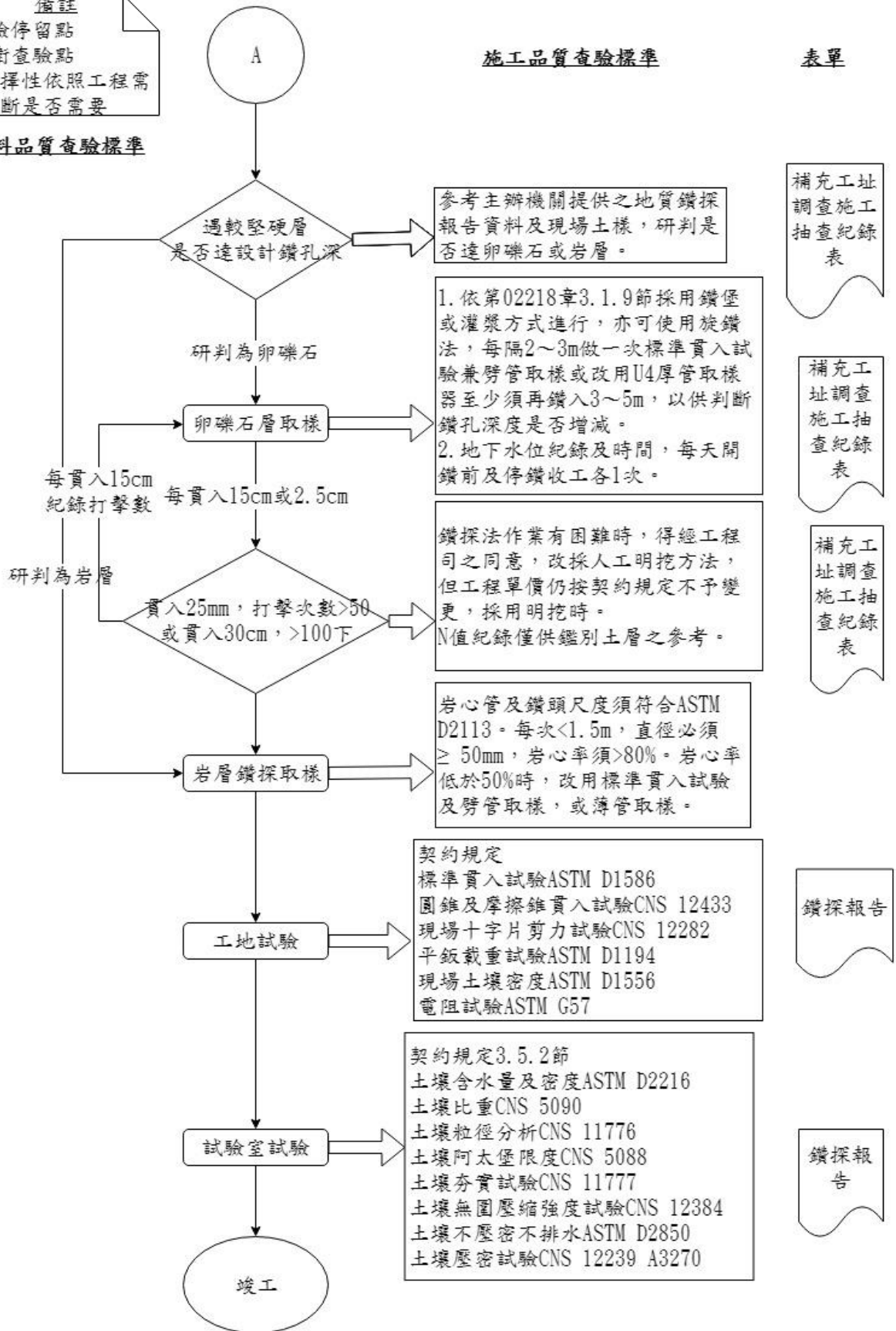
圖 022180-F-1 補充工址調查施工抽查流程圖 2/2
