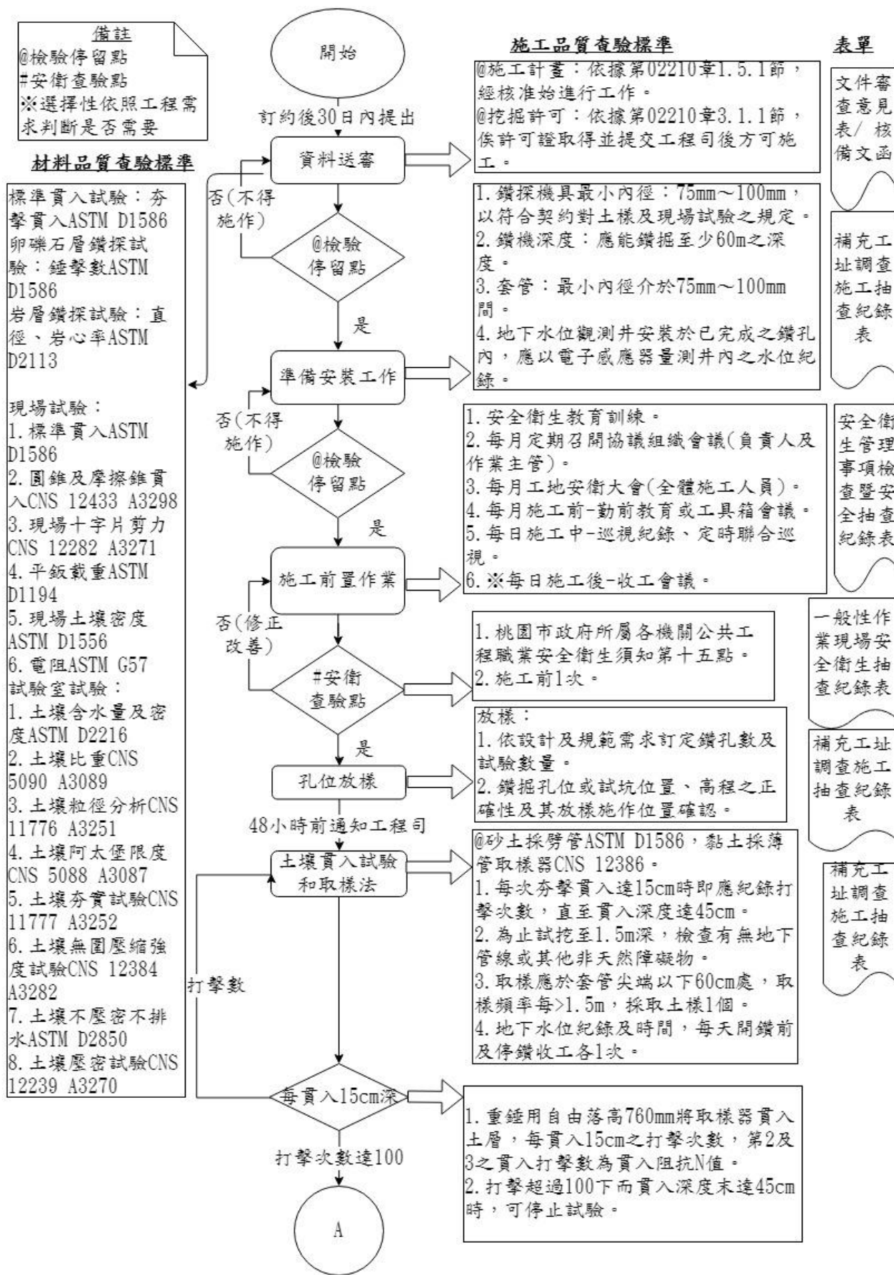
圖 022180-F-1 補充工址調查施工抽查流程圖 1/2
