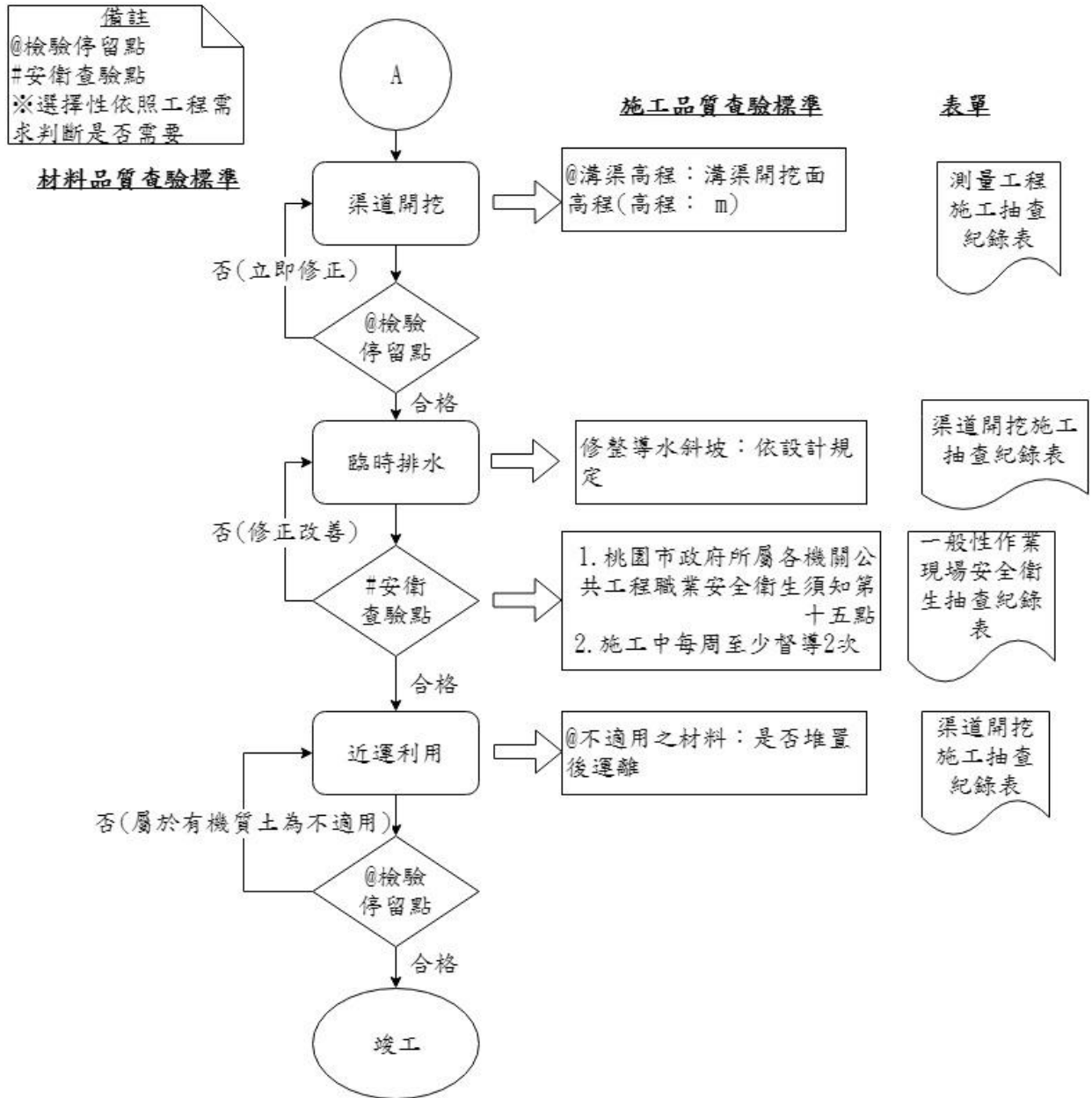
圖 023180-F-1 渠道開挖施工抽查流程圖 2/2
