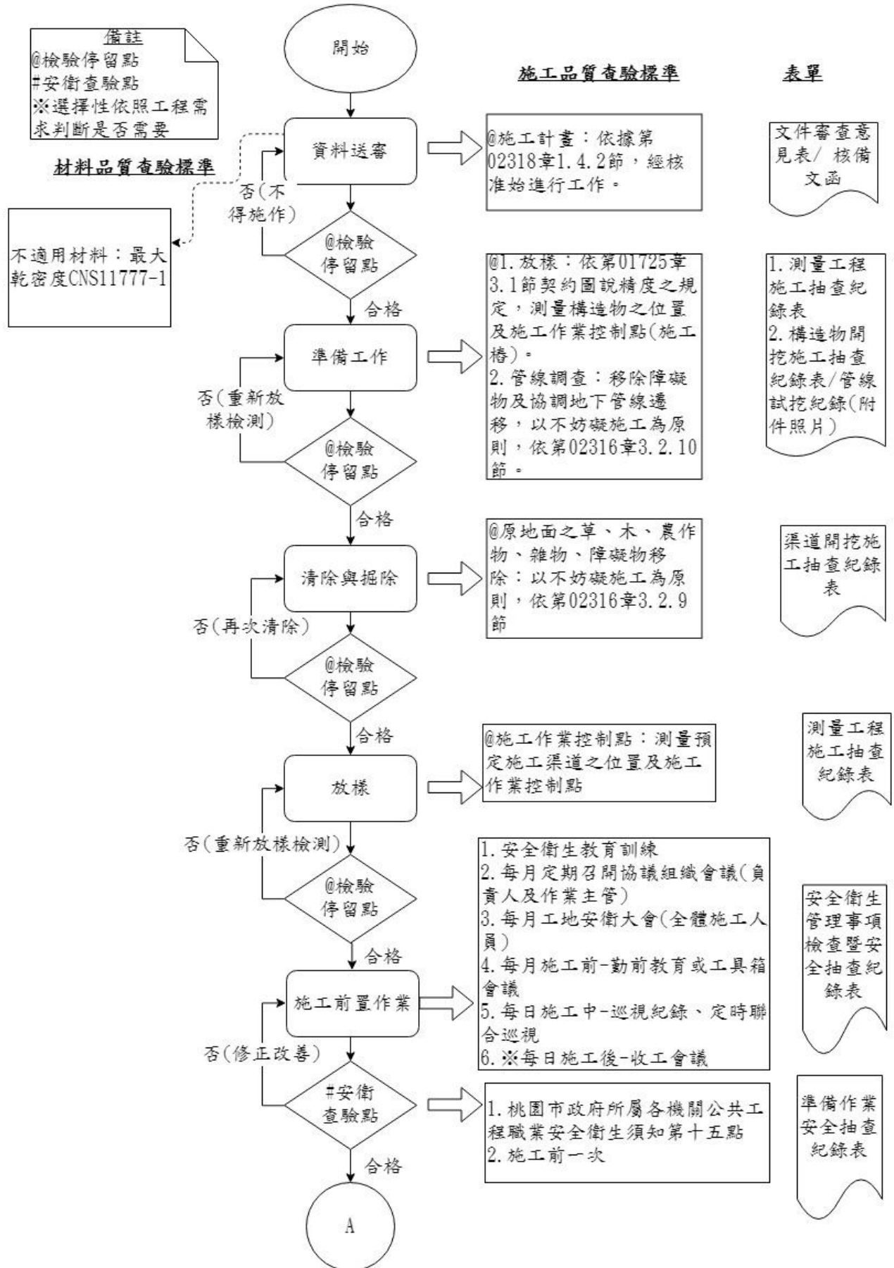
圖 023180-F-1 渠道開挖施工抽查流程圖 1/2
