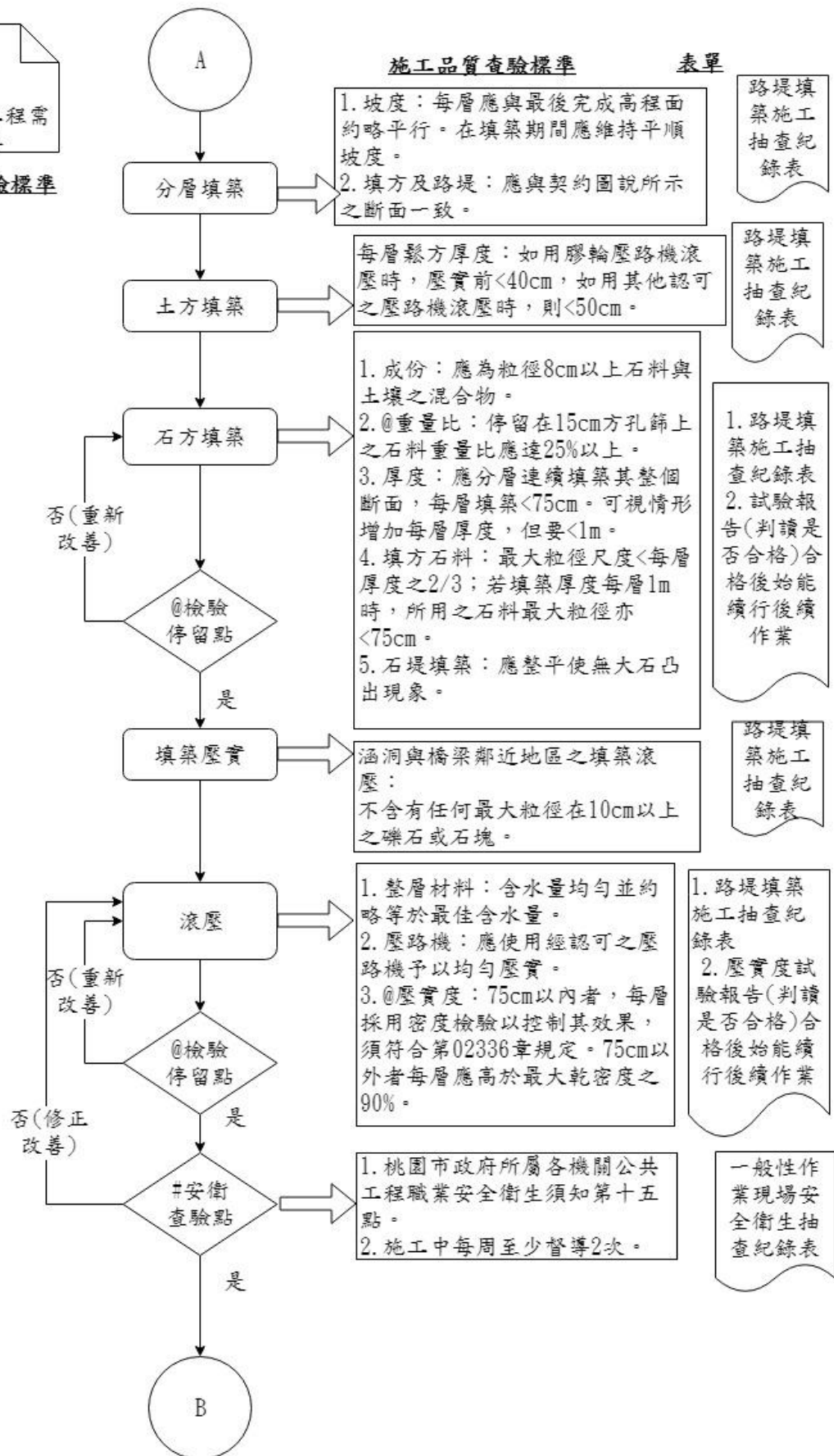
圖 023310-F-1 路堤填築施工抽查流程圖 2/3
