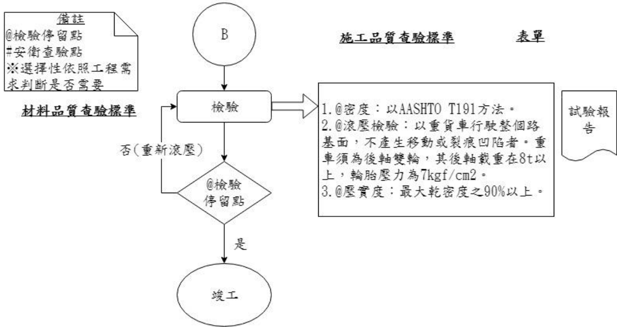
圖 023310-F-1 路堤填築施工抽查流程圖 3/3
