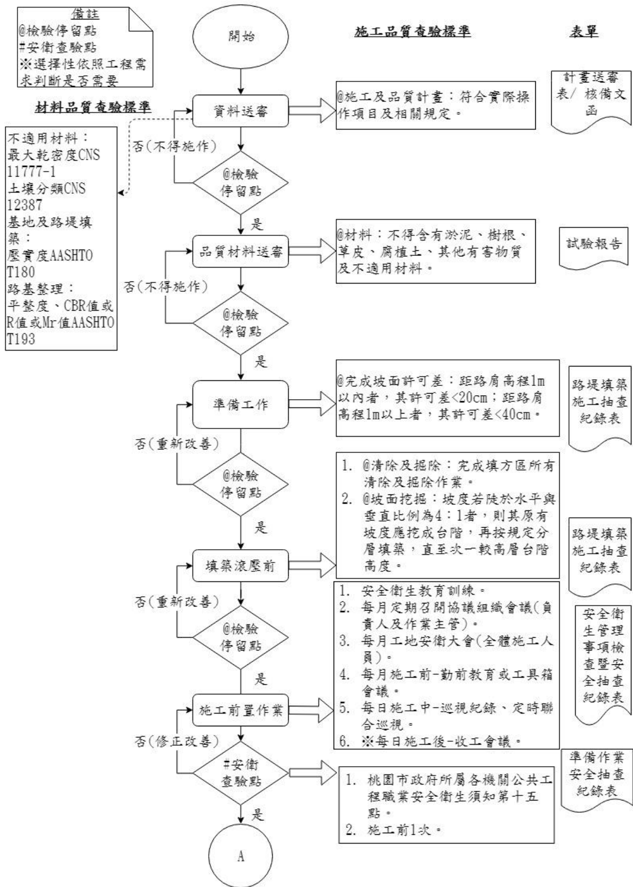
圖 023310-F-1 路堤填築施工抽查流程圖 1/3
