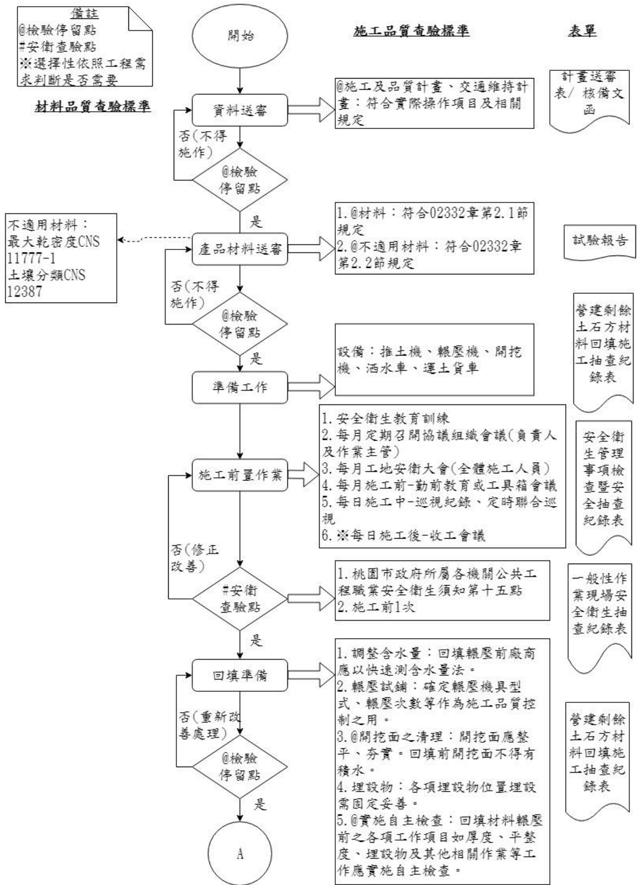
圖 023320-F-1 營建剩餘土石方材料回填施工抽查流程圖 1/3
