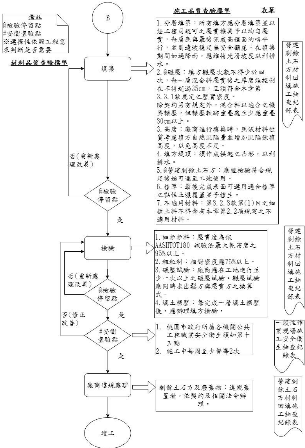
圖 023320-F-1 營建剩餘土石方材料回填施工抽查流程圖 3/3
