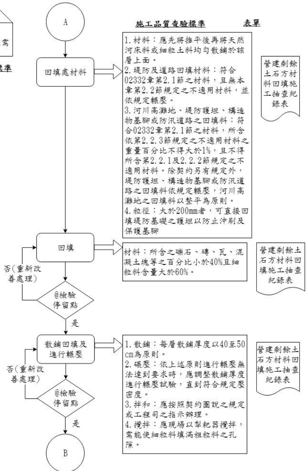
圖 023320-F-1 營建剩餘土石方材料回填施工抽查流程圖 2/3
