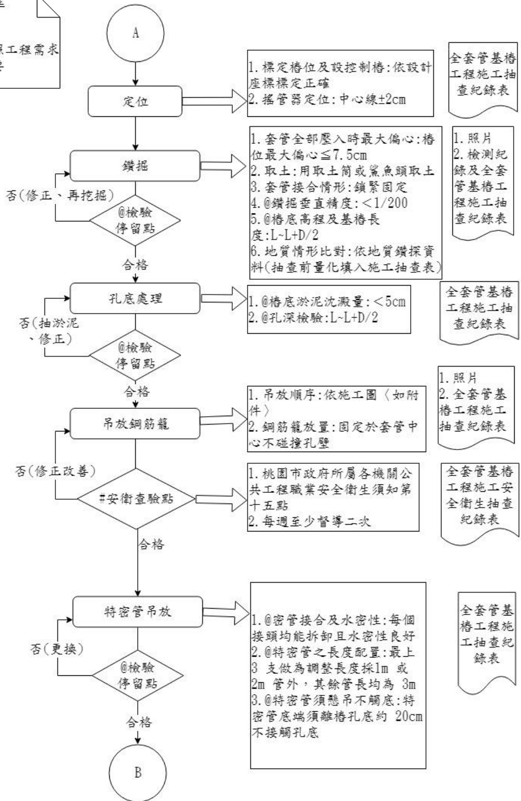
圖 024690-F-1 全套管基樁工程施工抽查流程圖 2/3
