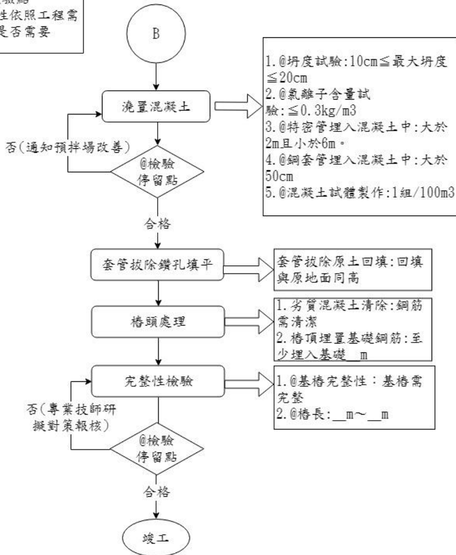
圖 024690-F-1 全套管基樁工程施工抽查流程圖 3/3
