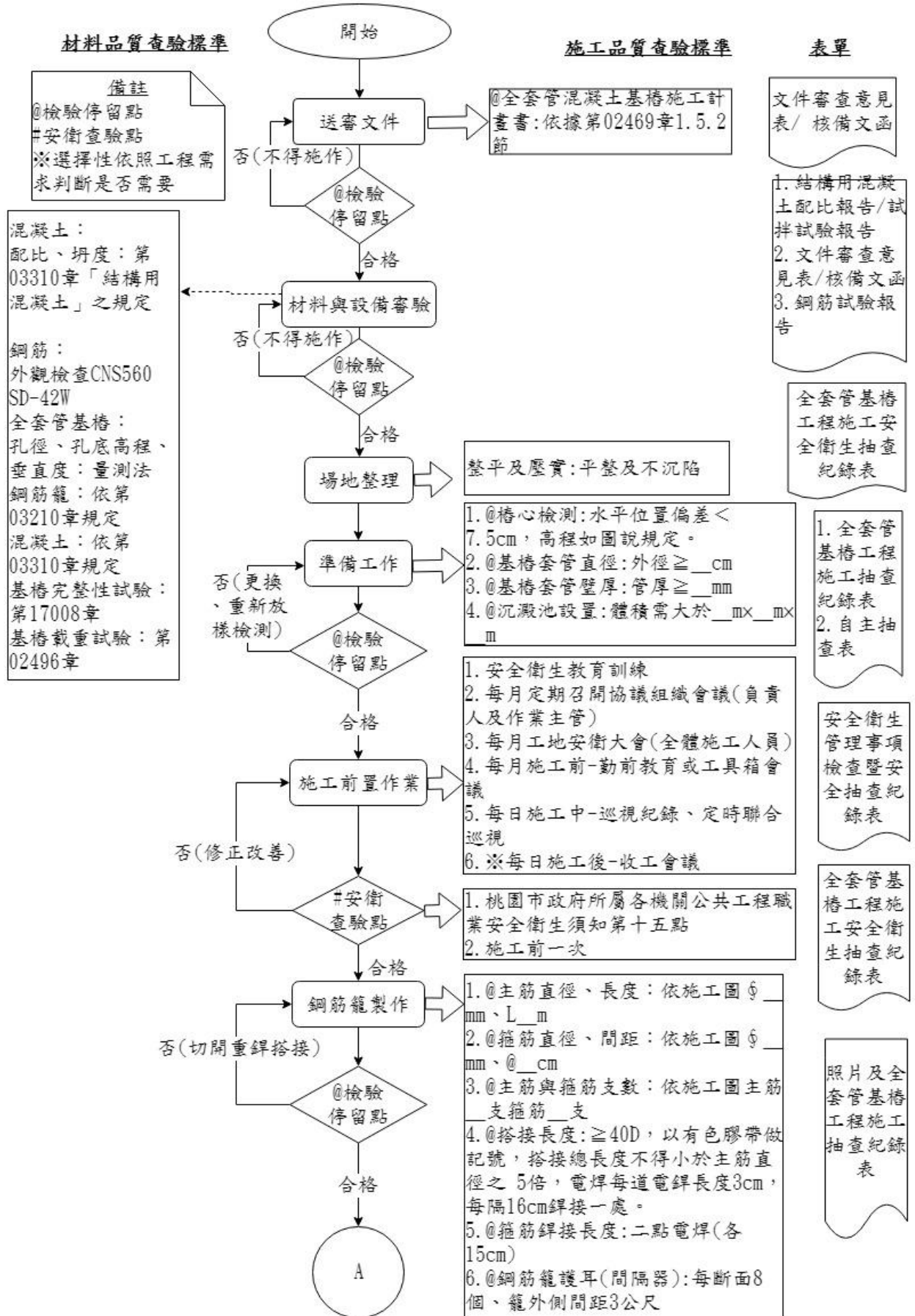
圖 024690-F-1 全套管基樁工程施工抽查流程圖 1/3
