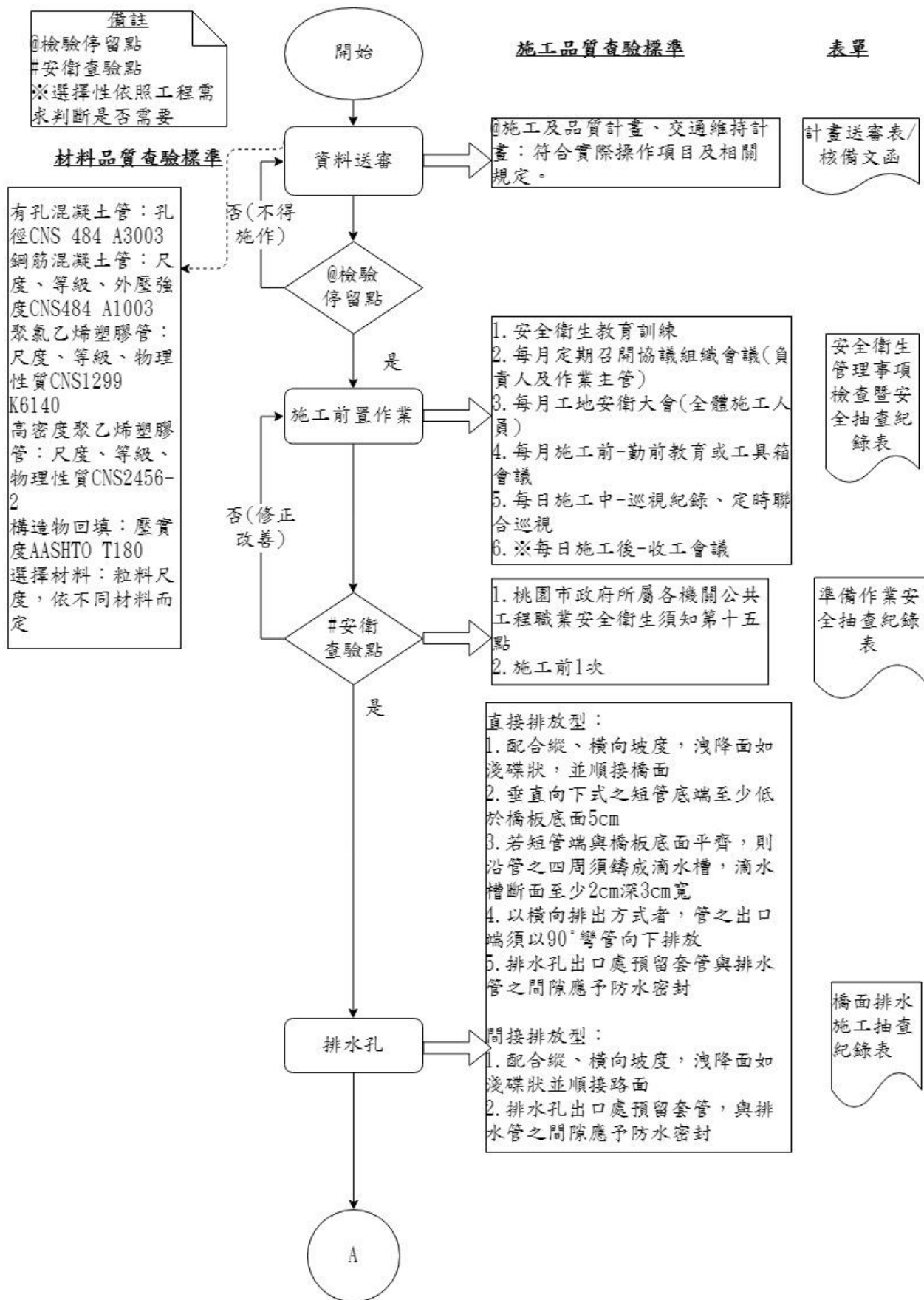
圖 026390-F-1 橋面排水施工抽查流程圖 1/2
