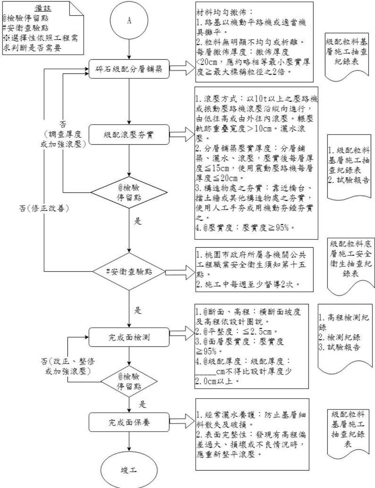
圖 027220-F-1 級配粒料基層施工抽查流程圖 2/2
