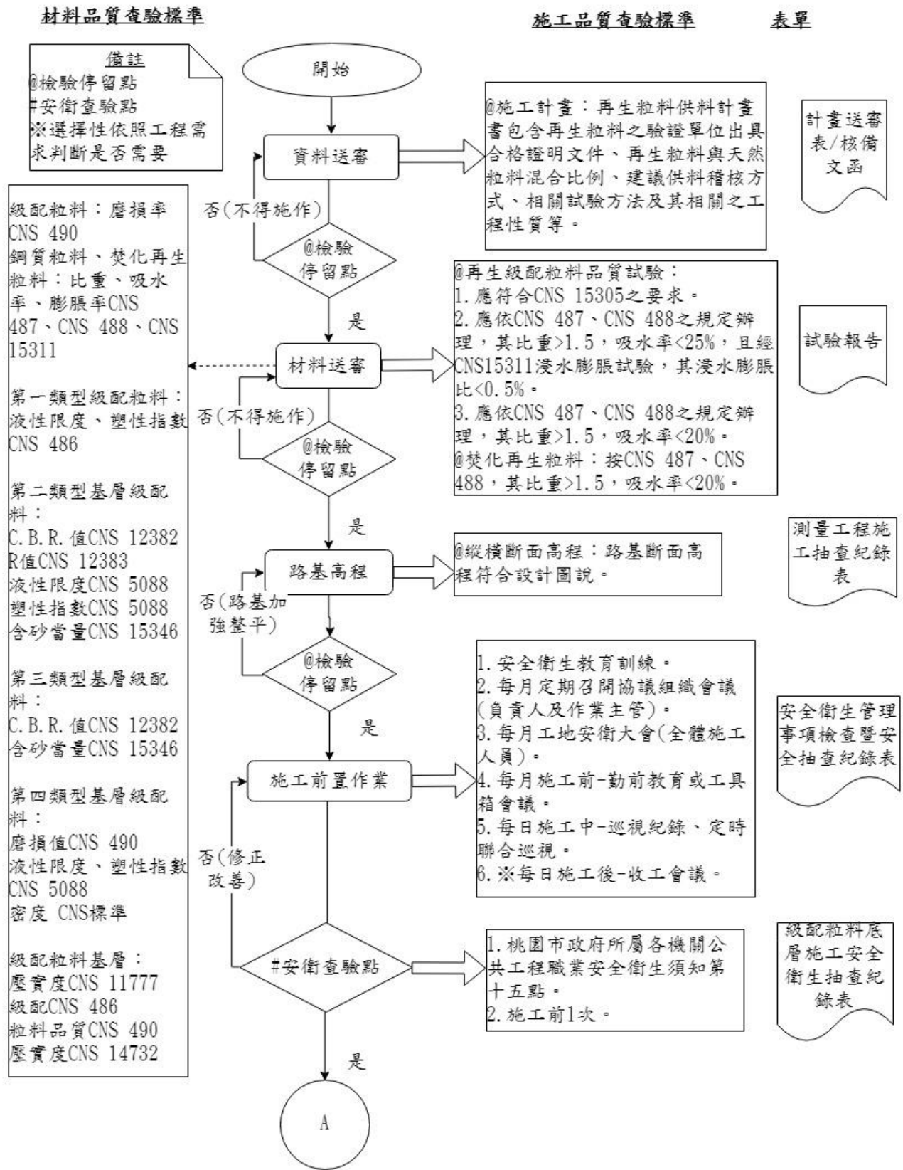
圖 027220-F-1 級配粒料基層施工抽查流程圖 1/2
