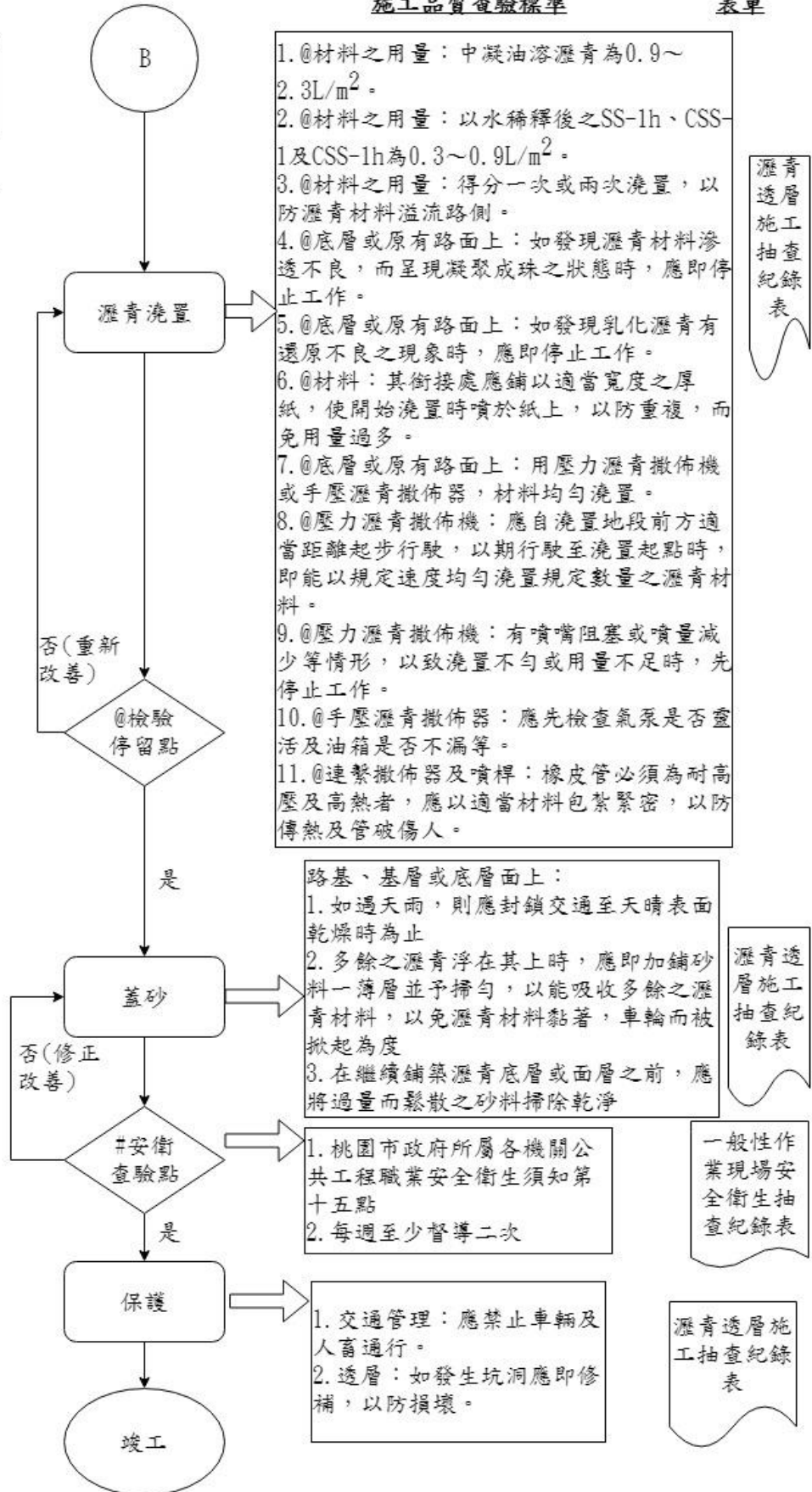
圖 027450-F-1 瀝青透層施工抽查流程圖 3/3
