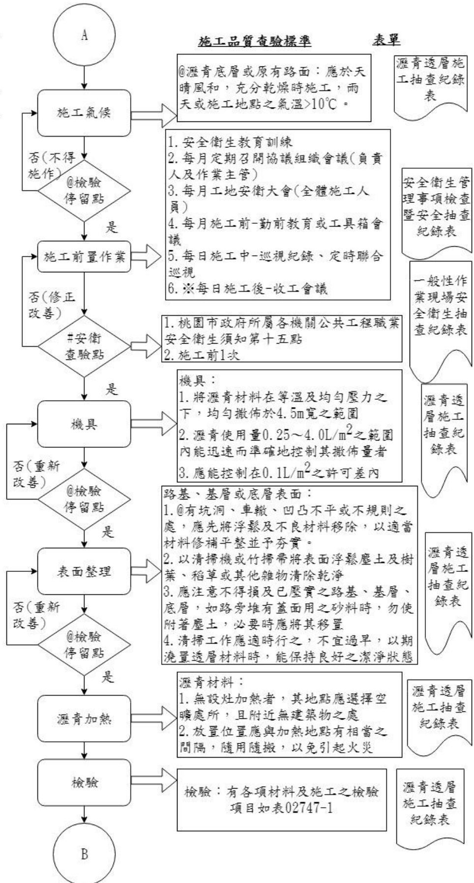
圖 027450-F-1 瀝青透層施工抽查流程圖 2/3
