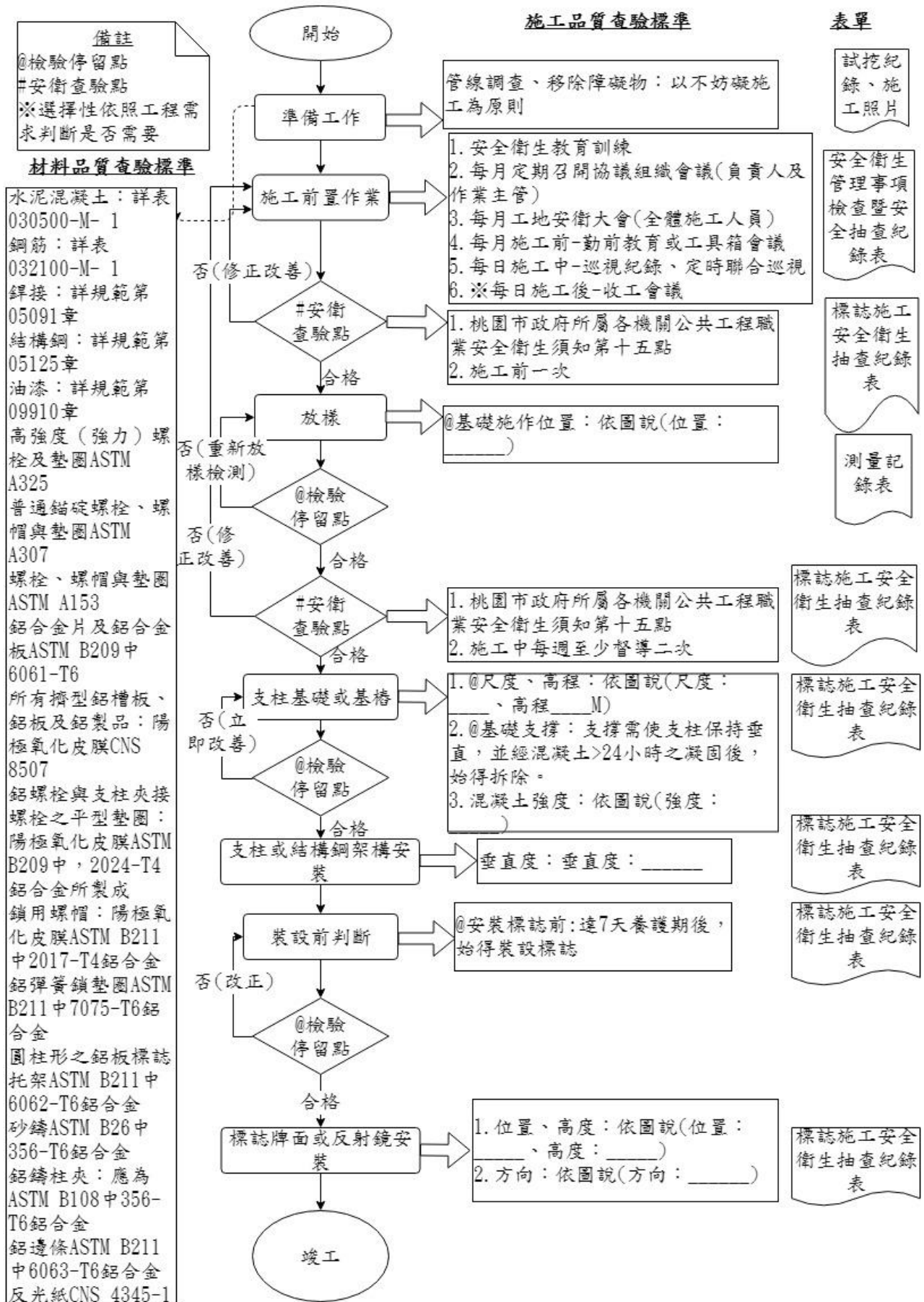
圖 028910-F-1 標誌工程施工抽查流程圖 1/1
