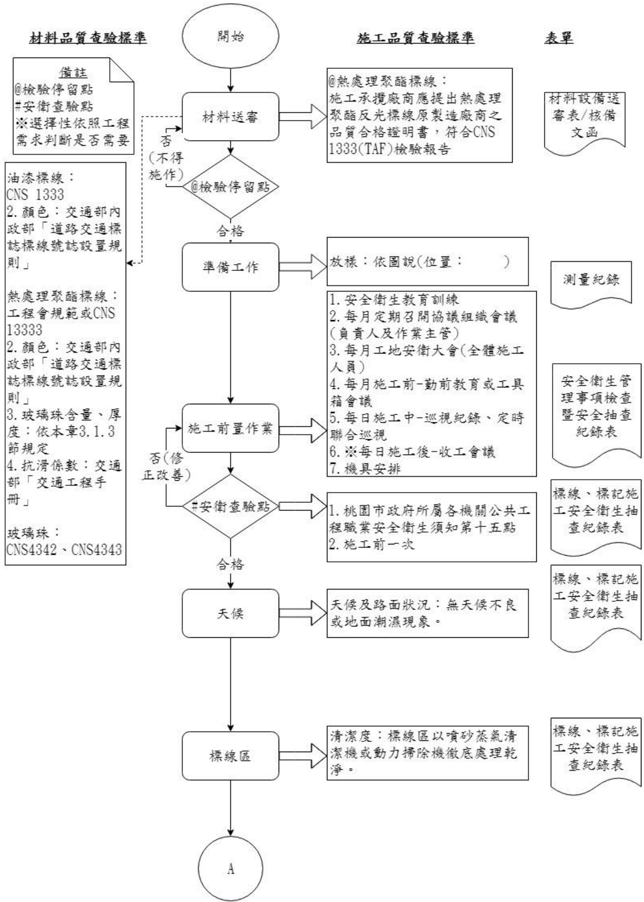
圖 028980-F-1 標線、標記工程施工抽查流程圖 1/2
