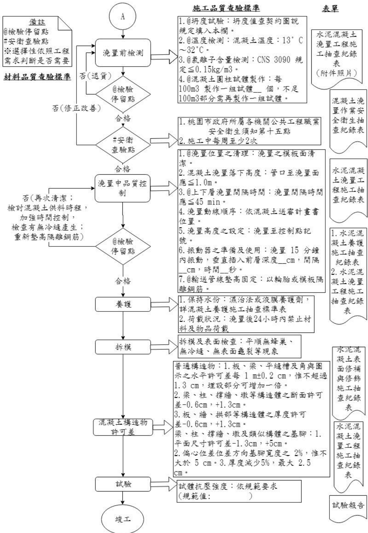
圖 030500-F-1 水泥混凝土工程施工流程圖 2/2
