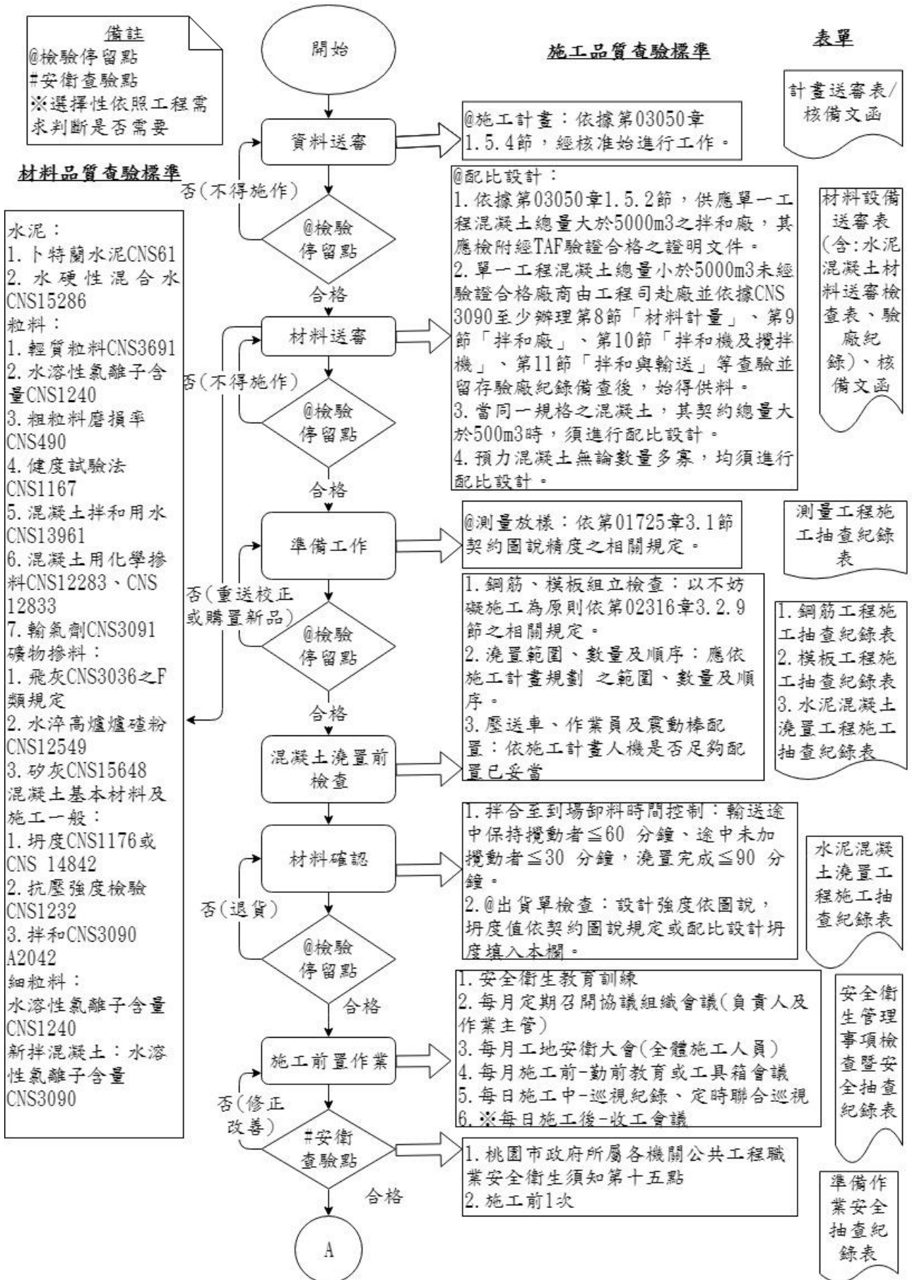
圖 030500-F-1 水泥混凝土工程施工流程圖 1/2
