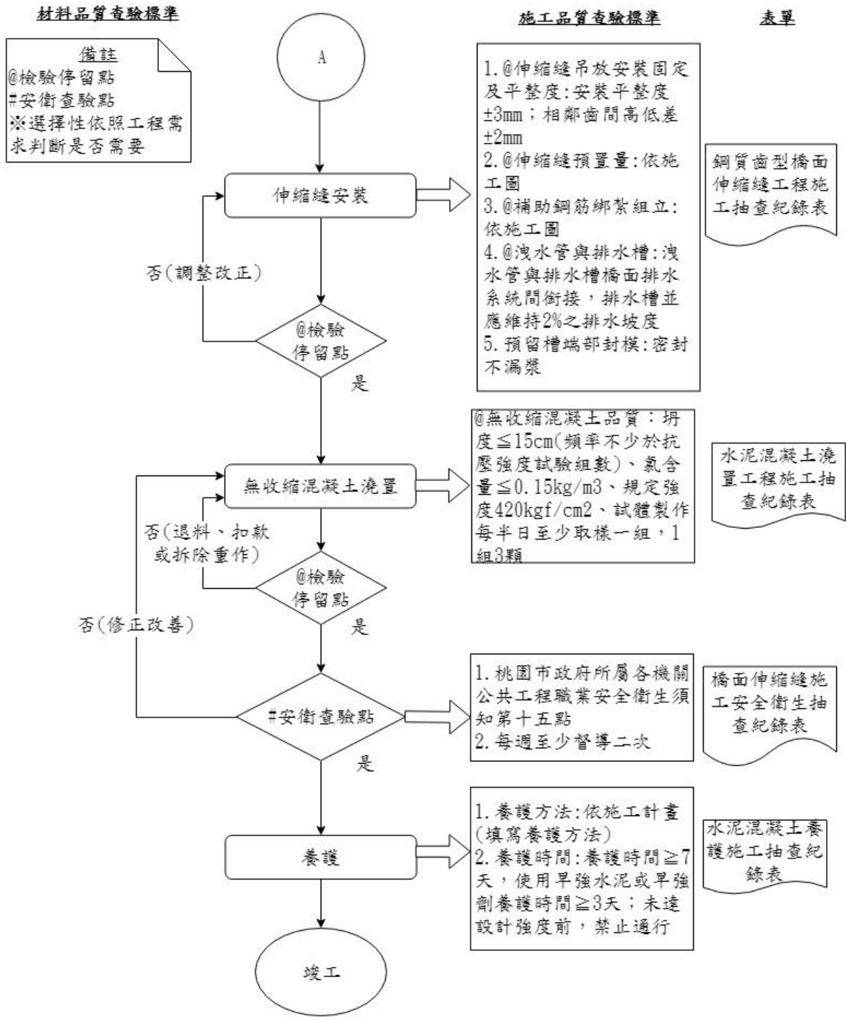
圖 058310-F-1 鋼質齒型橋面伸縮縫工程施工抽查流程圖 2/2
