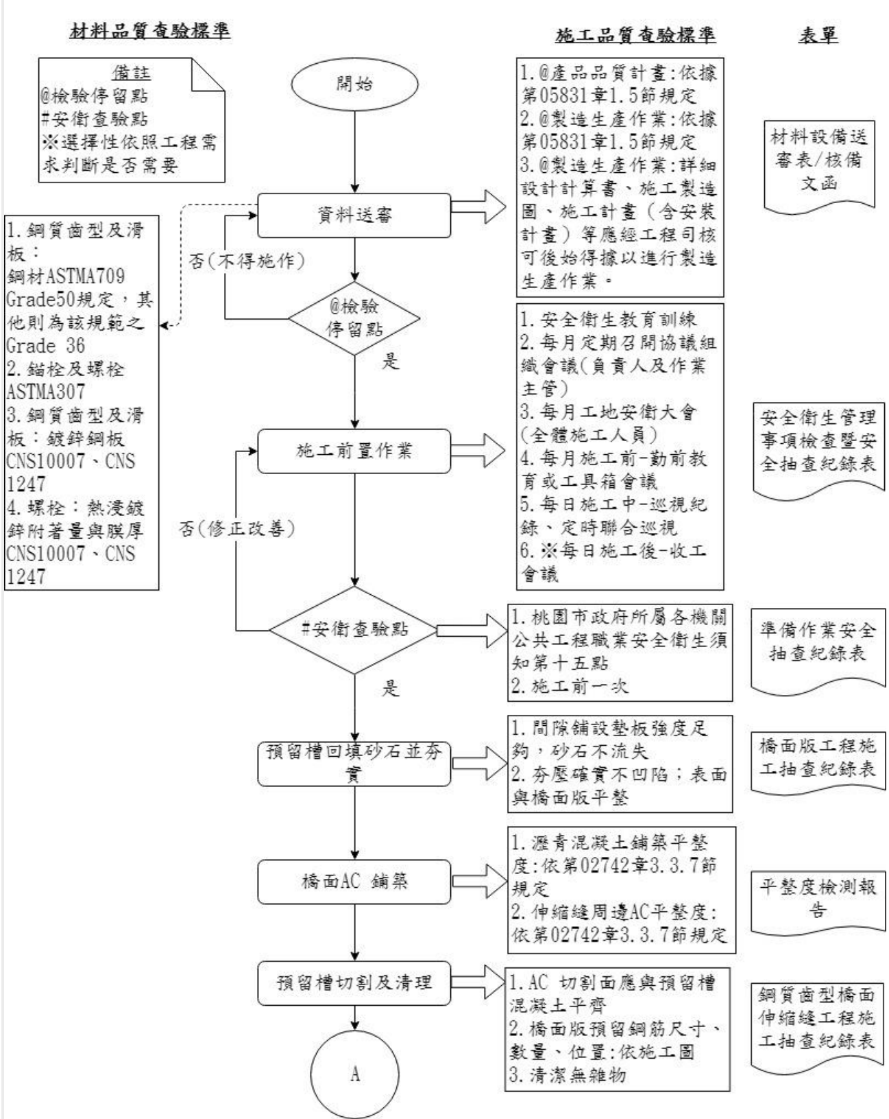
圖 058310-F-1 鋼質齒型橋面伸縮縫工程施工抽查流程圖 1/2
