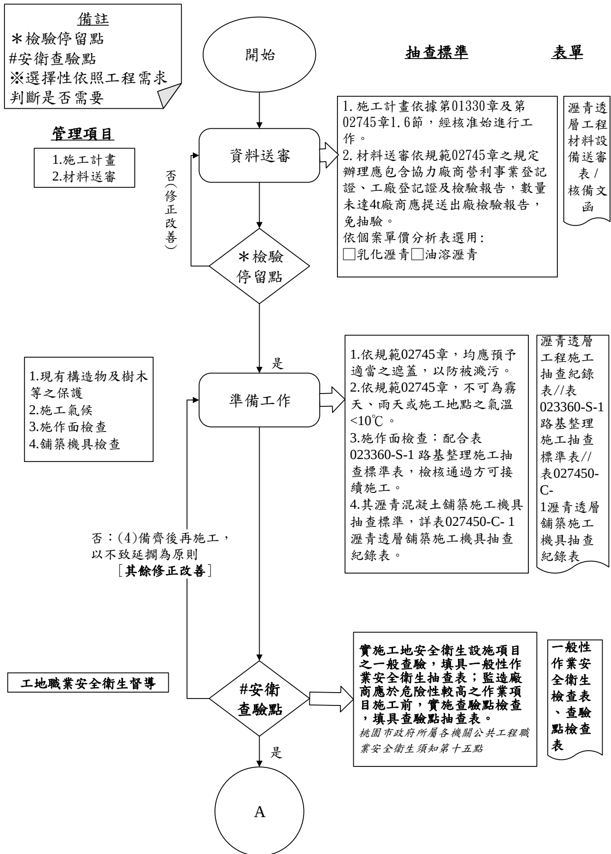
圖 027450-F-1 瀝青透層施工抽查流程圖 1/3
