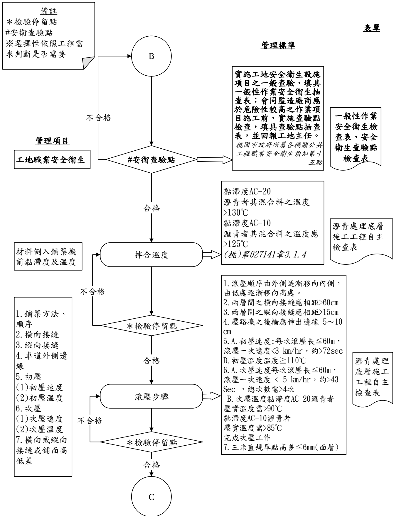
圖 027141-QCF-1 瀝青處理底層施工檢驗流程圖 3/4
