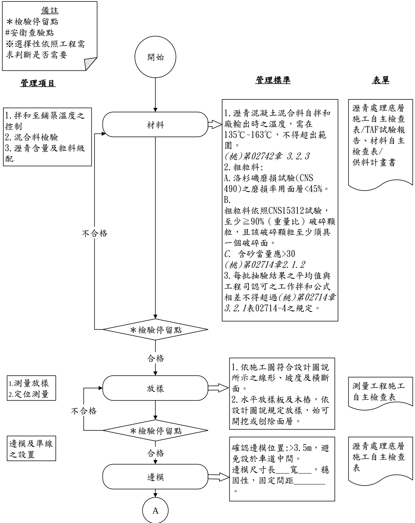
圖 027141-QCF-1 瀝青處理底層施工檢驗流程圖 1/4
