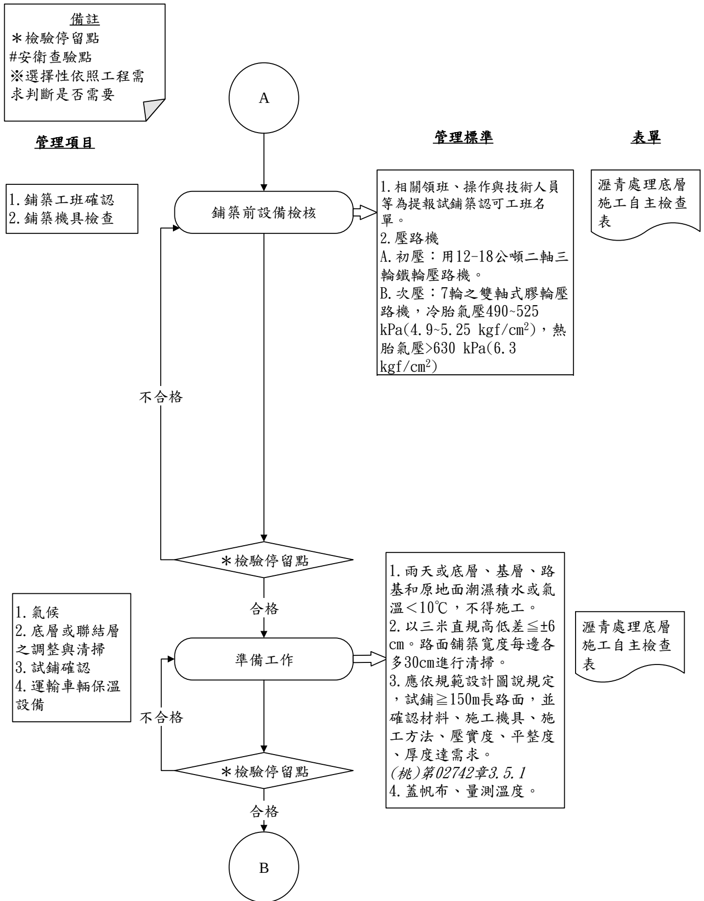
圖 027141-QCF-1 瀝青處理底層施工檢驗流程圖 2/4
