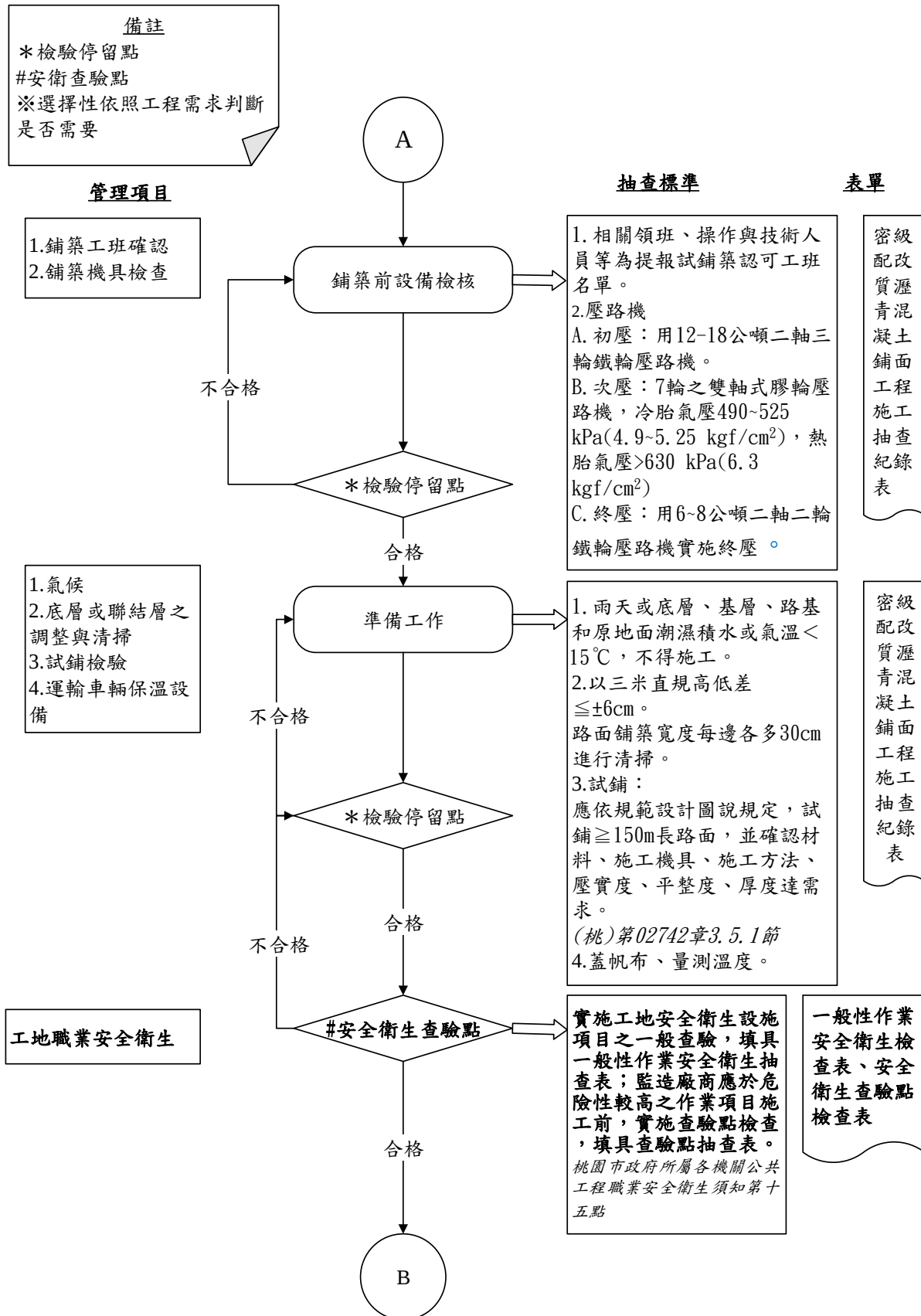
圖 027962-F-1 密級配改質瀝青混凝土鋪面工程施工抽查流程圖 2/5
