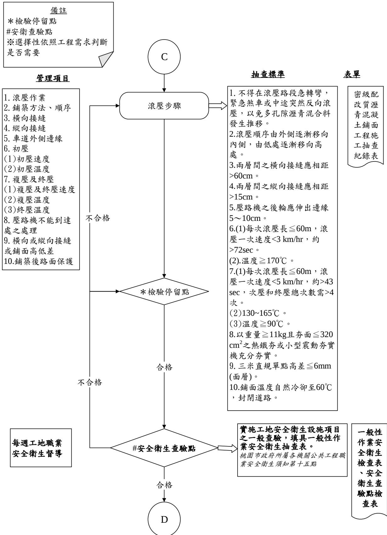
圖 027962-F-1 密級配改質瀝青混凝土鋪面工程施工抽查流程圖 4/5
