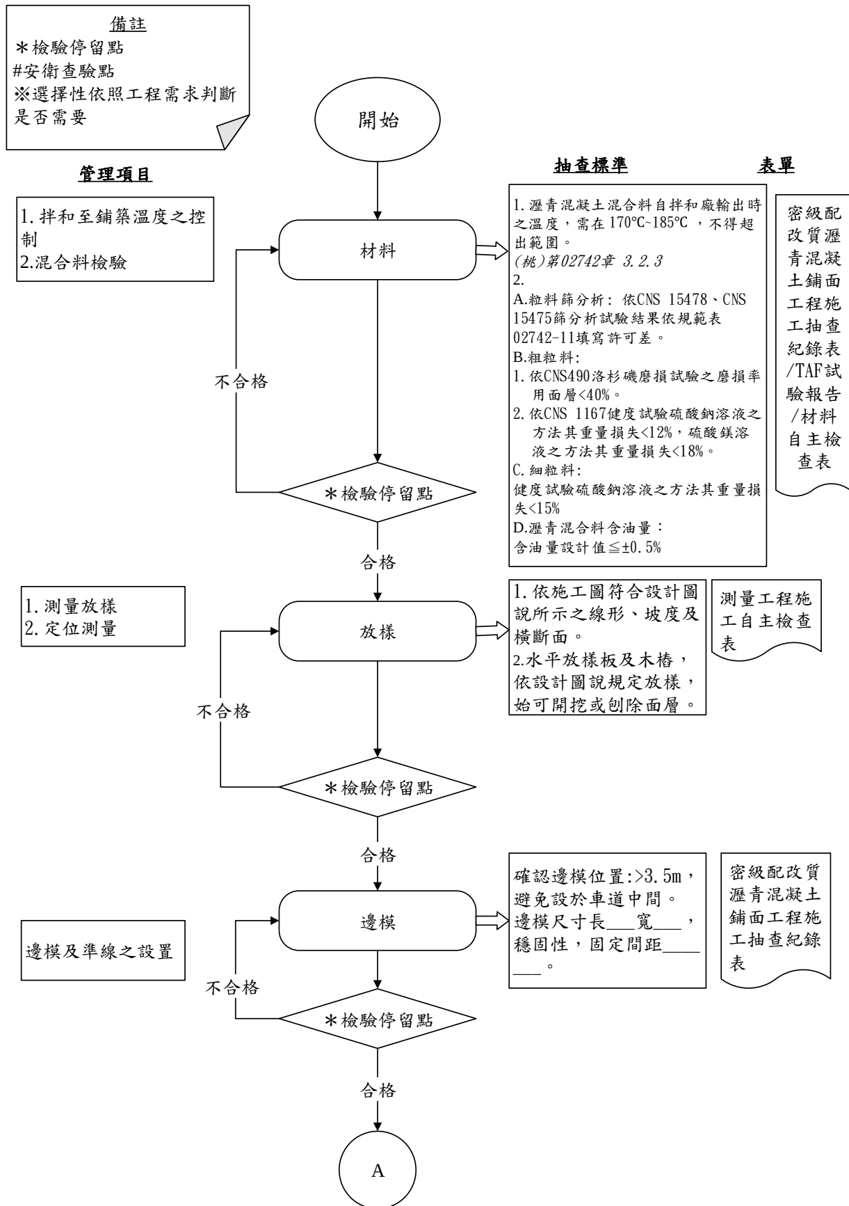
圖 027962-F-1 密級配改質瀝青混凝土鋪面工程施工抽查流程圖 1/5
