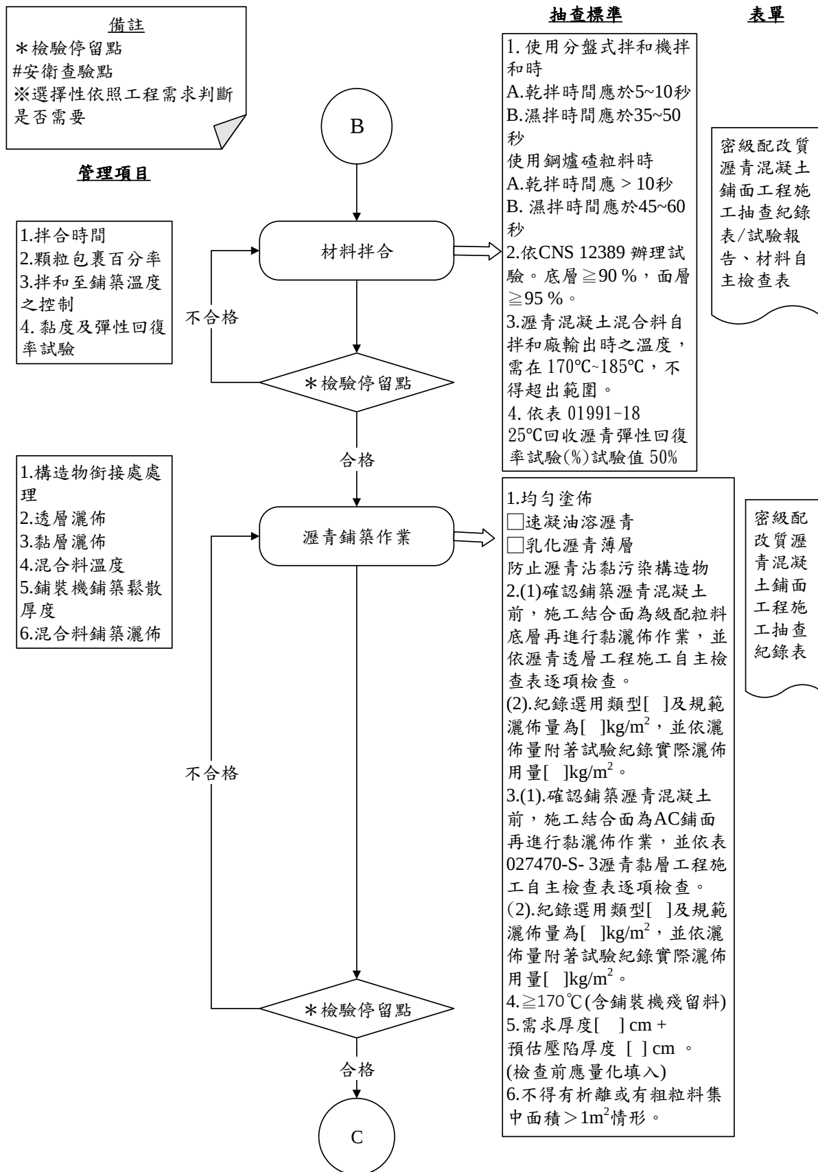
圖 027962-F-1 密級配改質瀝青混凝土鋪面工程施工抽查流程圖 3/5
