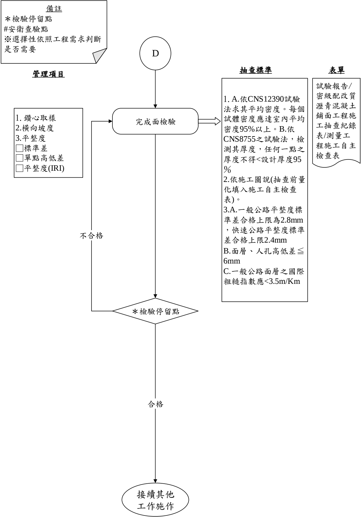
圖 027962-F-1 密級配改質瀝青混凝土鋪面工程施工抽查流程圖 5/5
