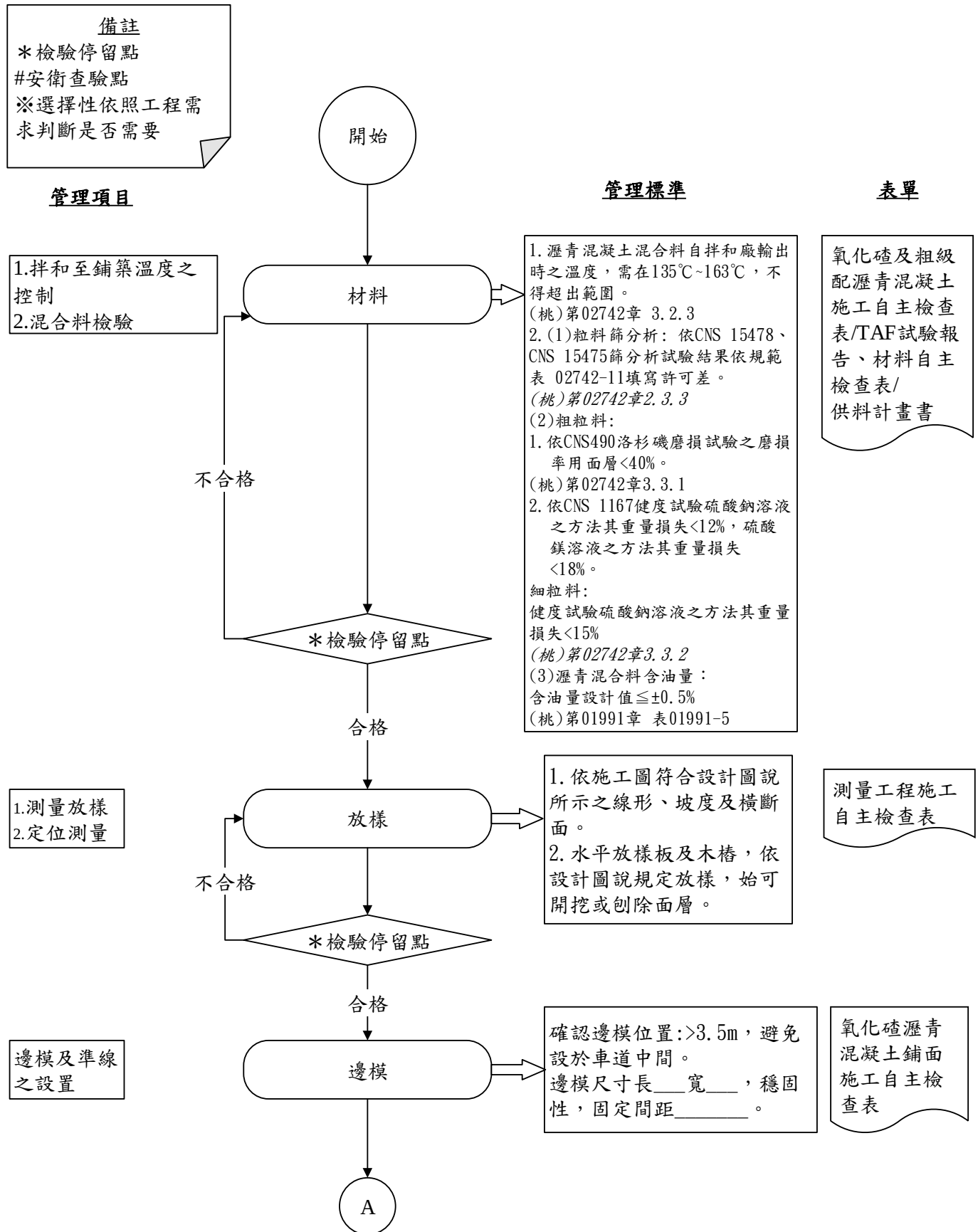
圖 027021-QCF-1 氧化碇瀝青混凝土鋪面施工檢驗流程圖 1/5
