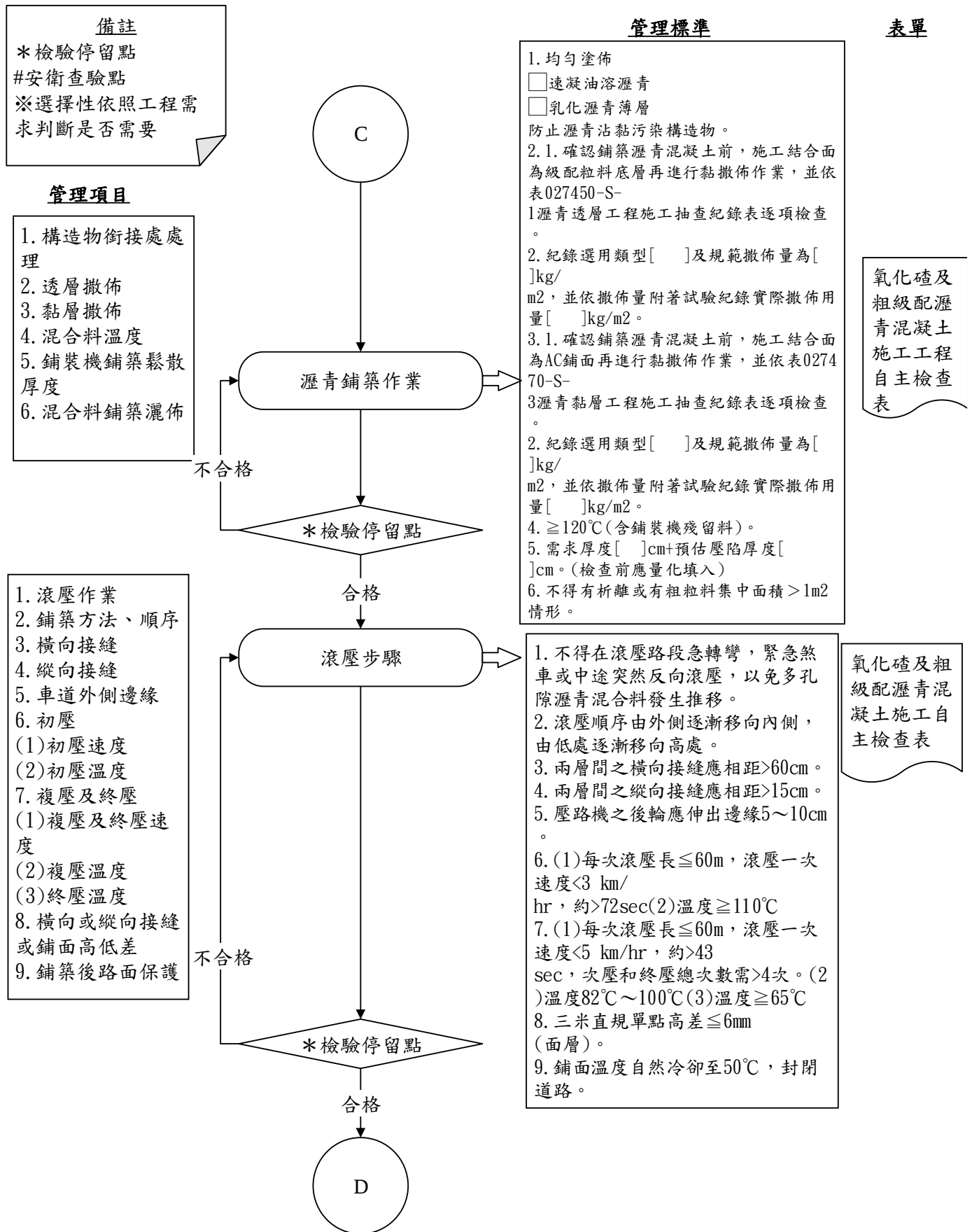
圖 027021-QCF-1 氧化碇瀝青混凝土鋪面施工檢驗流程圖 4/5
