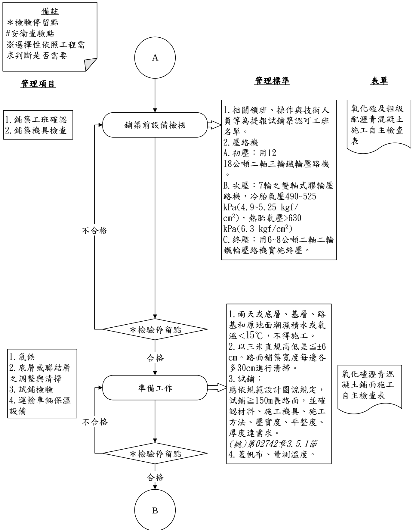
圖 027021-QCF-1 氧化碇瀝青混凝土鋪面施工檢驗流程圖 2/5
