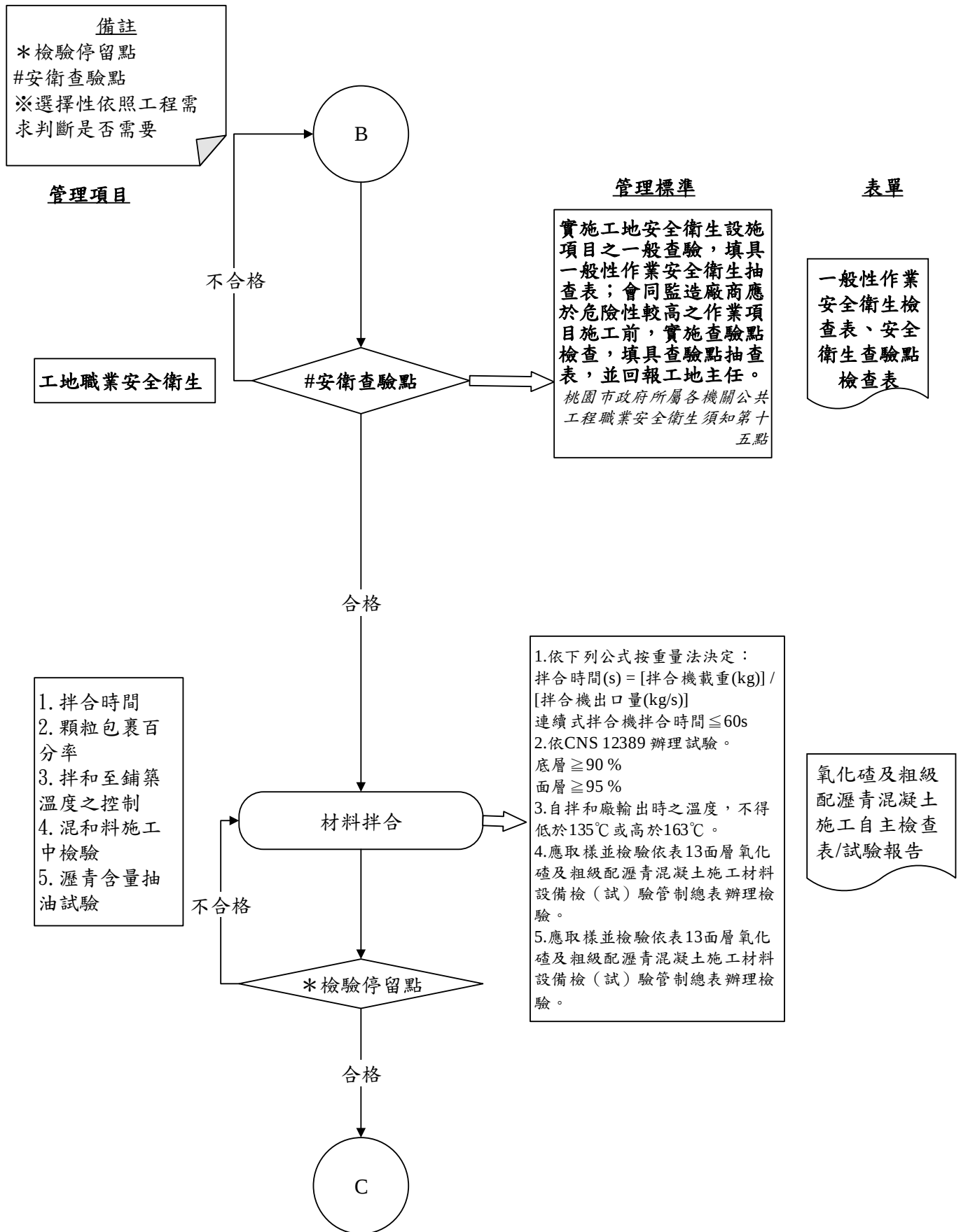
圖 027021-QCF-1 氧化矽瀝青混凝土鋪面施工檢驗流程圖 3/5
