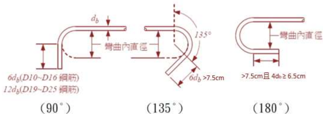
圖 03210- 2 肋筋及箍筋標準彎鉤
