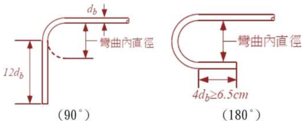
圖 03210- 1 主鋼筋之標準彎鉤
