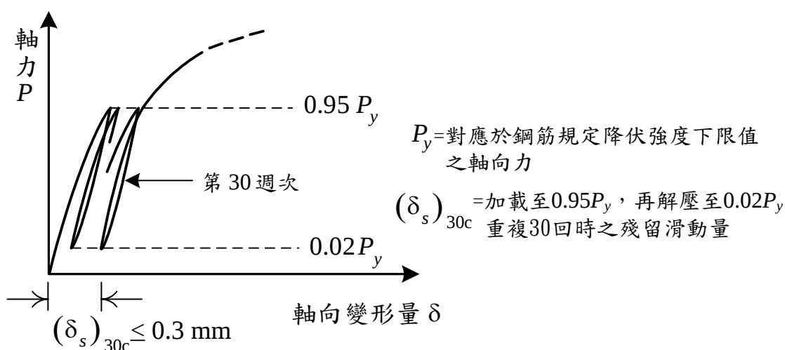
圖三 續接試體重複負載及滑動試驗加載程式示意圖
