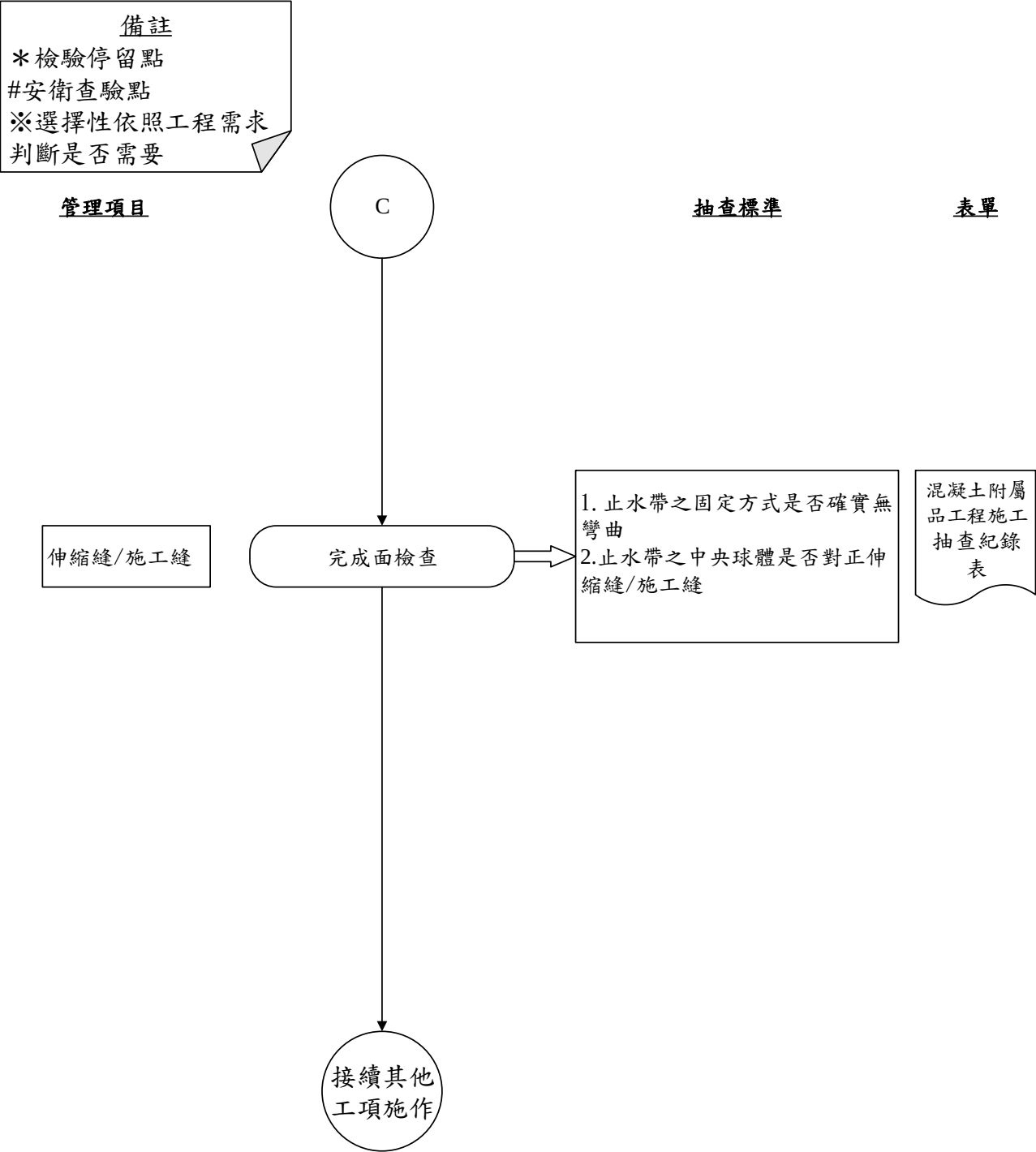
圖 031502-F- 4 混凝土附屬品工程施工抽查流程圖 4/4
