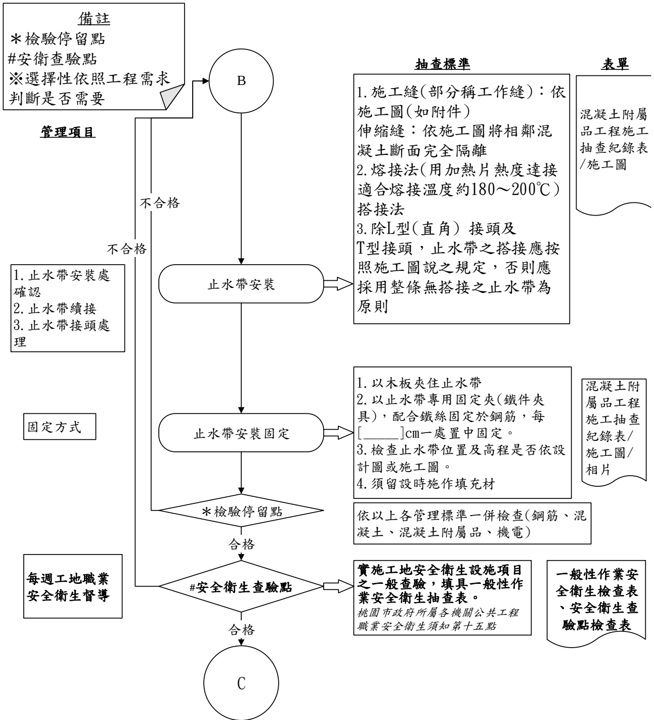
圖 031502-F- 3 混凝土附屬品工程施工抽查流程圖 3/4
