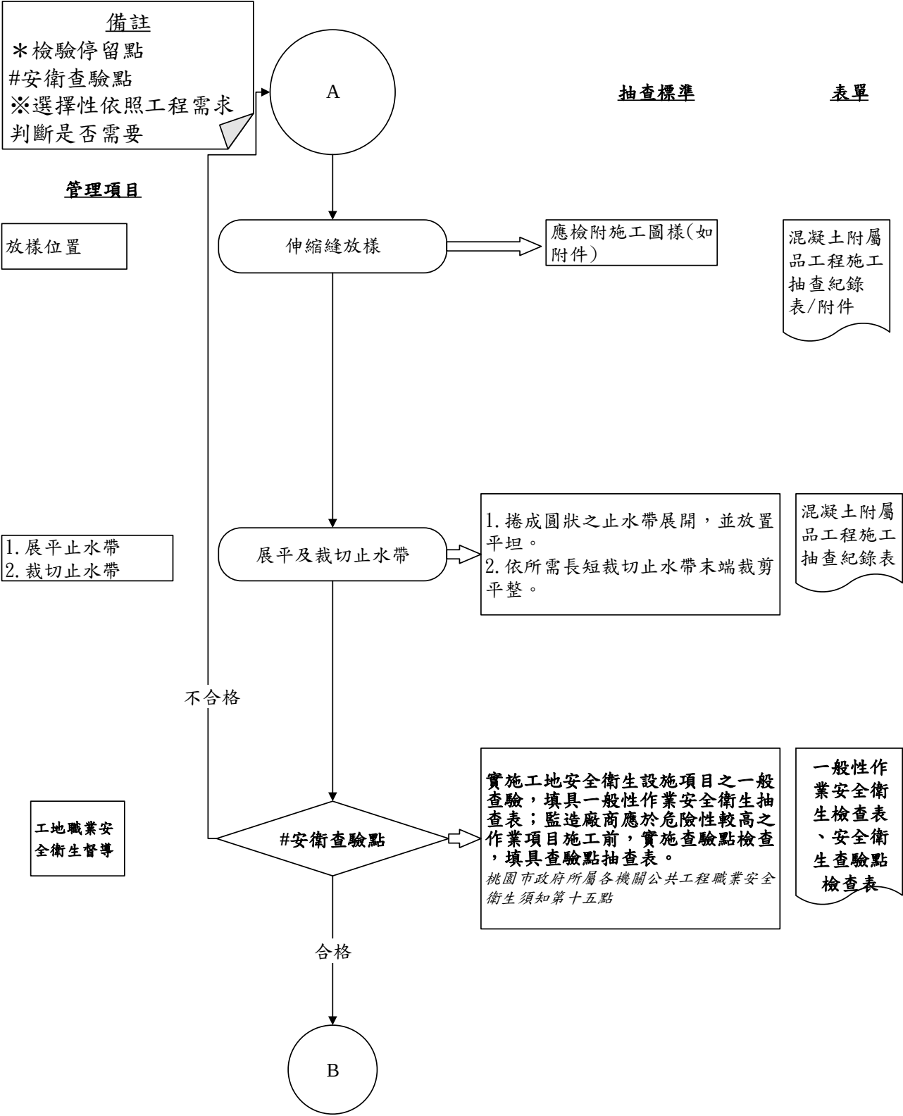
圖 031502-F- 2 混凝土附屬品工程施工抽查流程圖 2/4
