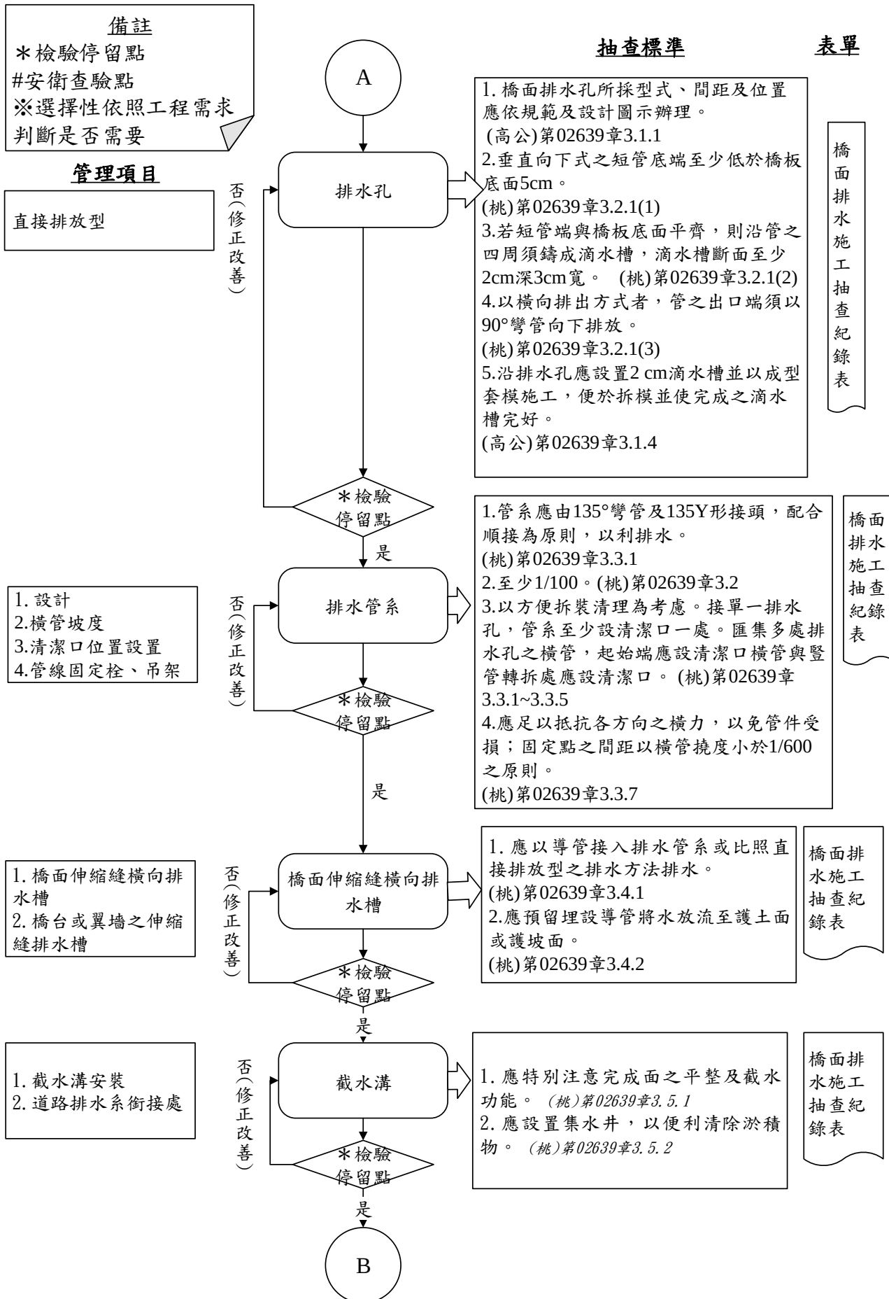
圖 026390-F-2 橋面排水施工抽查流程圖 2/4
