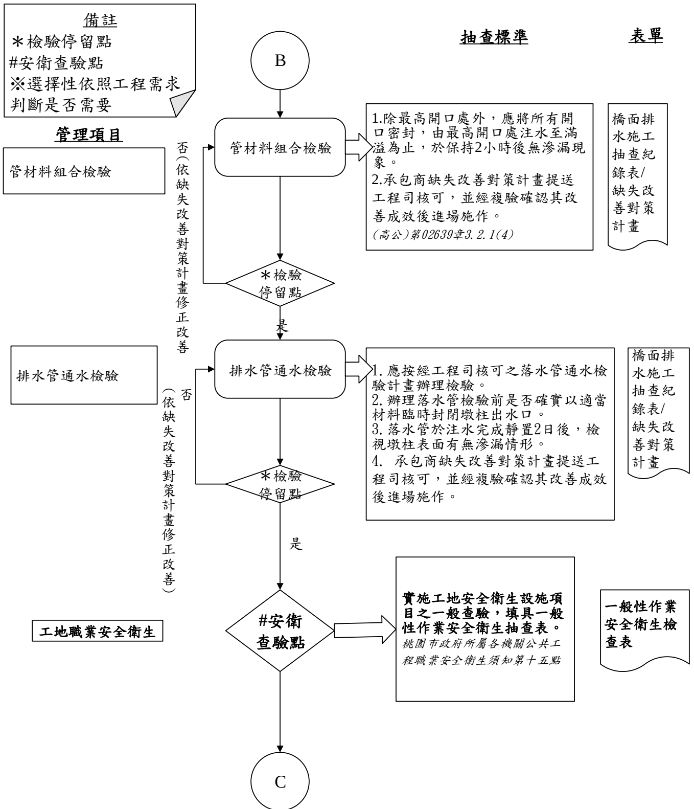
圖 026390-F- 3 橋面排水施工抽查流程圖 3/4
