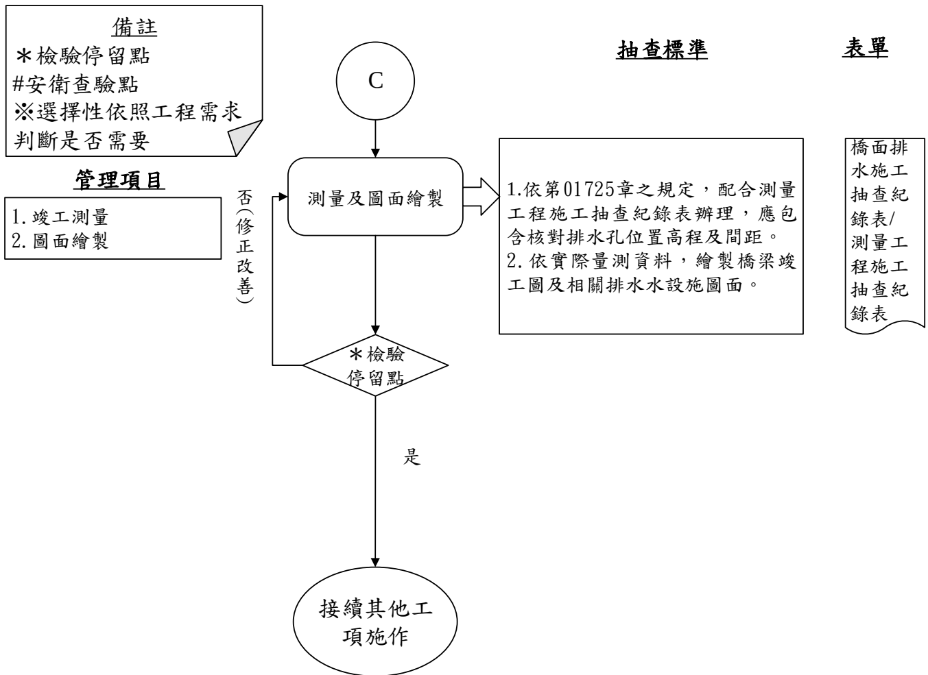
圖 026390-F- 4 橋面排水施工抽查流程圖 4/4
