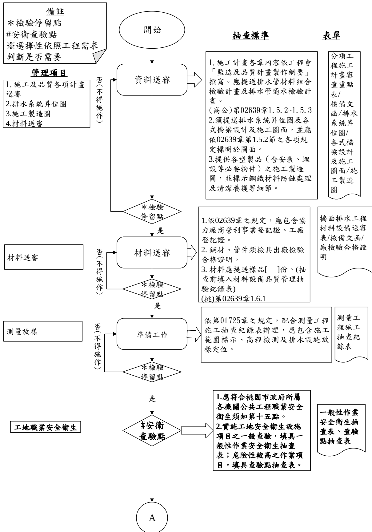
圖 026390-F-1 橋面排水施工抽查流程圖 1/4
