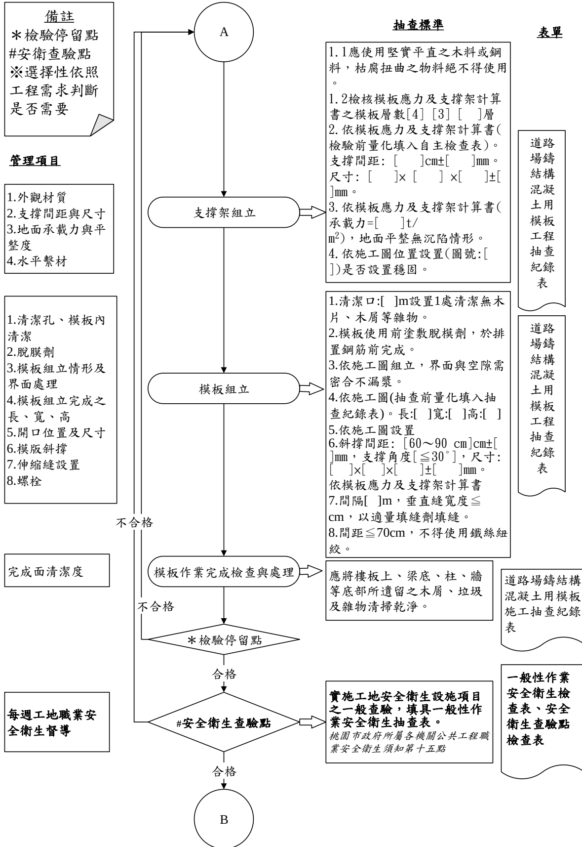
圖 031102-F- 2 道路場鑄結構混凝土用模板工程施工抽查流程圖 2/3
