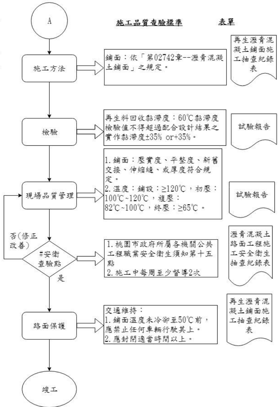
圖 029660-F-1 再生瀝青混凝土鋪面施工抽查流程圖 2/2
