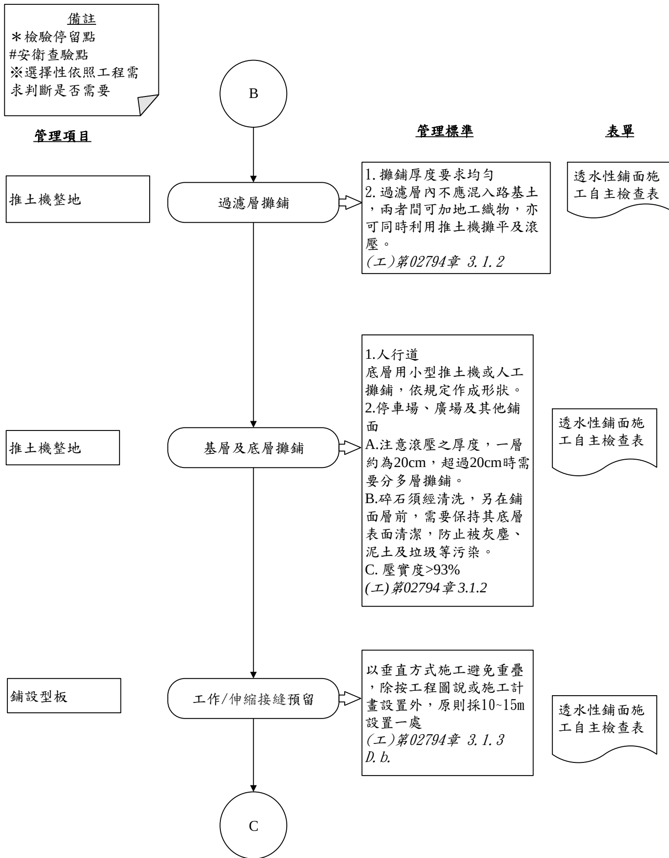
圖 027941-QCF-1 透水性鋪面工程施工檢驗流程圖 3/6
