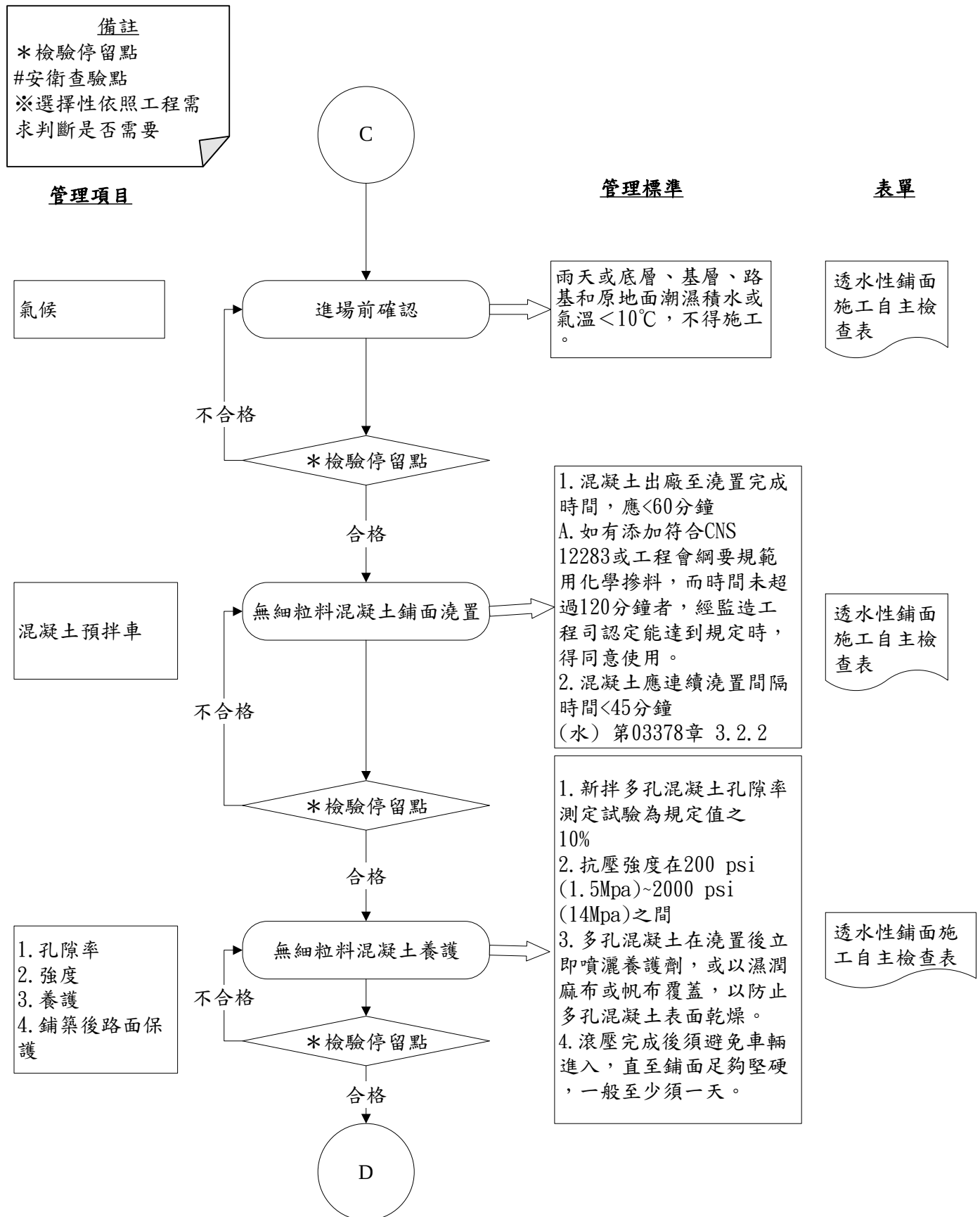
圖 027941-QCF-1 透水性鋪面工程施工檢驗流程圖 4/6
