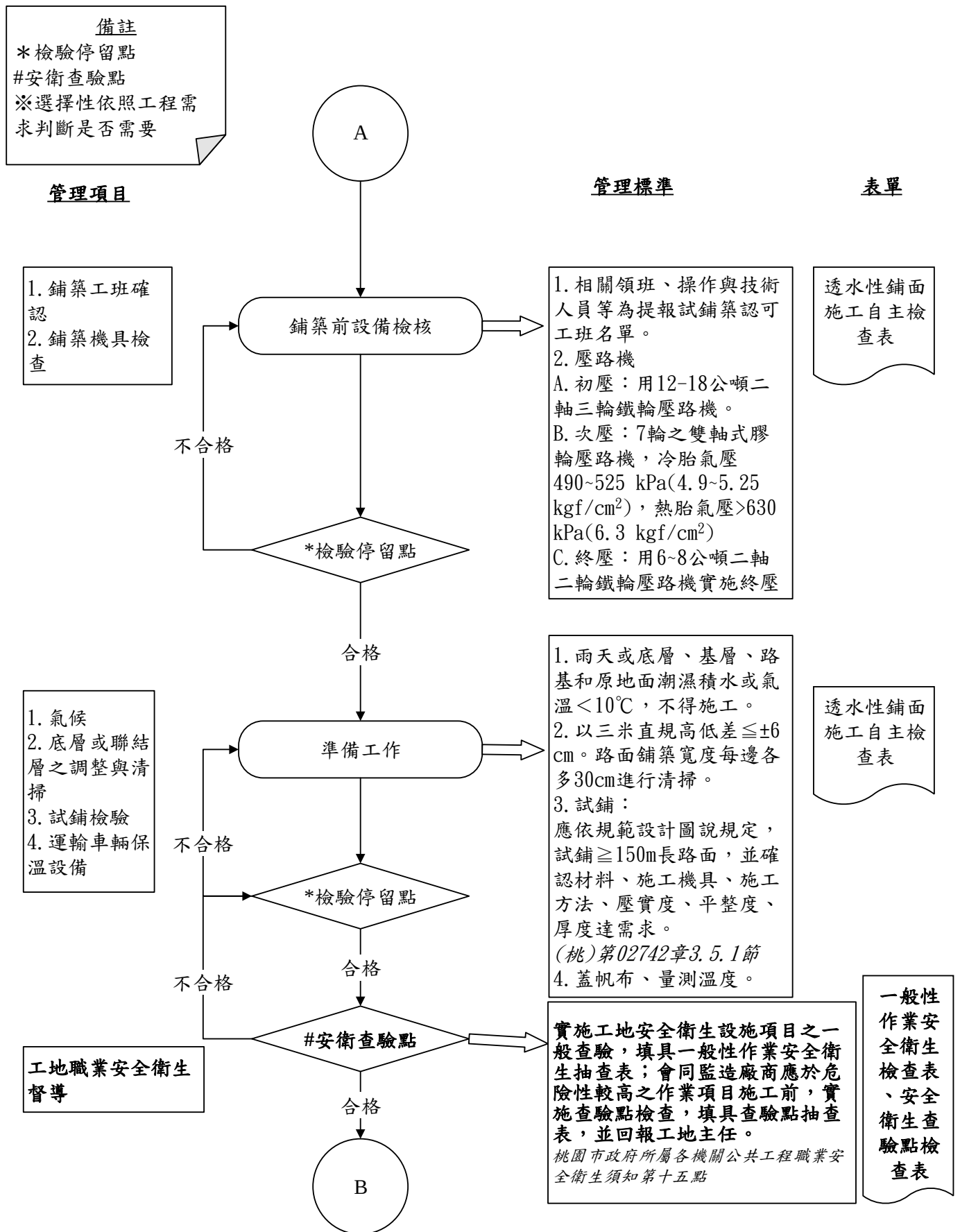
圖 027941-QCF-1 透水性鋪面工程施工檢驗流程圖 2/6
