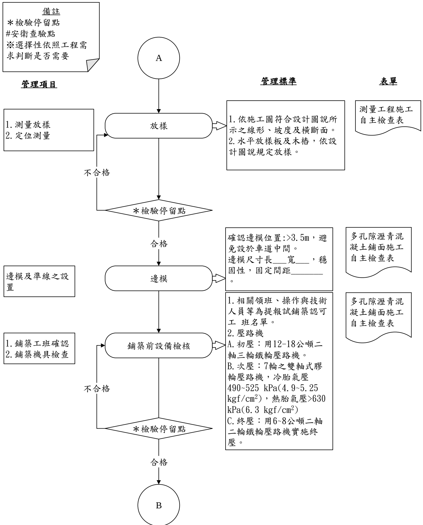
圖 027981-QCF-1 多孔隙瀝青混凝土鋪面工程施工檢驗流程圖 2/6
