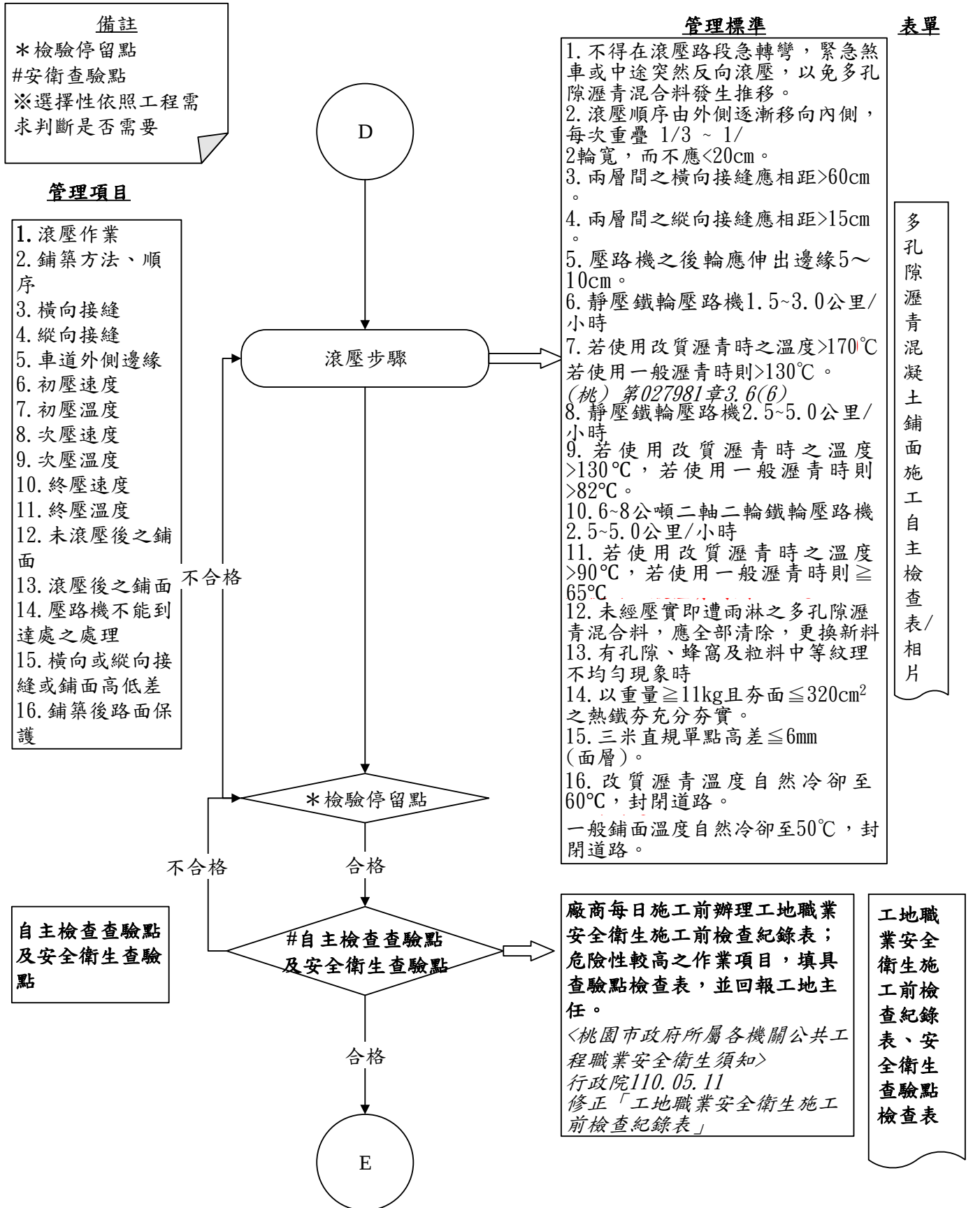
圖 027981-QCF-1 多孔隙瀝青混凝土鋪面工程施工檢驗流程圖 5/6
