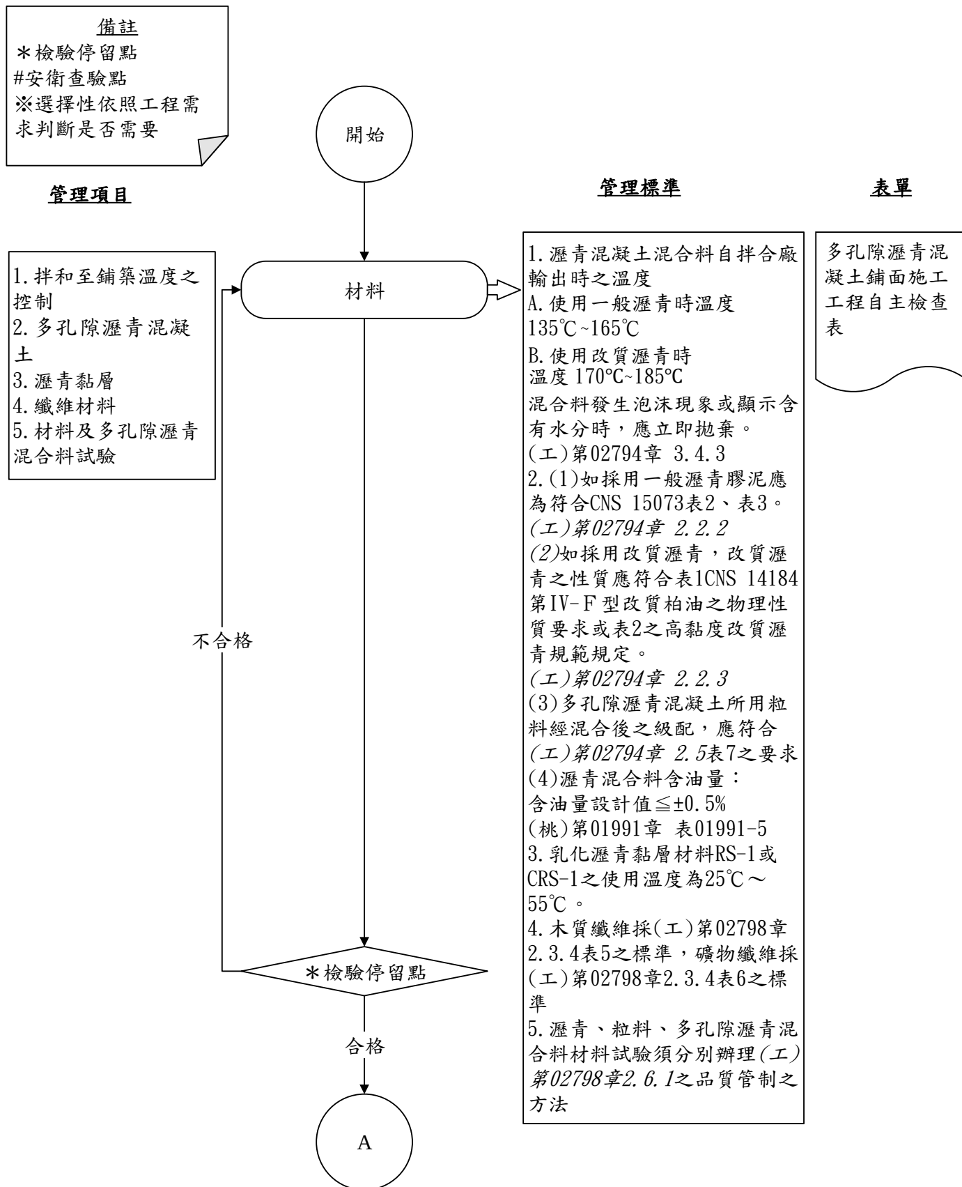
圖 027981-QCF-1 多孔隙瀝青混凝土鋪面工程施工檢驗流程圖 1/6
