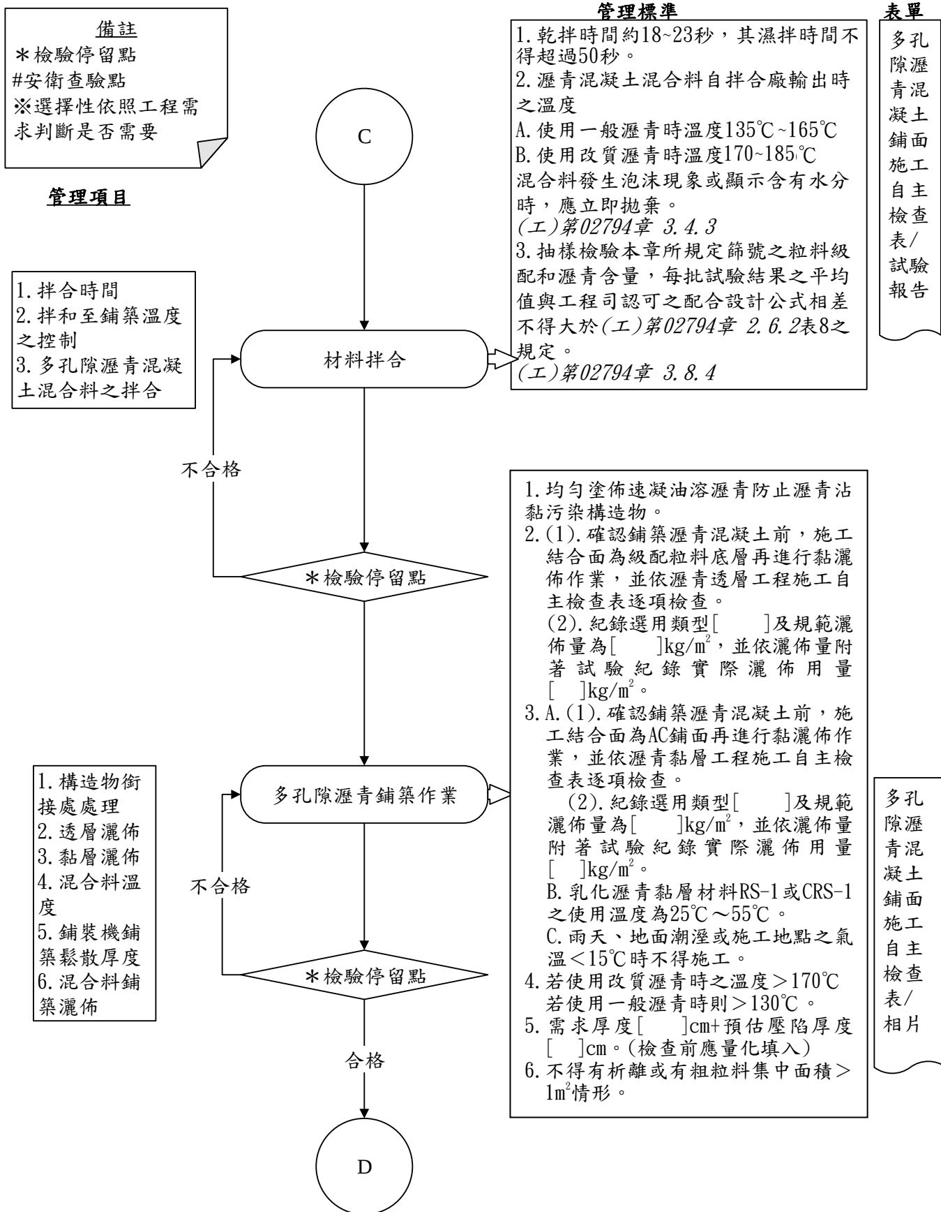
圖 027981-QCF-1 多孔隙瀝青混凝土鋪面工程施工檢驗流程圖 4/6
