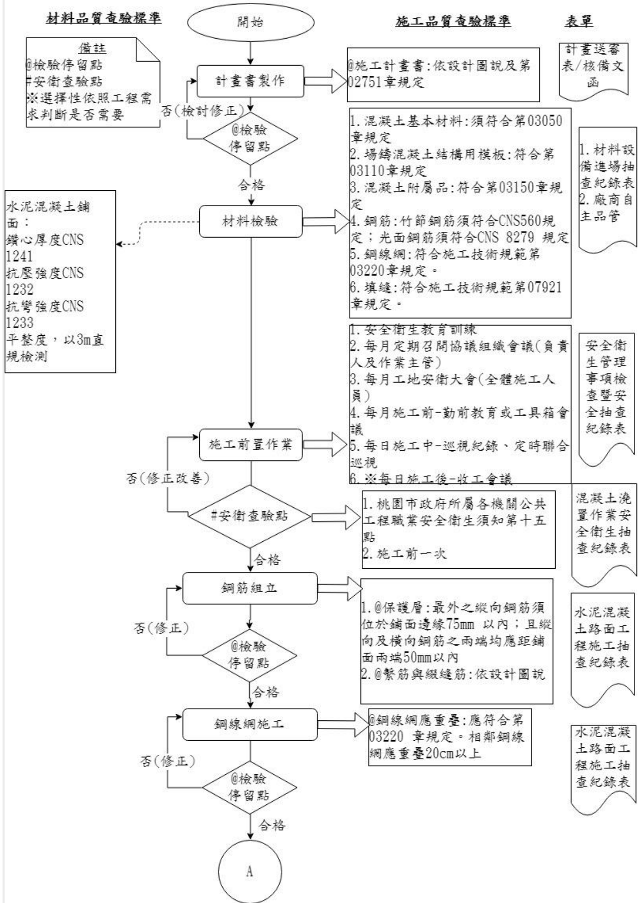
圖 027510-F-1 水泥混凝土路面工程施工抽查流程圖 1/3
