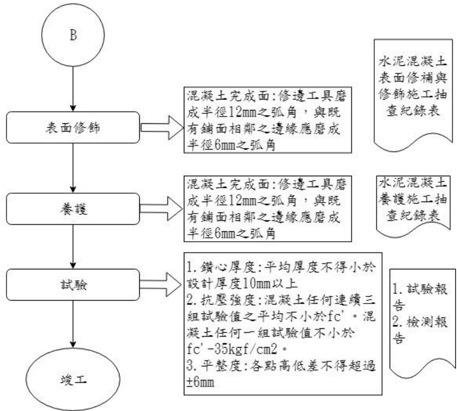
圖 027510-F-1 水泥混凝土路面工程施工抽查流程圖 3/3
