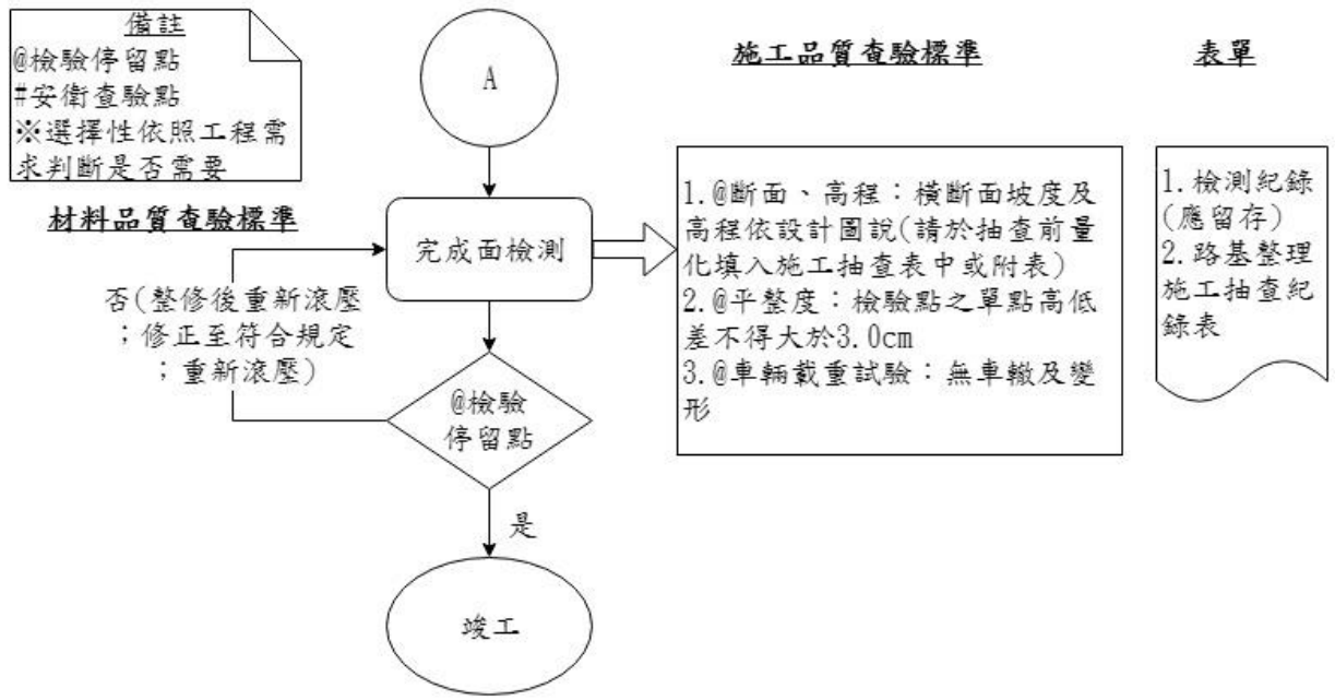
圖 023360-F-1 路基整理施工抽查流程圖 2/2
