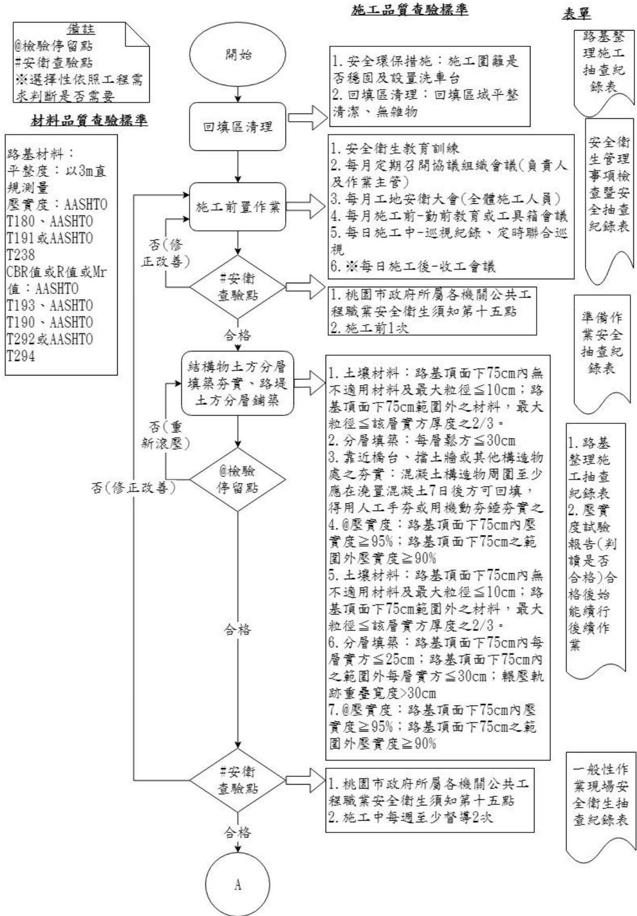
圖 023360-F-1 路基整理施工抽查流程圖 1/2
