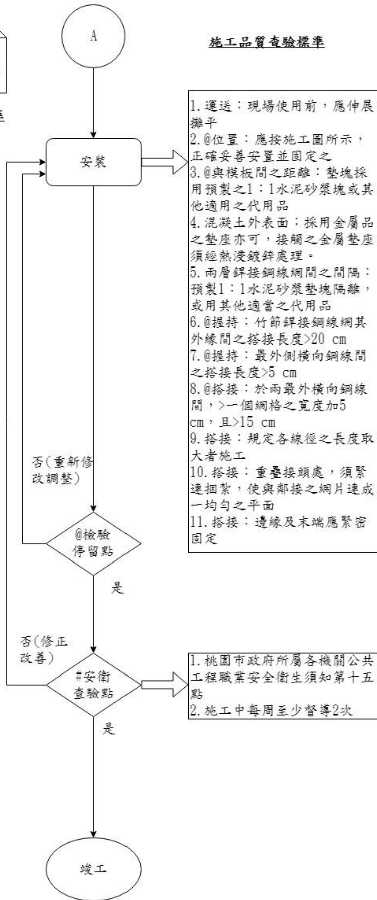
圖 032200-F-1 銲接鋼線網施工抽查流程圖 2/2
