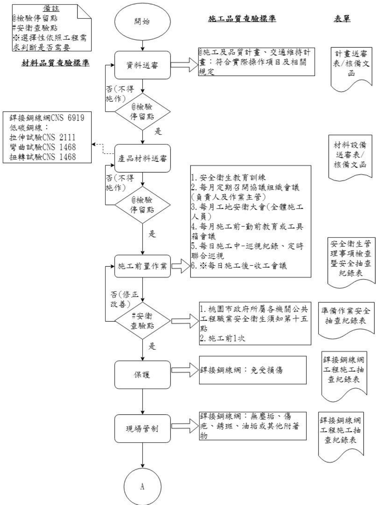
圖 032200-F-1 銲接鋼線網施工抽查流程圖 1/2
