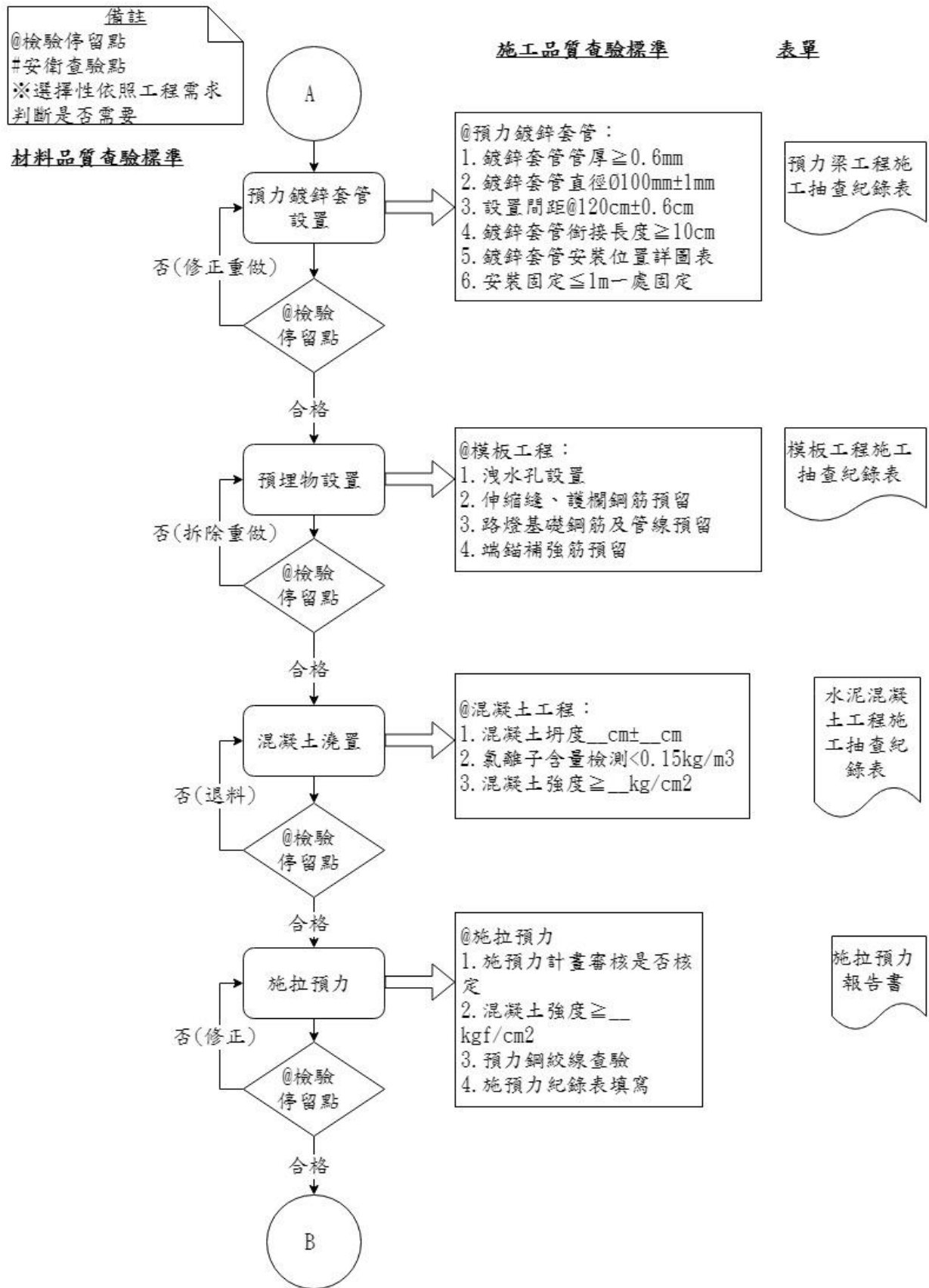
圖 034320-F-1 預力梁工程施工抽查流程圖 2/3
