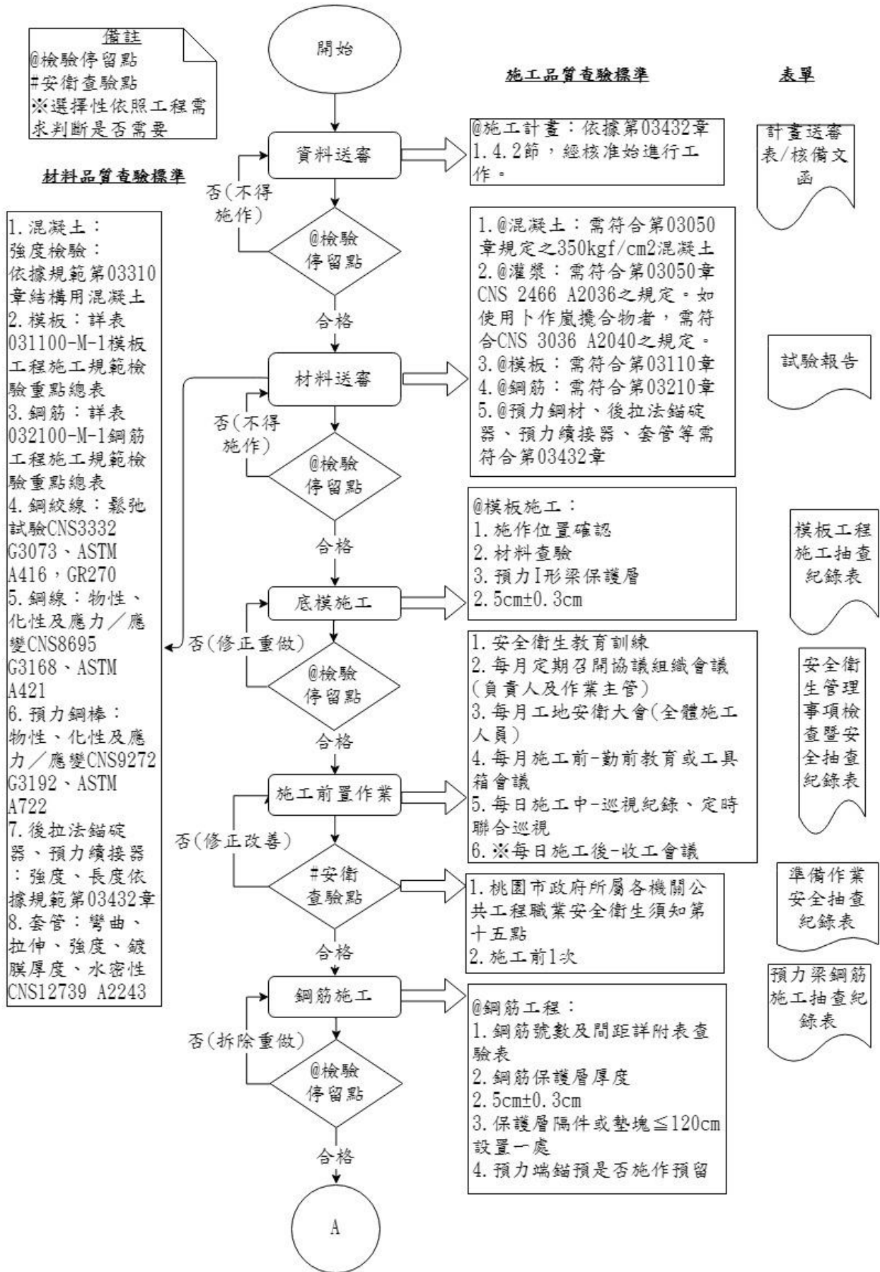
圖 034320-F-1 預力梁工程施工抽查流程圖 1/3
