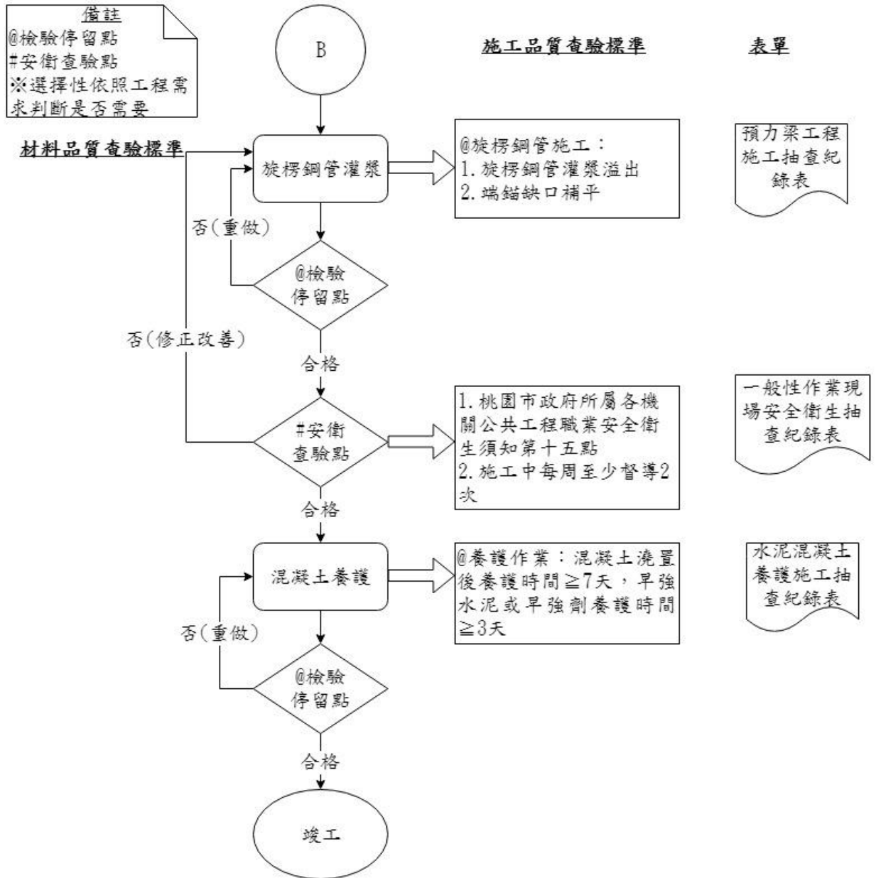
圖 034320-F-1 預力梁工程施工抽查流程圖 3/3
