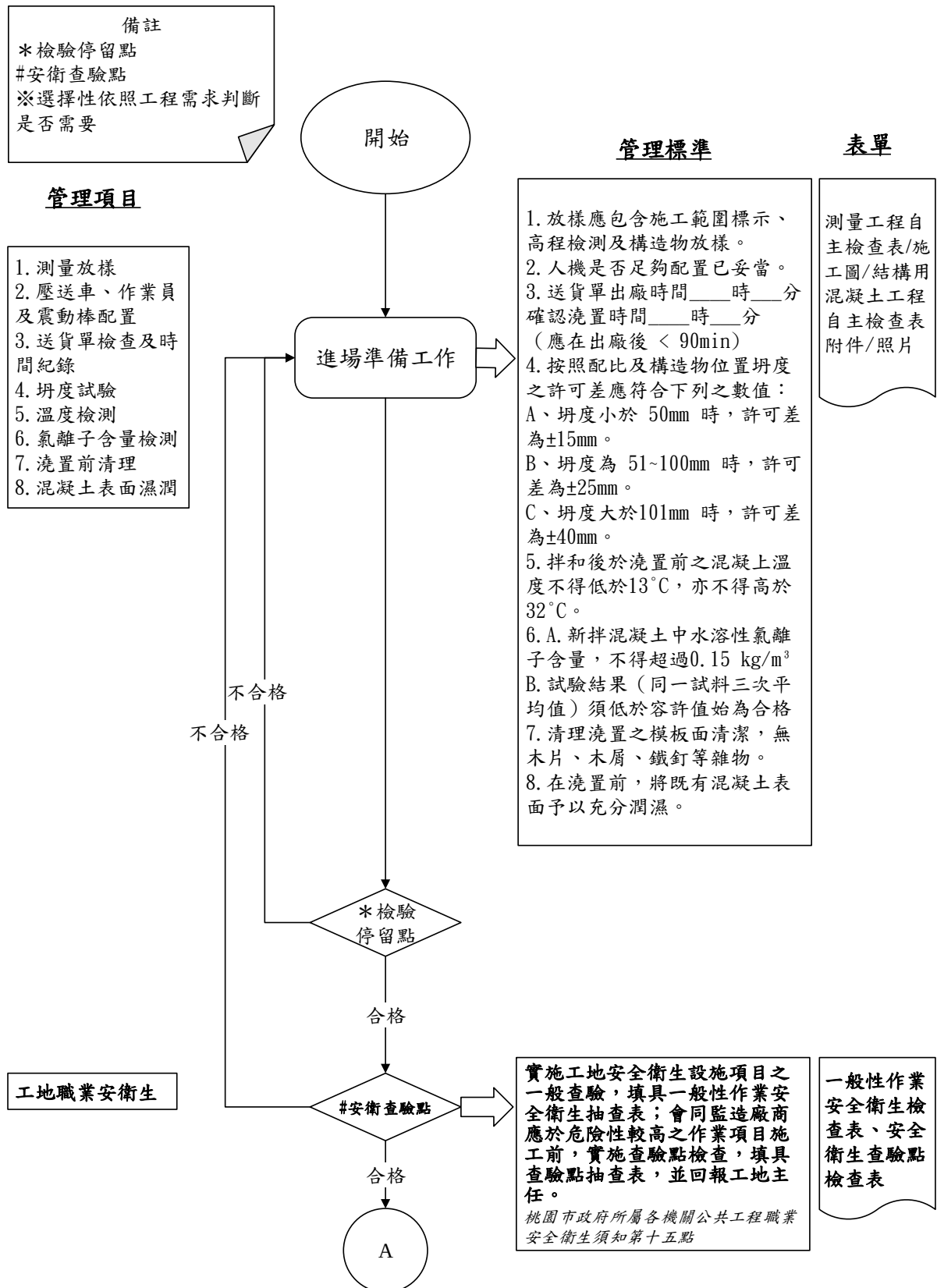
圖 033101-QCF- 1 結構用混凝土工程施工檢驗流程圖 1/4
