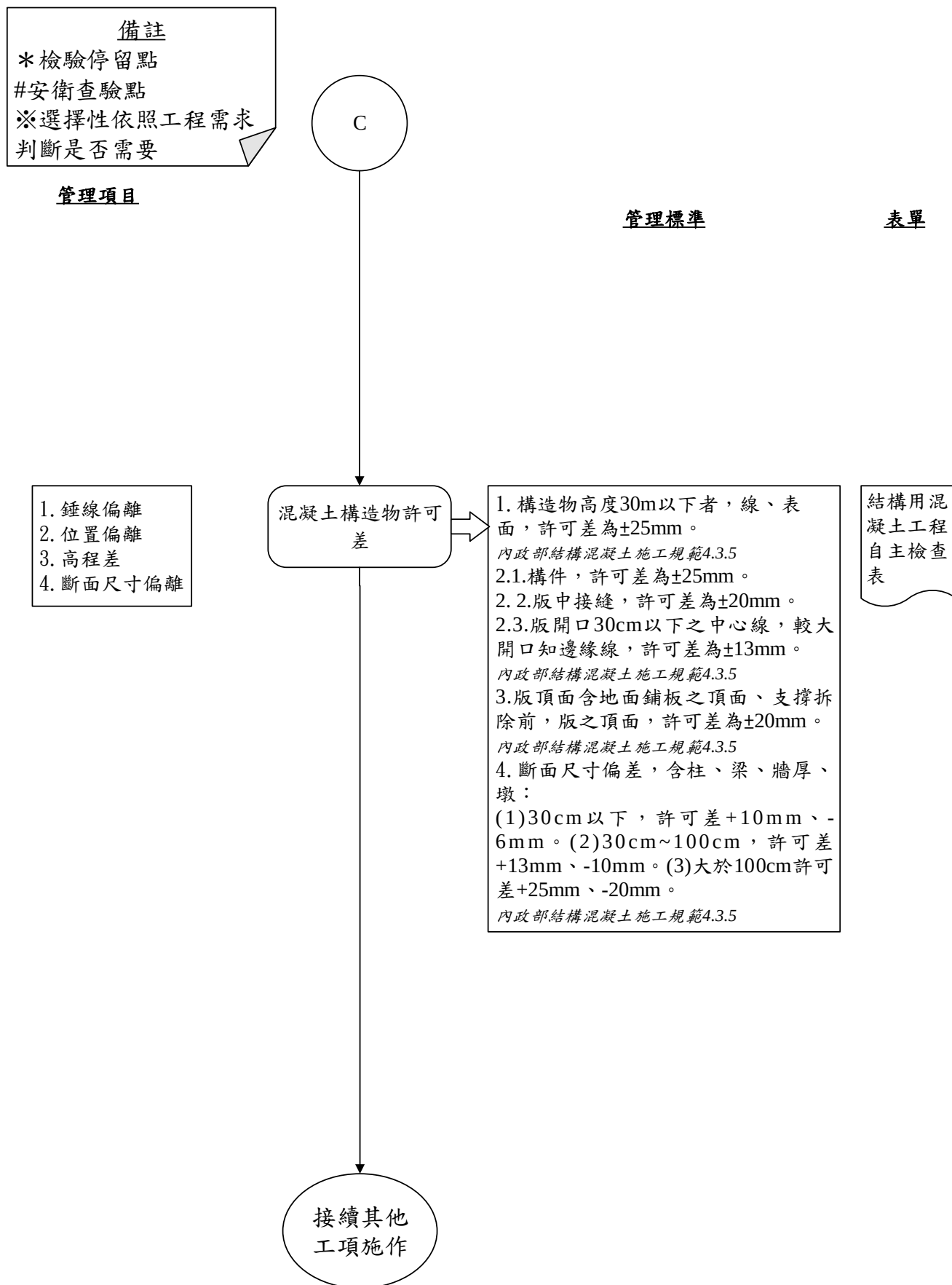
圖 033101-QCF- 4 結構用混凝土工程施工檢驗流程圖 4/4
