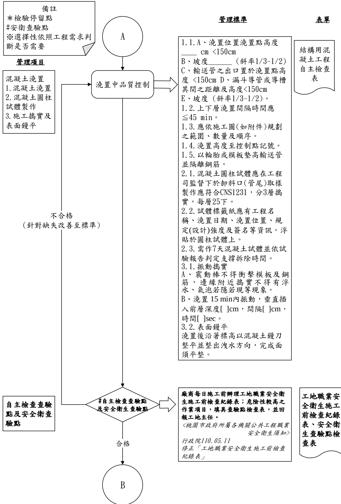
圖 033101-QCF- 2 結構用混凝土工程施工檢驗流程圖 2/4
