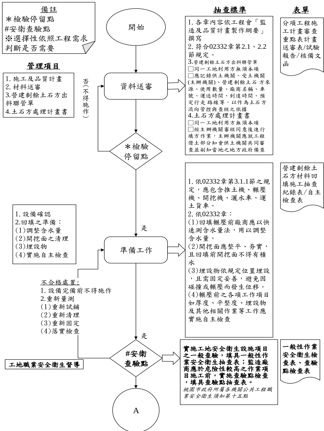
圖 023320-F-1 營建剩餘土石方材料回填施工抽查流程圖 1/3
