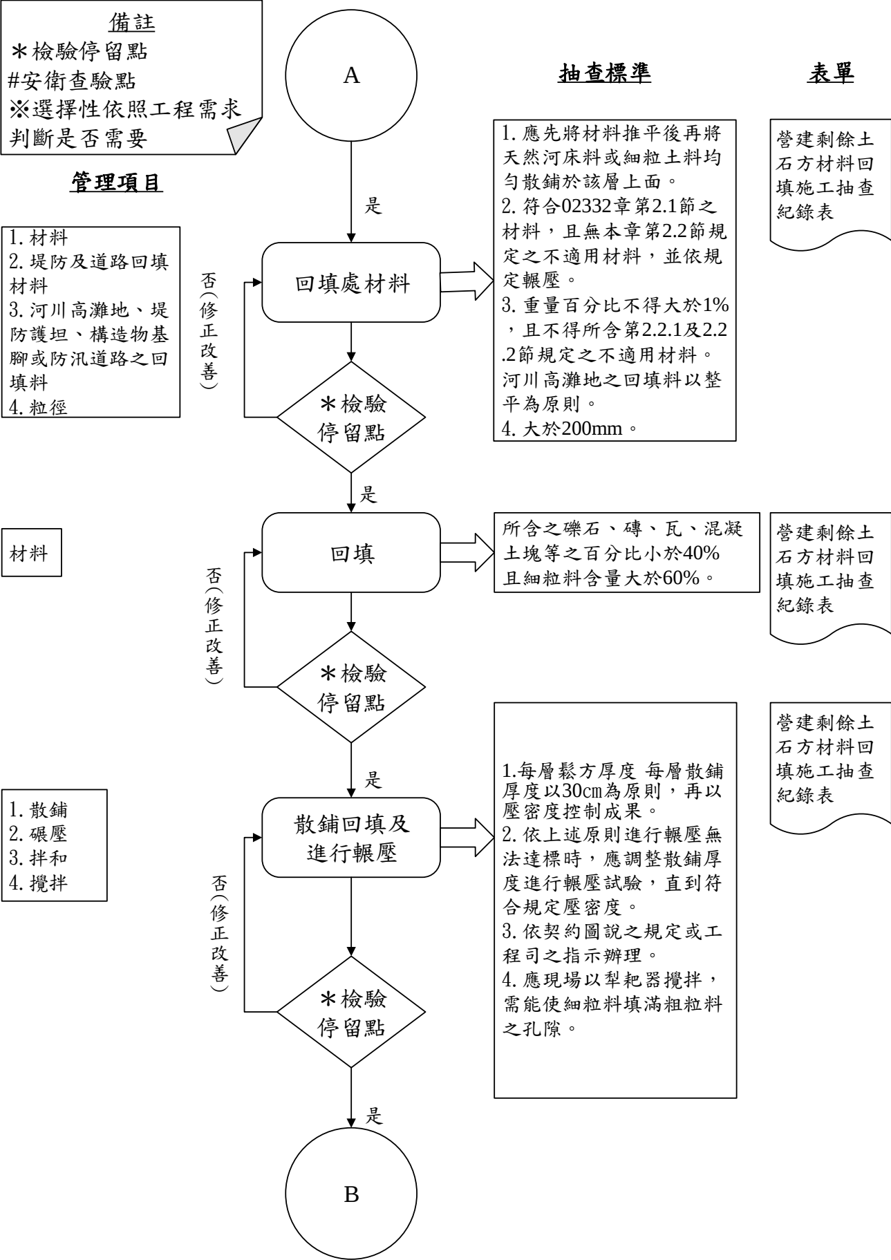
圖 023320-F-2 營建剩餘土石方材料回填施工抽查流程圖 2/3
