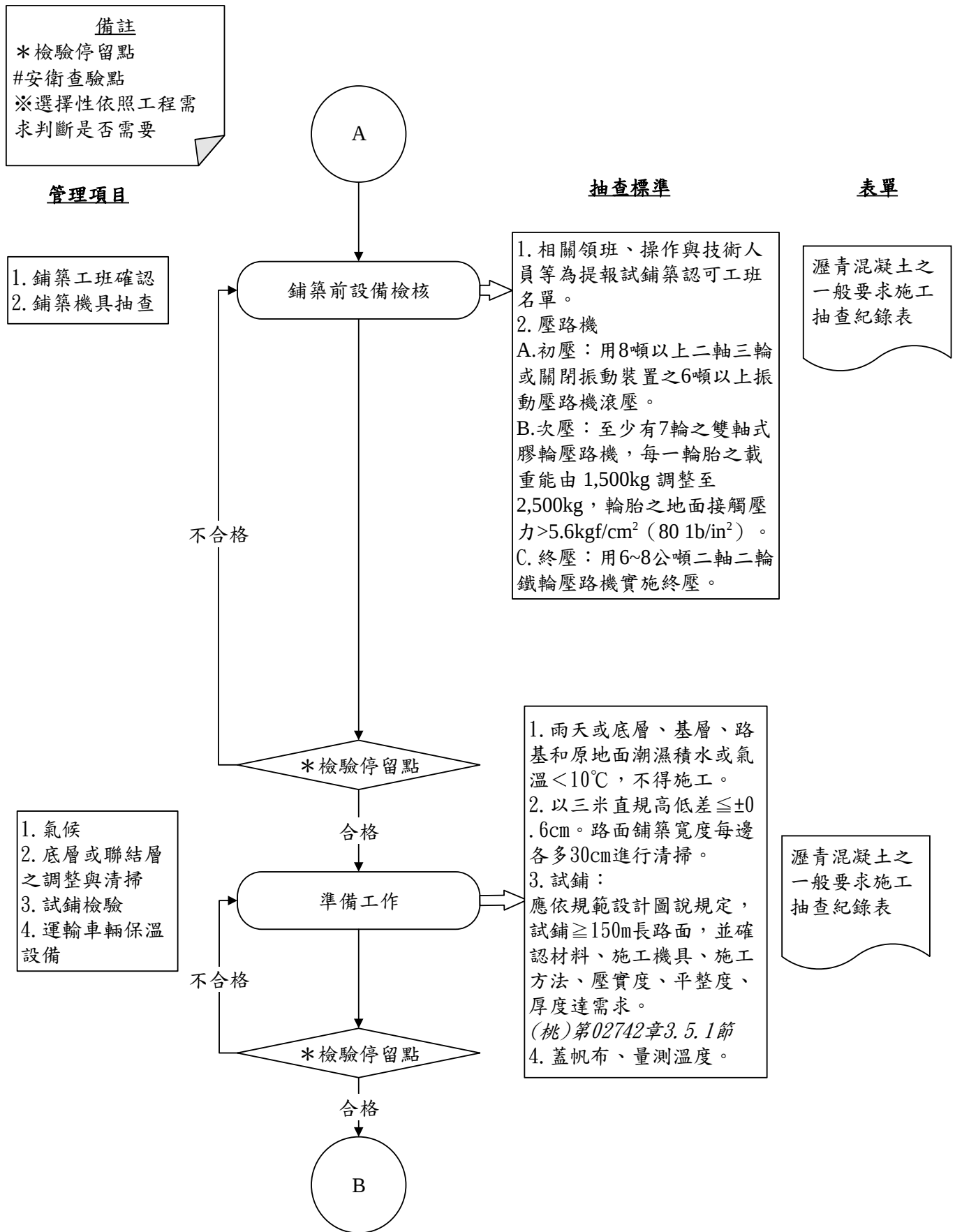
圖 027412-F-1 瀝青混凝土之一般要求施工抽查流程圖 2/5
