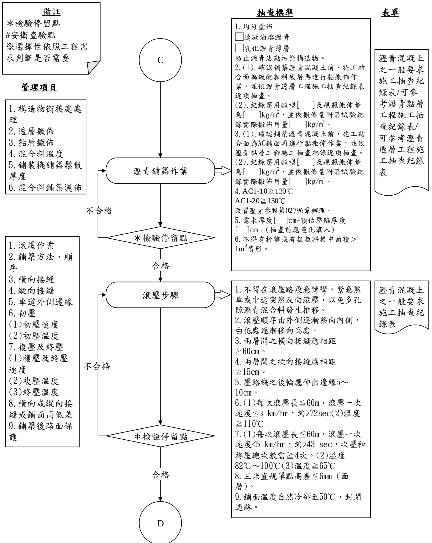
圖 027412-F-1 瀝青混凝土之一般要求施工抽查流程圖 4/5
