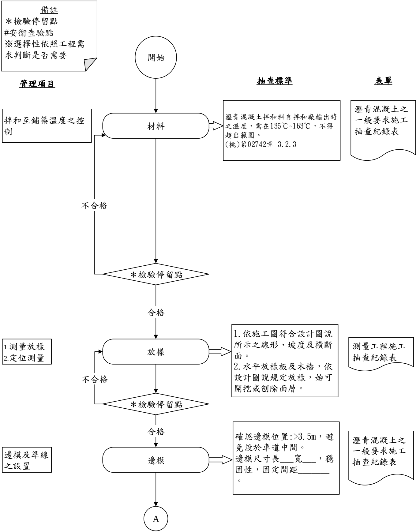
圖 027412-F-1 瀝青混凝土之一般要求施工抽查流程圖 1/5
