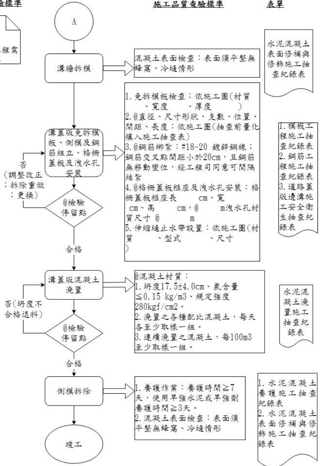
圖 026350-F-1 道路蓋版邊溝施工抽查流程圖 2/2
