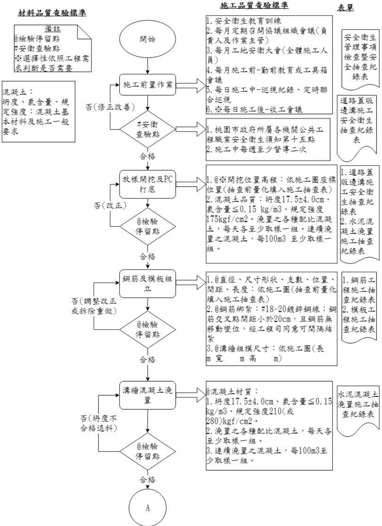
圖 026350-F-1 道路蓋版邊溝施工抽查流程圖 1/2
