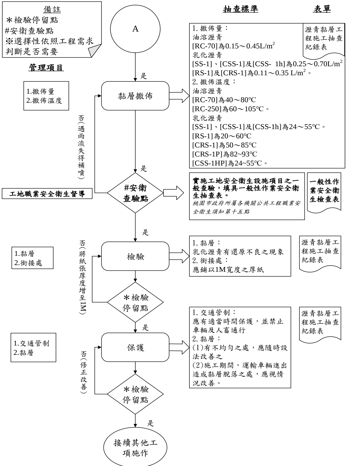
圖 027470-F-2 瀝青黏層施工抽查流程圖 2/2
