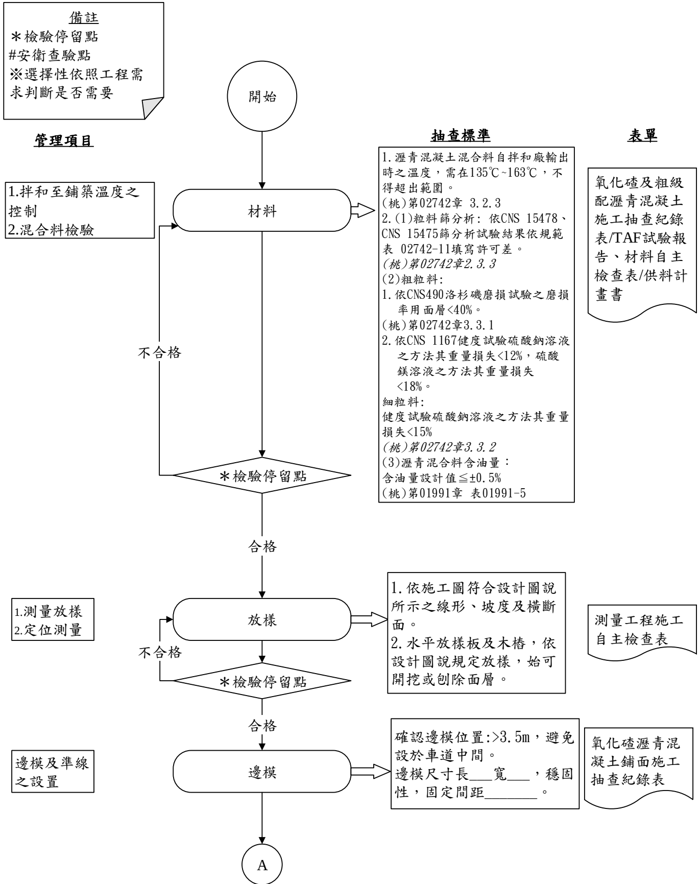
圖 027022-F-1 氧化碇瀝青混凝土鋪面施工抽查流程圖 1/5
