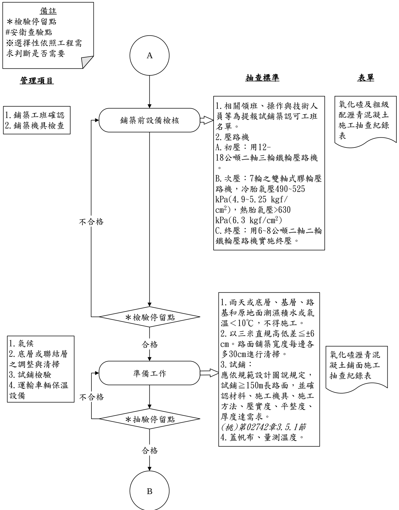
圖 027022-F-1 氧化矽瀝青混凝土鋪面施工抽查流程圖 2/5
