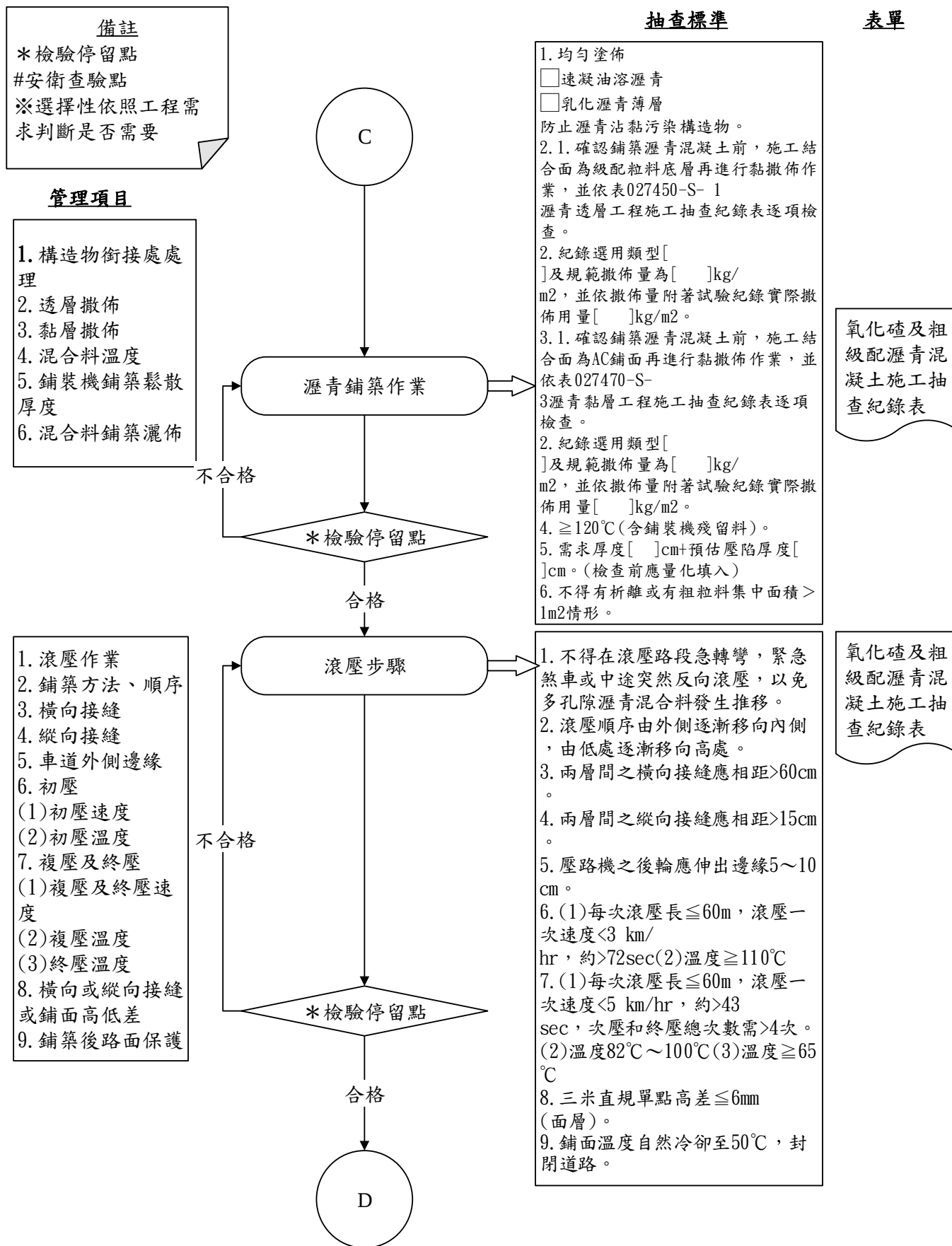
圖 027022-F-1 氧化碇瀝青混凝土鋪面施工抽查流程圖 4/5
