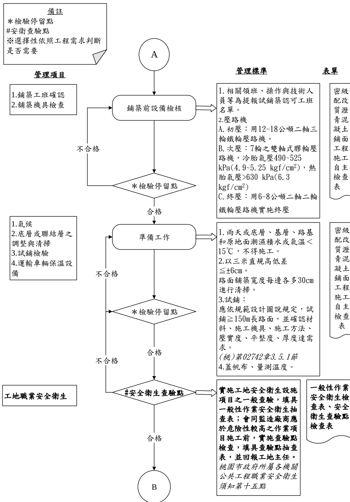
圖 027961-QCF-1 密級配改質瀝青混凝土鋪面工程施工檢驗流程圖 2/5
