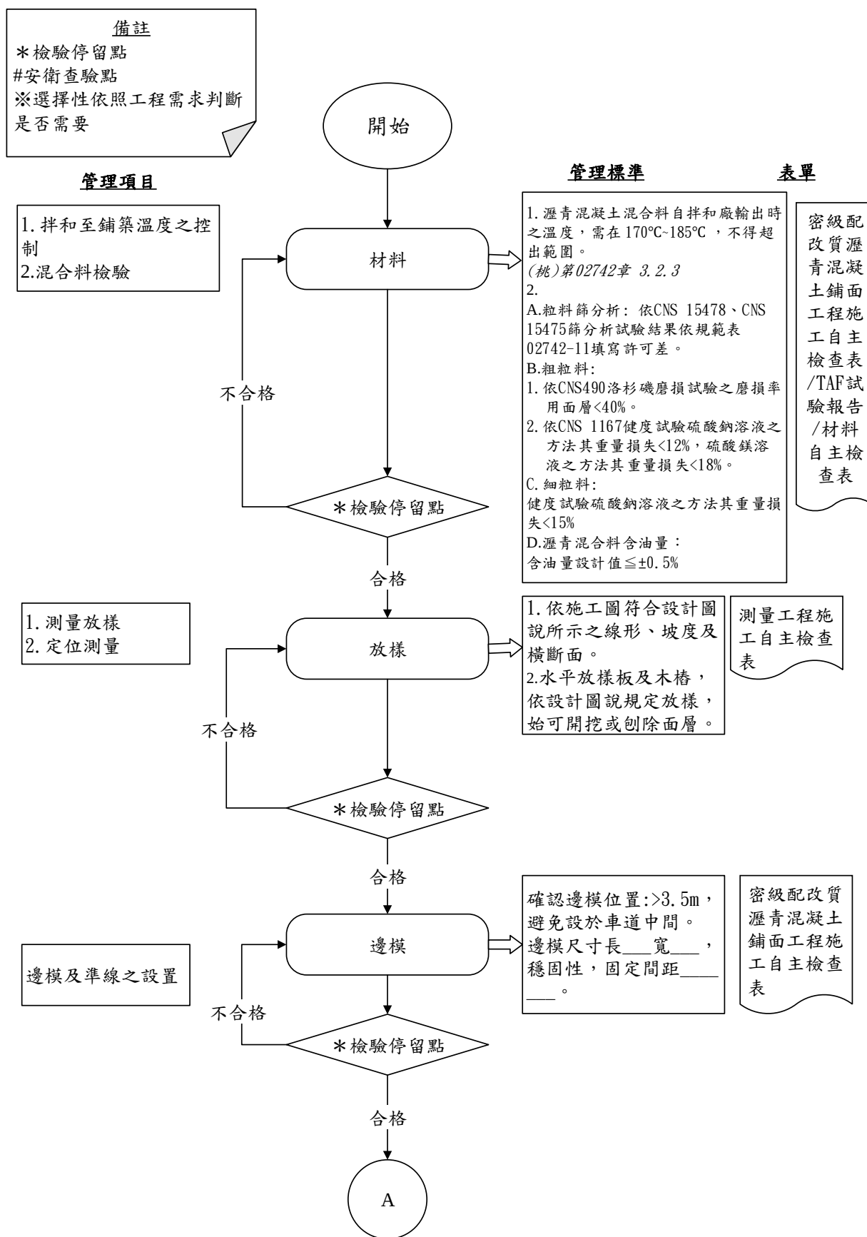
圖 027961-QCF-1 密級配改質瀝青混凝土鋪面工程施工檢驗流程圖 1/5
