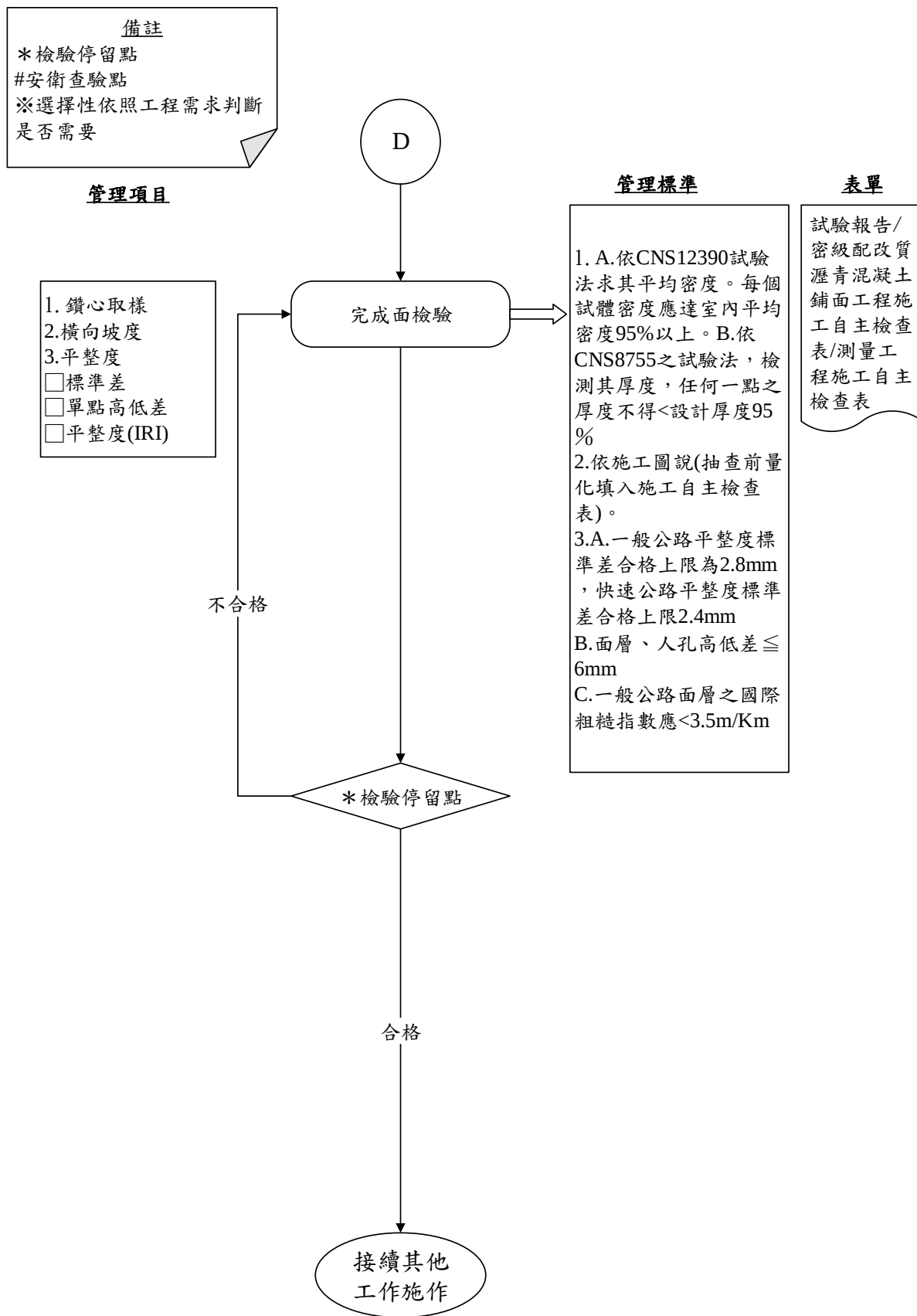
圖 027961-QCF-1 密級配改質瀝青混凝土鋪面工程施工檢驗流程圖 5/5
