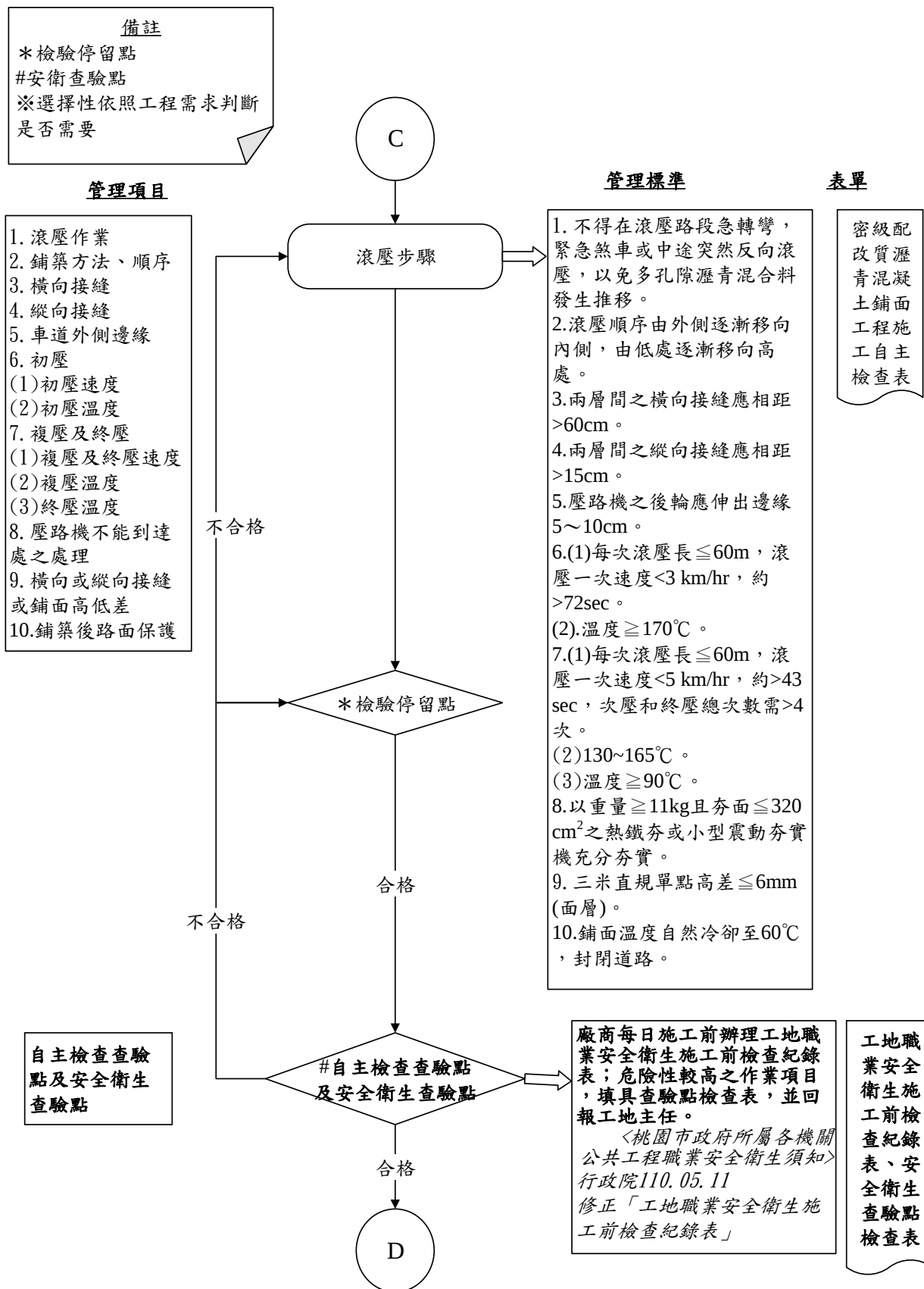
圖 027961-QCF-1 密級配改質瀝青混凝土鋪面工程施工檢驗流程圖 4/5
