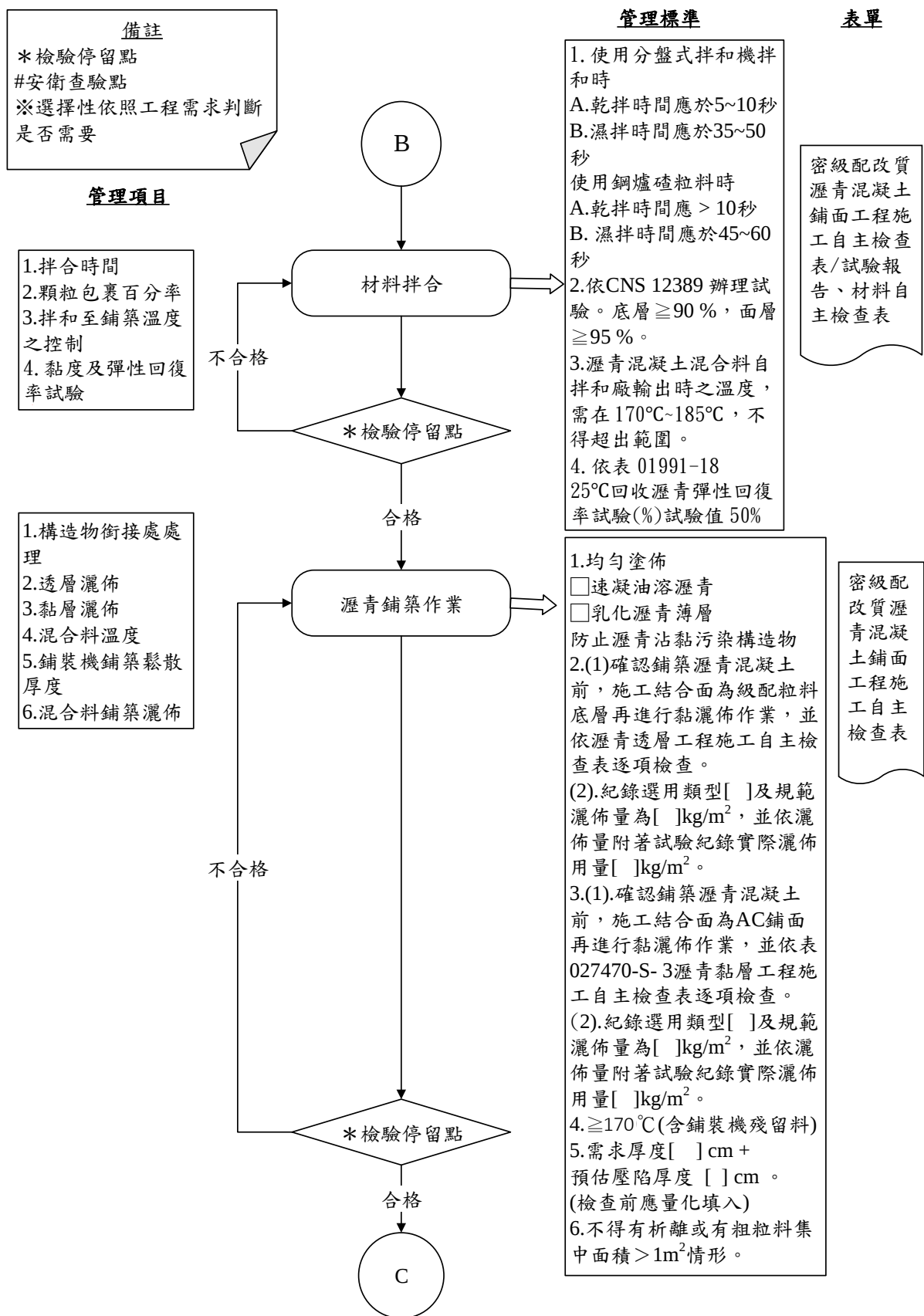
圖 027961-QCF-1 密級配改質瀝青混凝土鋪面工程施工檢驗流程圖 3/5
