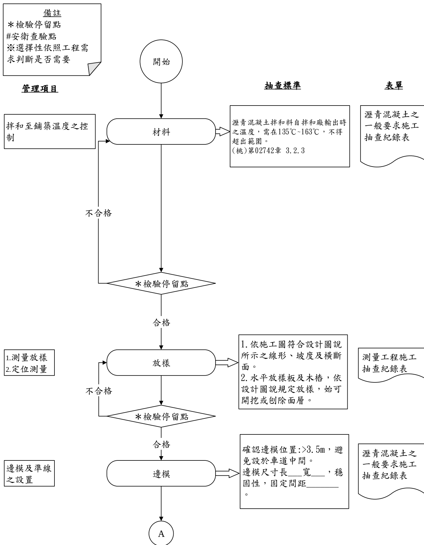
圖 027422-F-1 瀝青混凝土鋪面施工抽查流程圖 1/5
