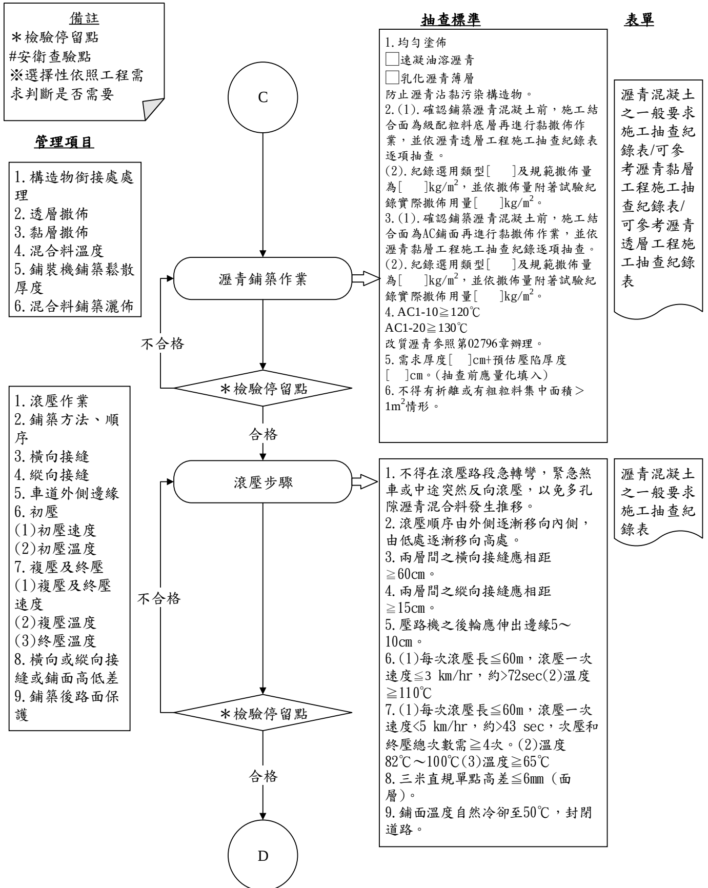
圖 027422-F-1 瀝青混凝土鋪面施工抽查流程圖 4/5
