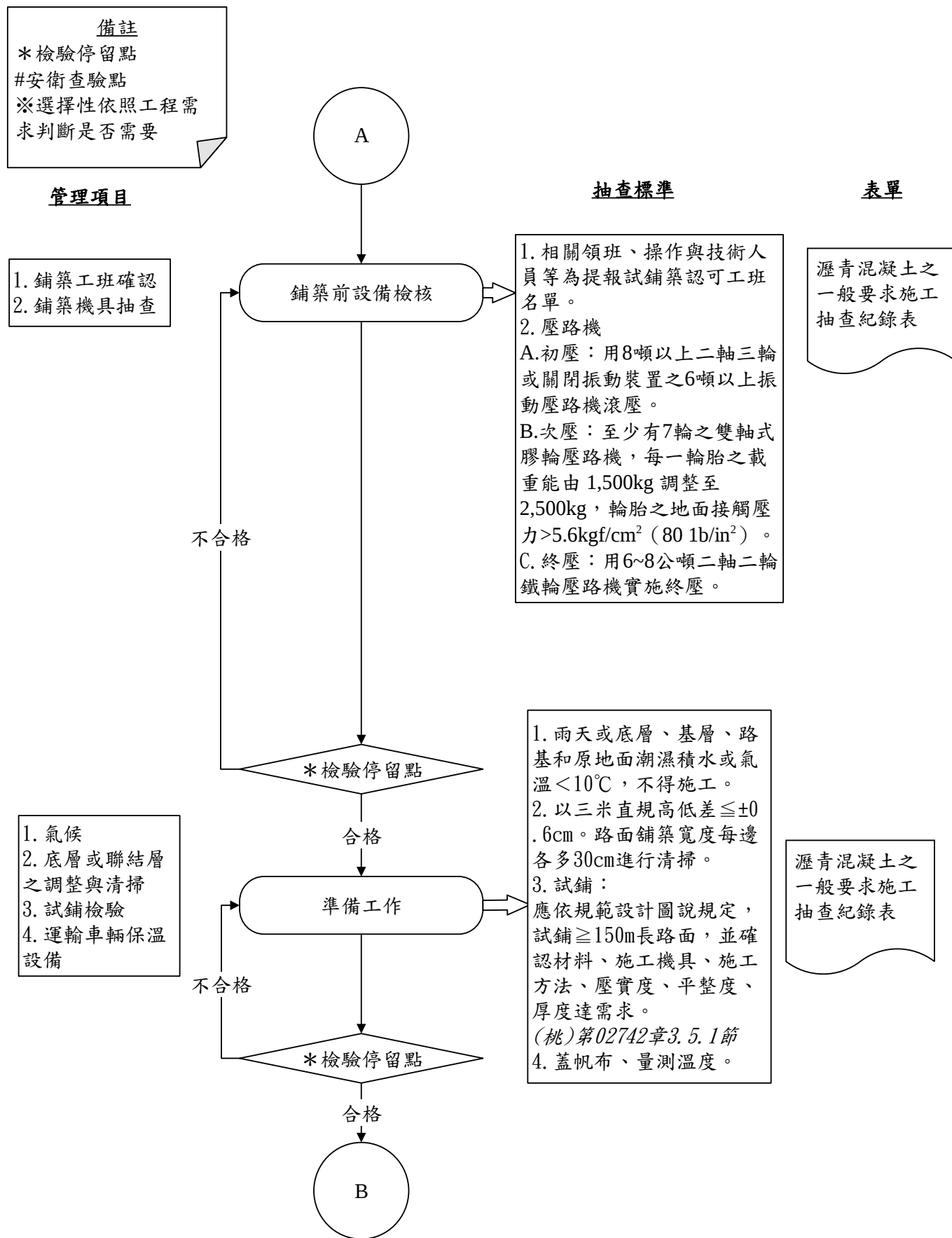
圖 027422-F-1 瀝青混凝土鋪面施工抽查流程圖 2/5
