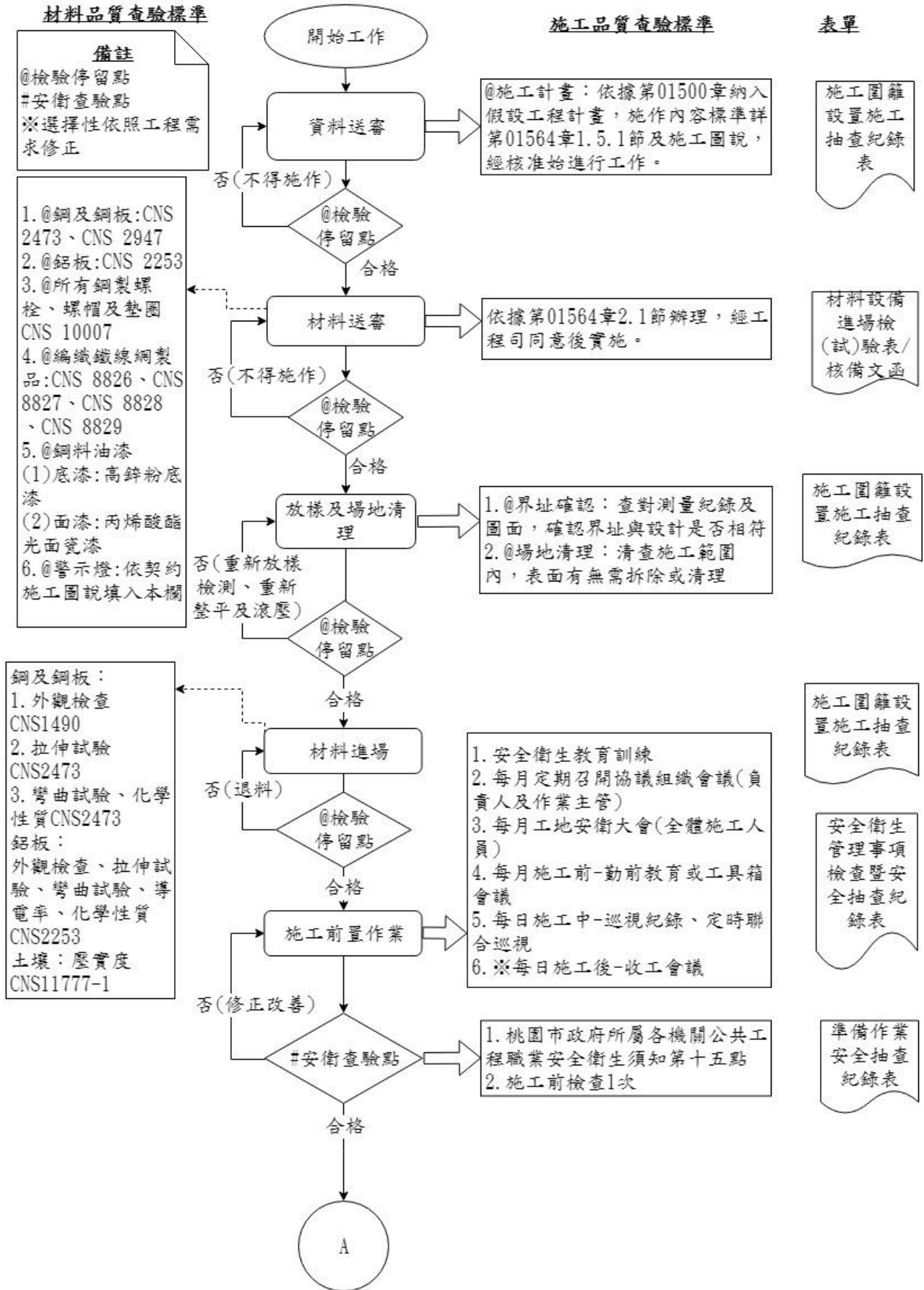
圖 015640-F-1 施工圍籬施工抽查流程圖 1/2
