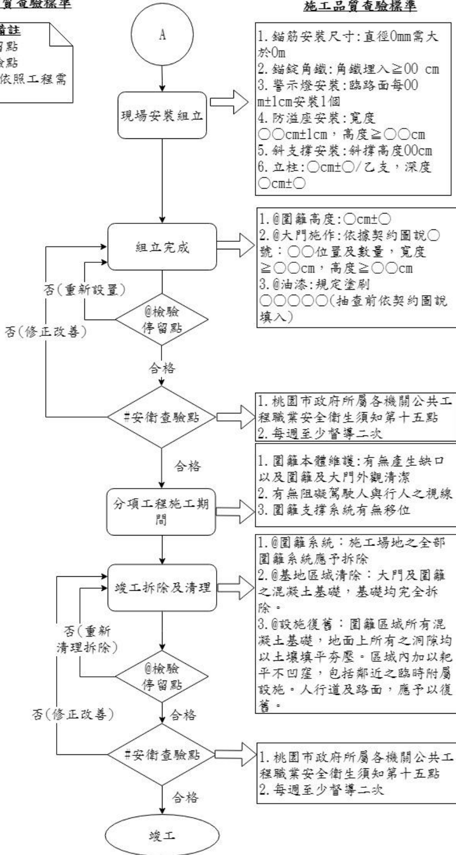
圖 015640-F-1 施工圍籬施工抽查流程圖 2/2
