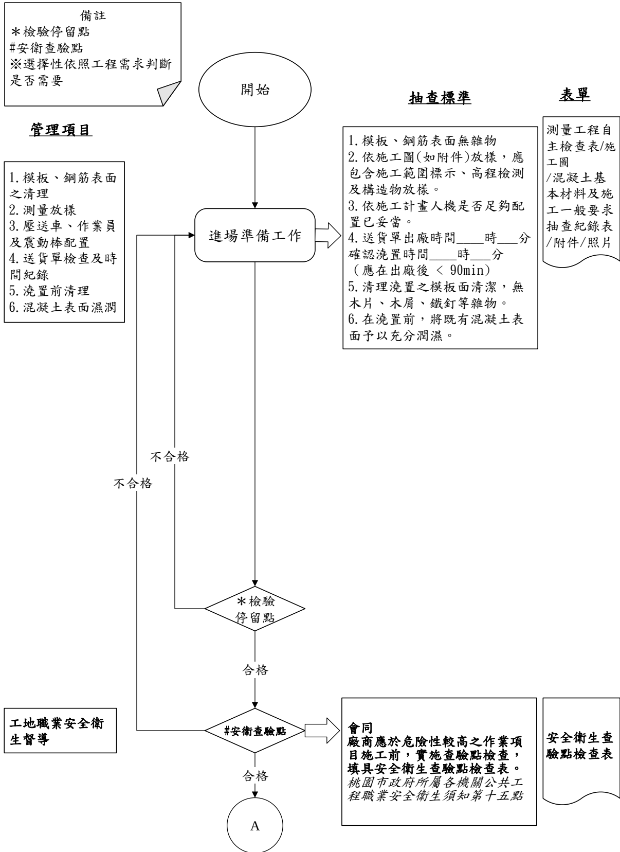
圖 030502-F-1 混凝土基本材料及施工一般要求施工流程圖 1/4
