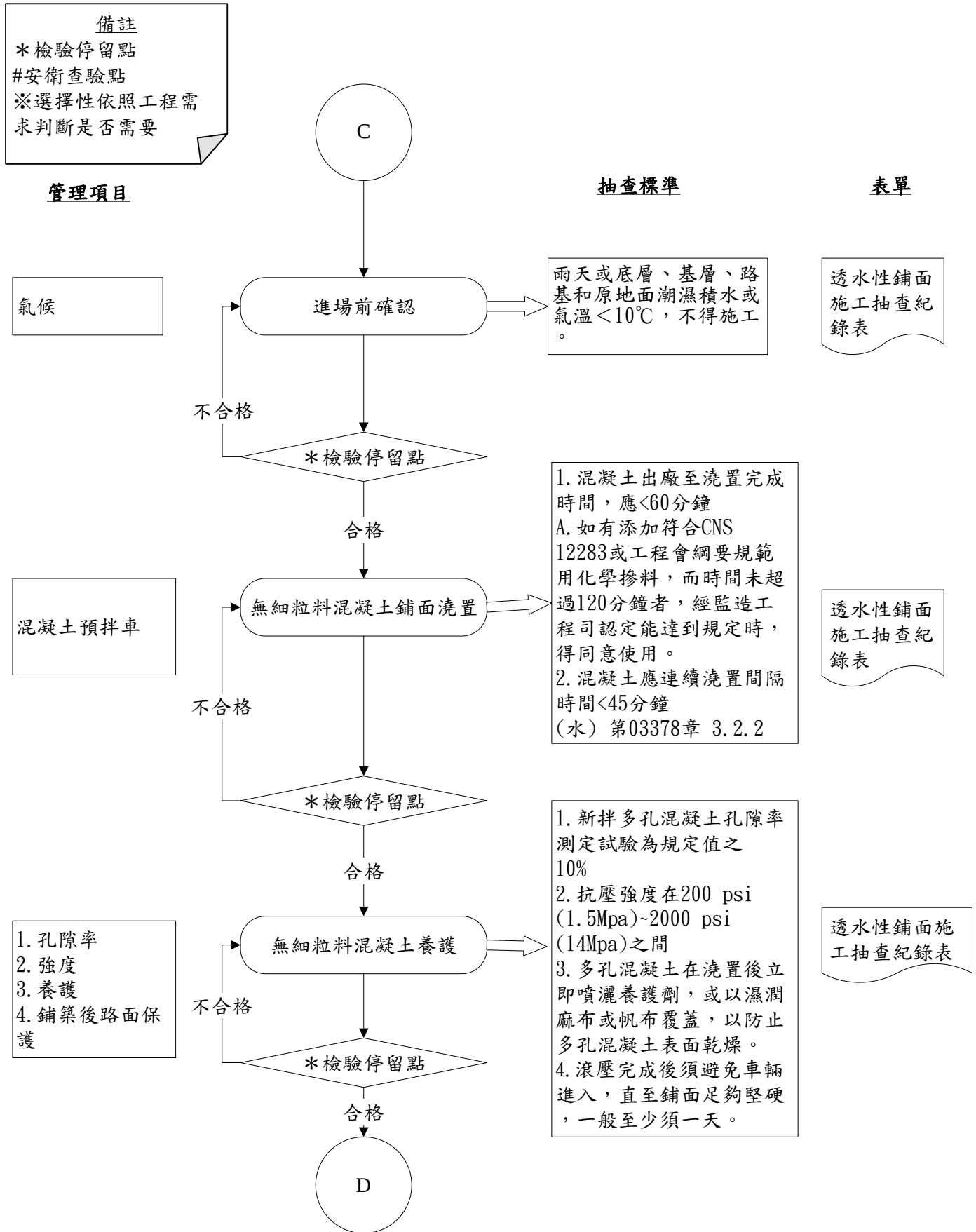
圖 027942-F-1 透水性鋪面工程施工抽查流程圖 4/6
