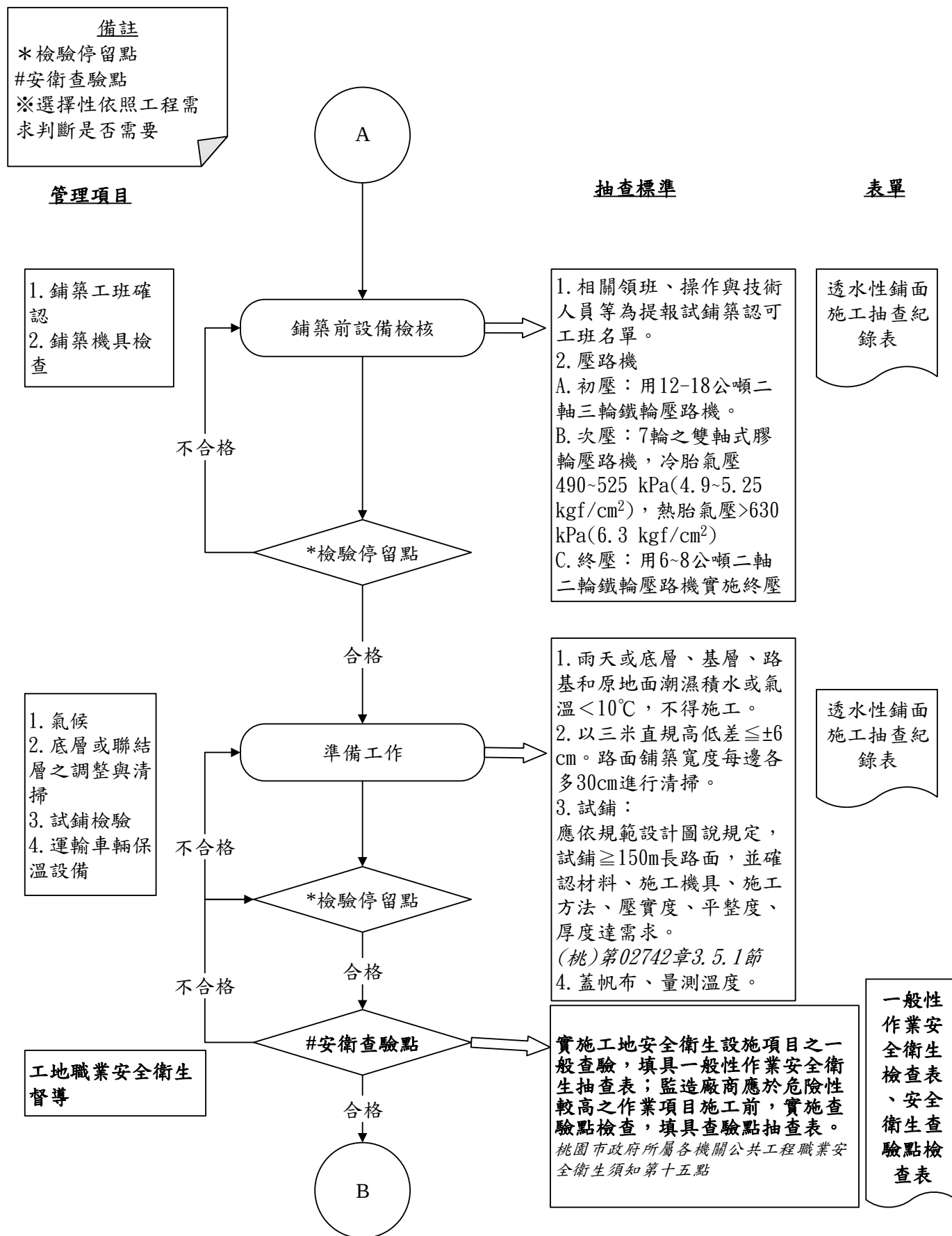
圖 027942-F-1 透水性鋪面工程施工抽查流程圖 2/6
