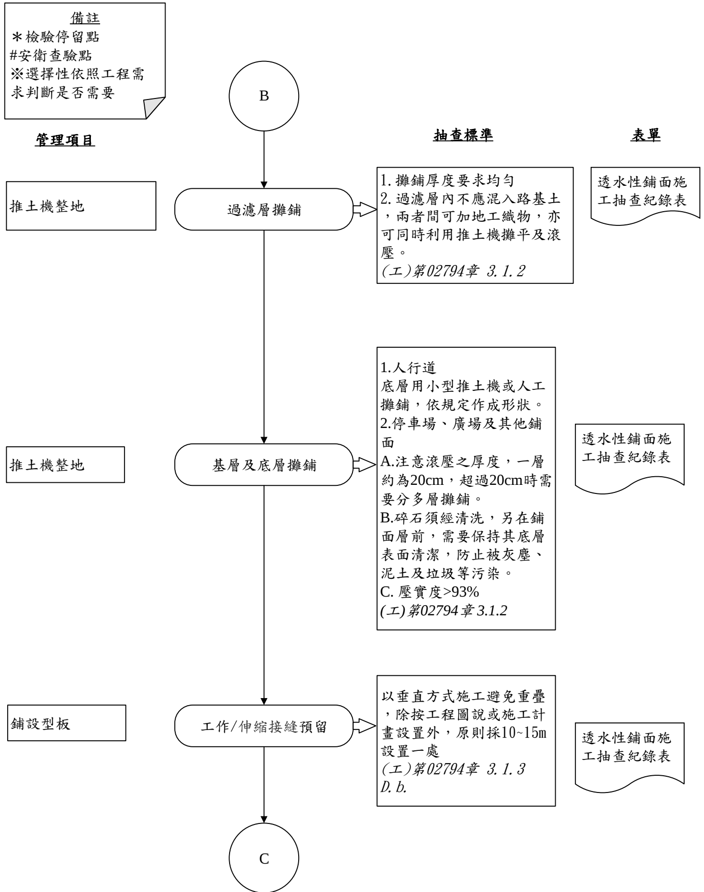
圖 027942-F-1 透水性鋪面工程施工抽查流程圖 3/6
