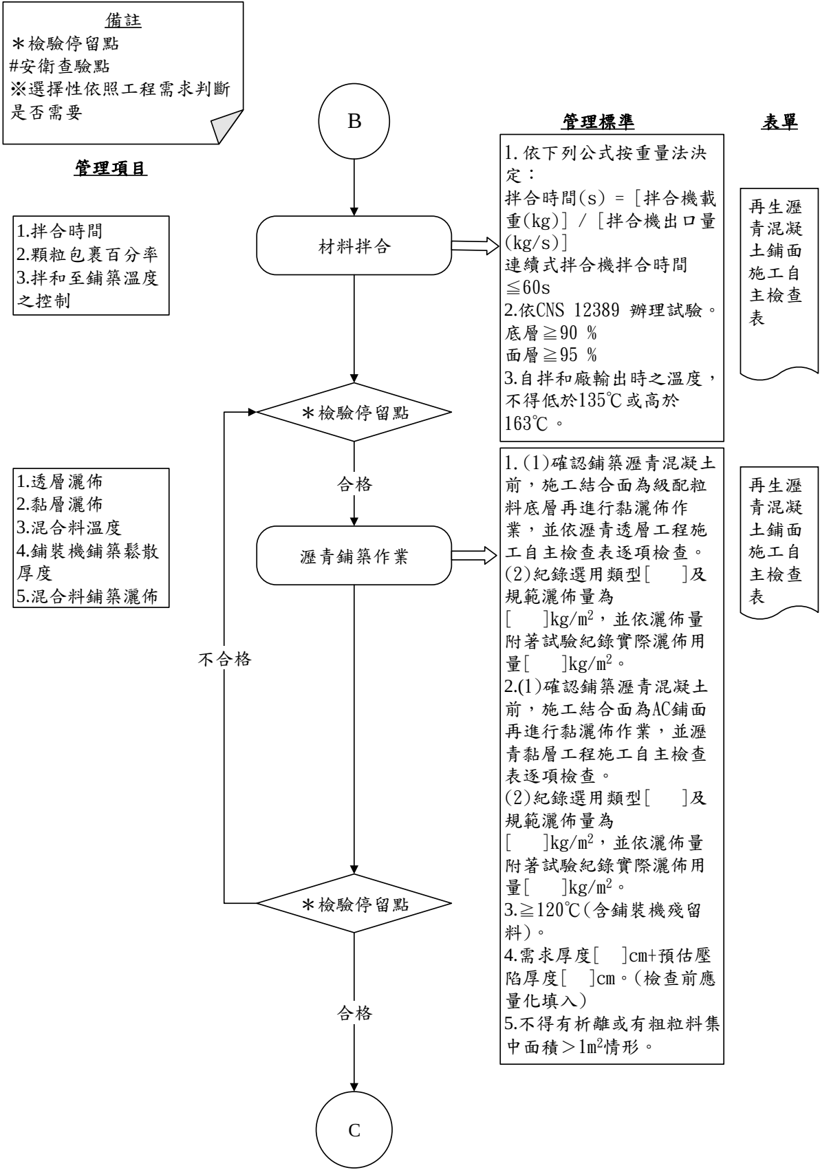
圖 029661-QCF-1 再生瀝青混凝土鋪面施工檢驗流程圖 3/5
