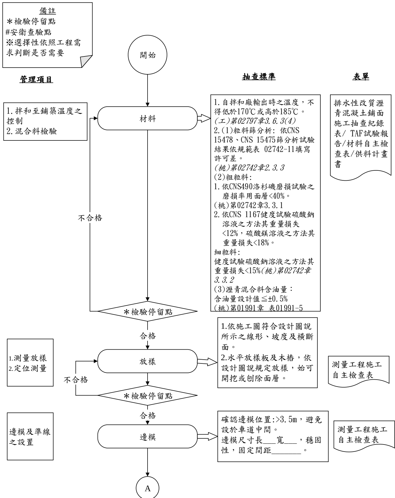
圖 027972-F-1 排水性改質瀝青混凝土鋪面施工抽查流程圖 1/5
