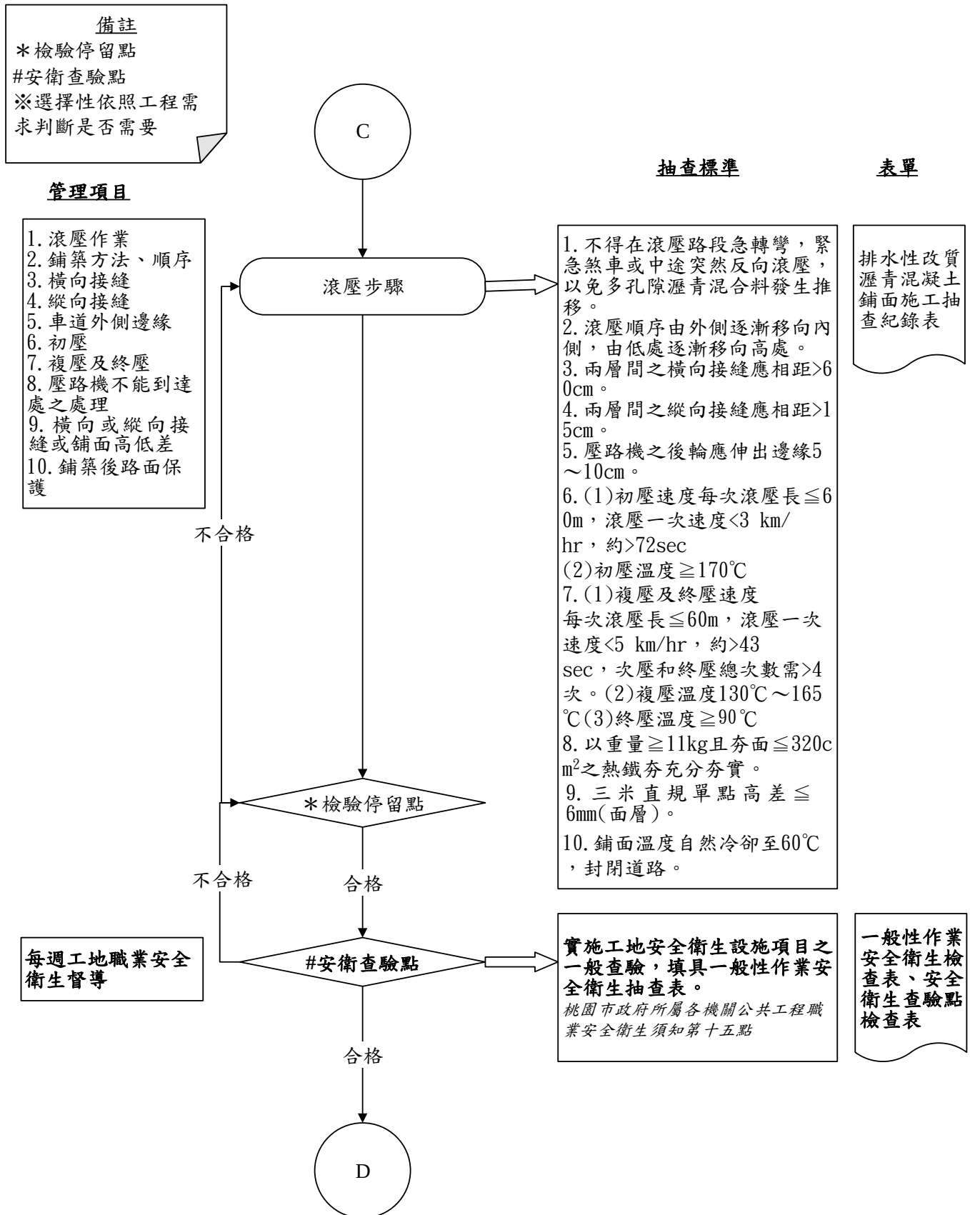
圖 027972-F-1 排水性改質瀝青混凝土鋪面施工抽查流程圖 4/5
