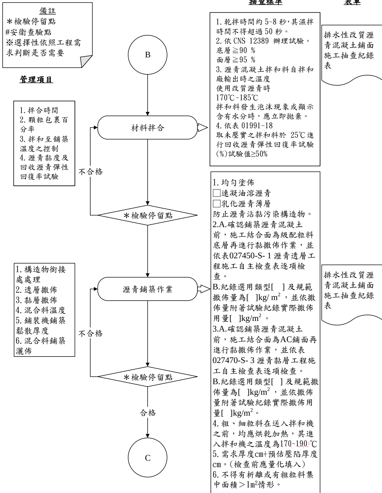
圖 027972-F-1 排水性改質瀝青混凝土鋪面施工抽查流程圖 3/5
