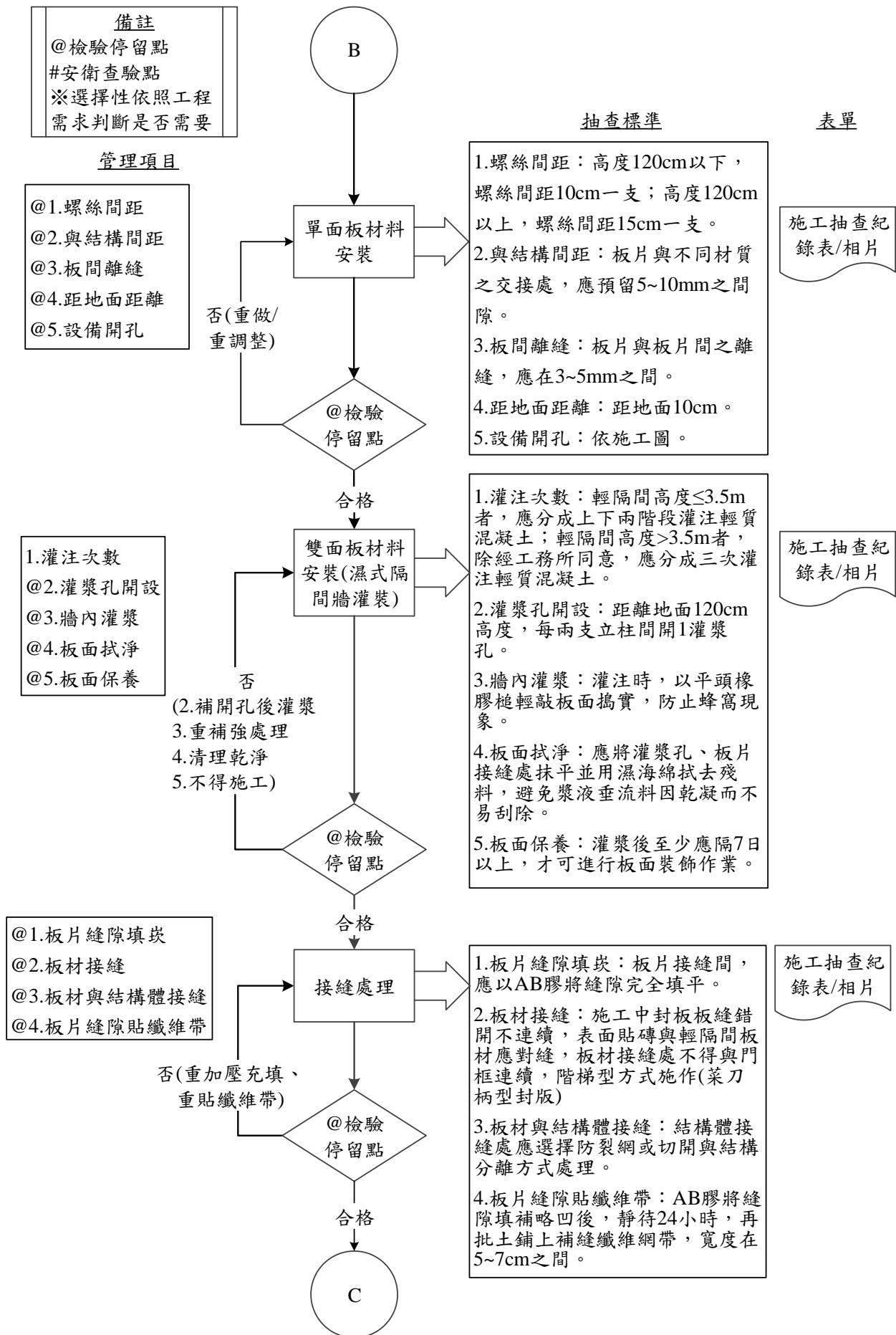
圖 092601-F-1 輕鋼架隔間牆-濕式工程施工抽查流程圖 3/4
