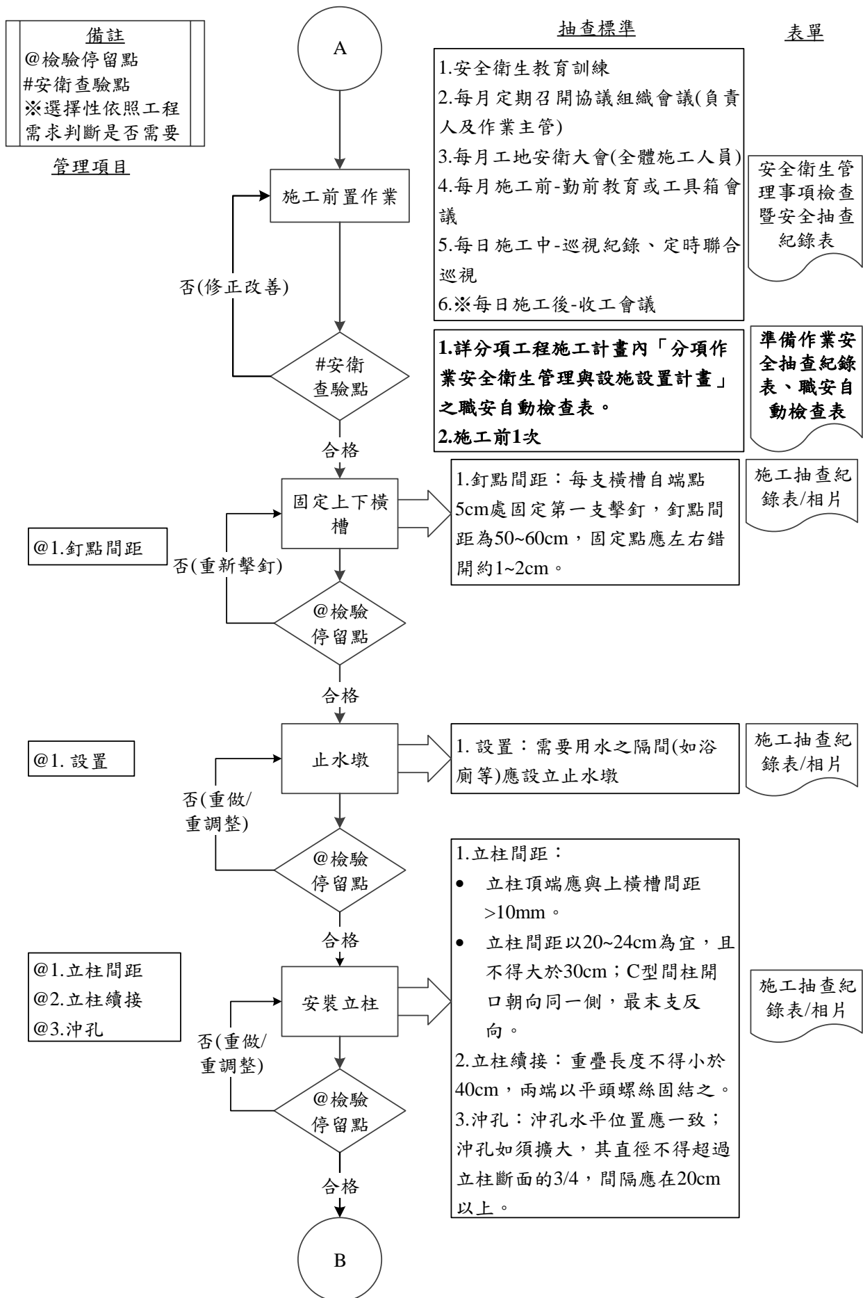
圖 092601-F-1 輕鋼架隔間牆-濕式工程施工抽查流程圖 2/4
