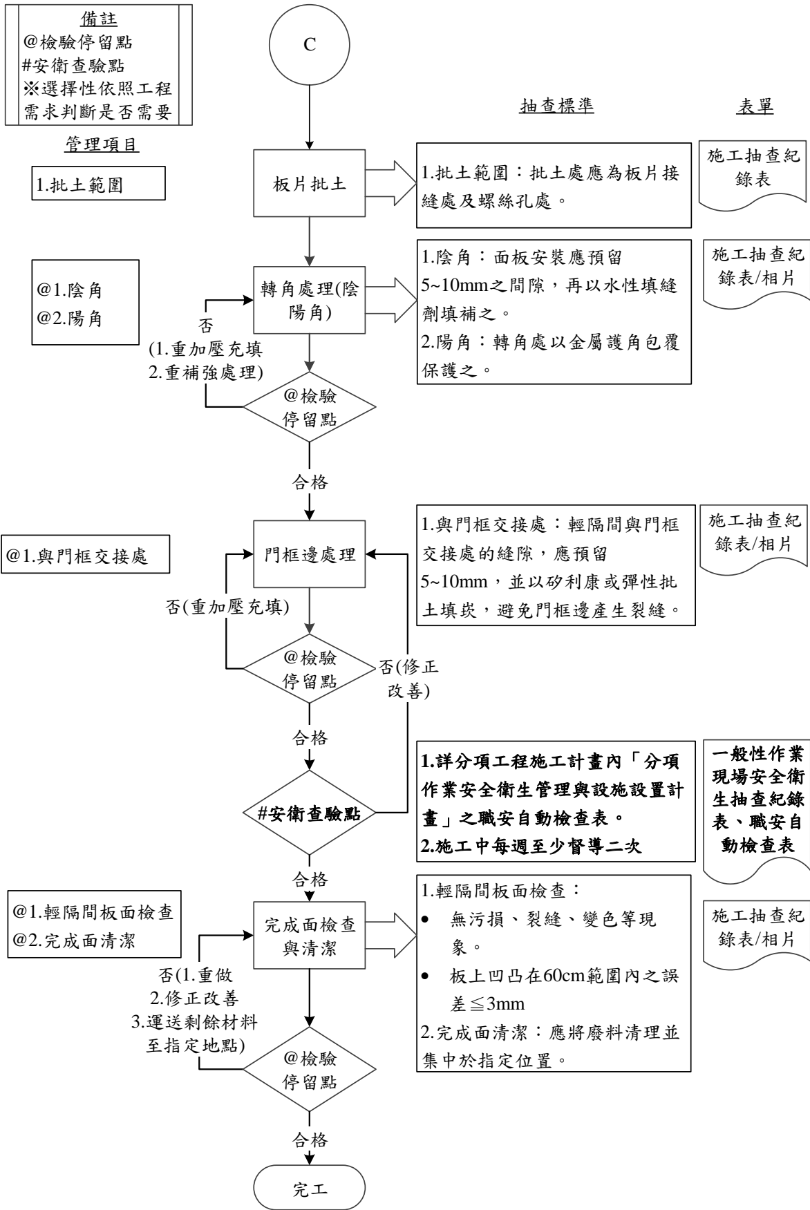
圖 092601-F-1 輕鋼架隔間牆-濕式工程施工抽查流程圖 4/4
