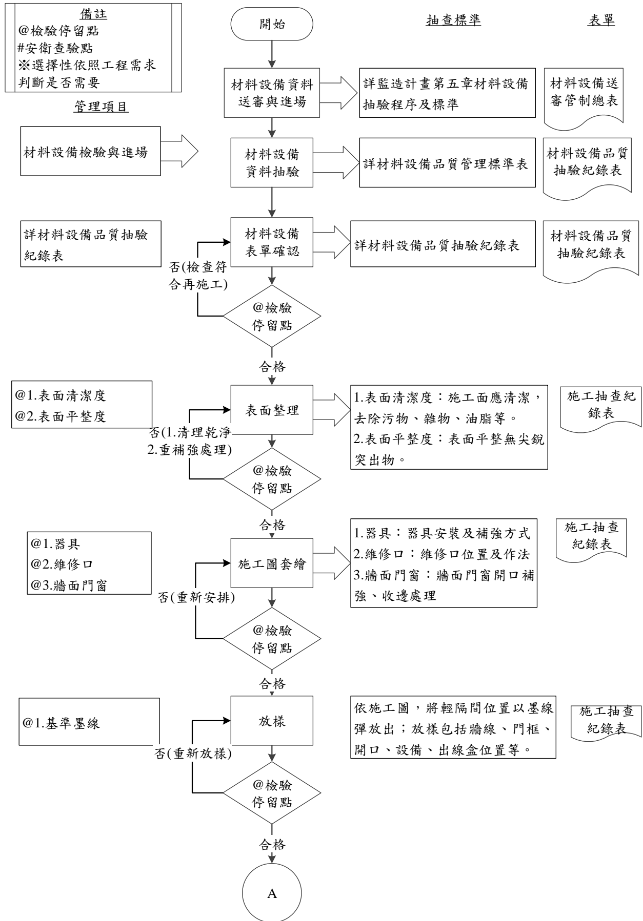
圖 092601-F-1 輕鋼架隔間牆-濕式工程施工抽查流程圖 1/4
