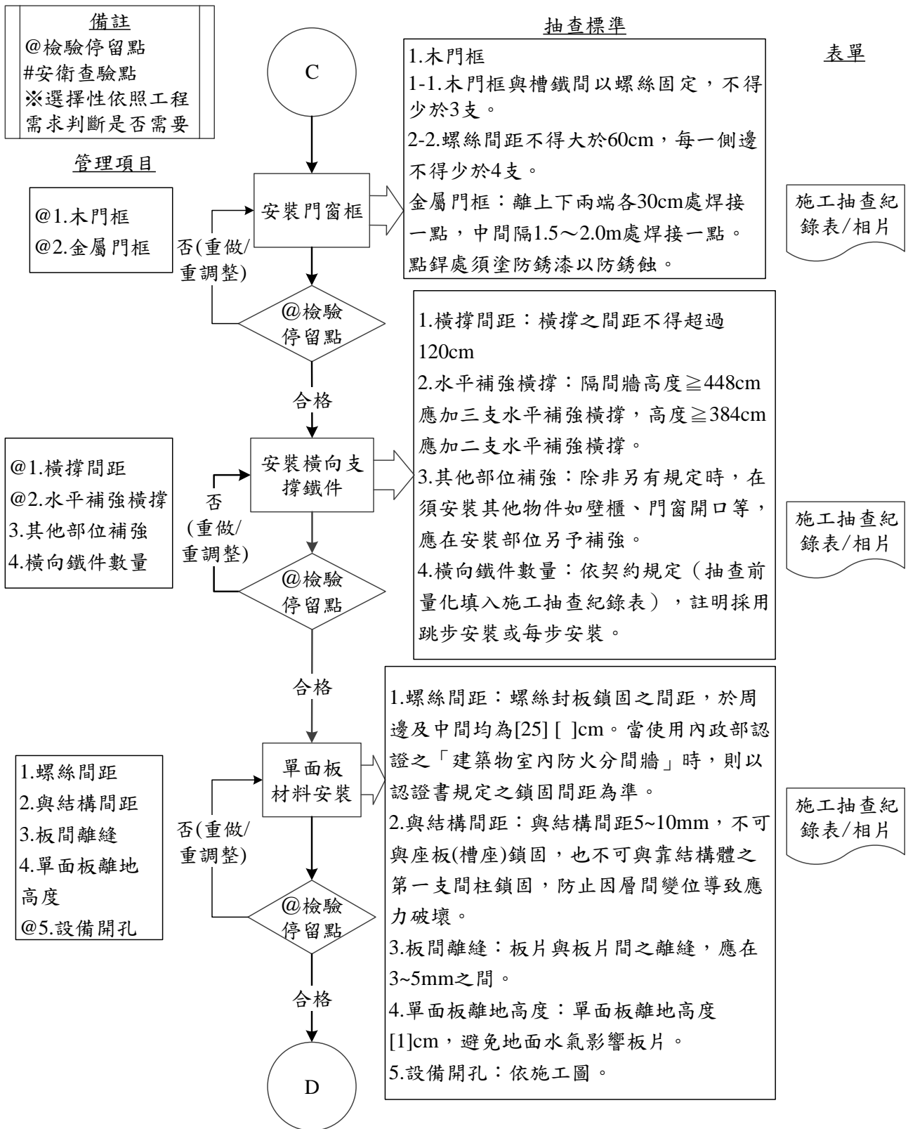
圖 092602-F-1 輕鋼架隔間牆-乾式工程施工抽查流程圖 4/6
