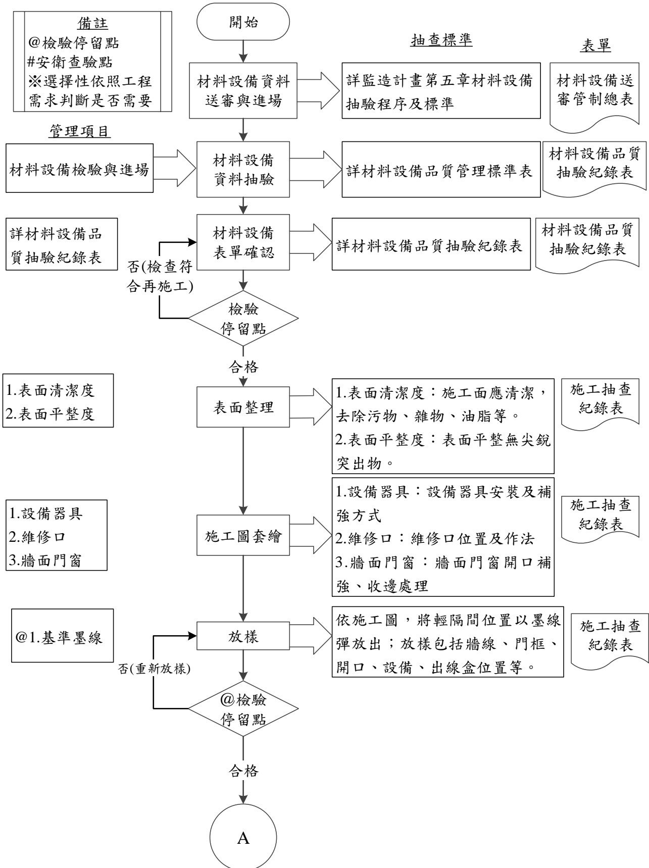
圖 092602-F-1 輕鋼架隔間牆-乾式工程施工抽查流程图 1/6
