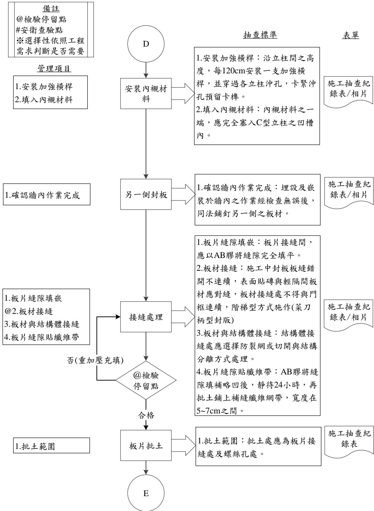
圖 092602-F-1 輕鋼架隔間牆-乾式工程施工抽查流程圖 5/6
