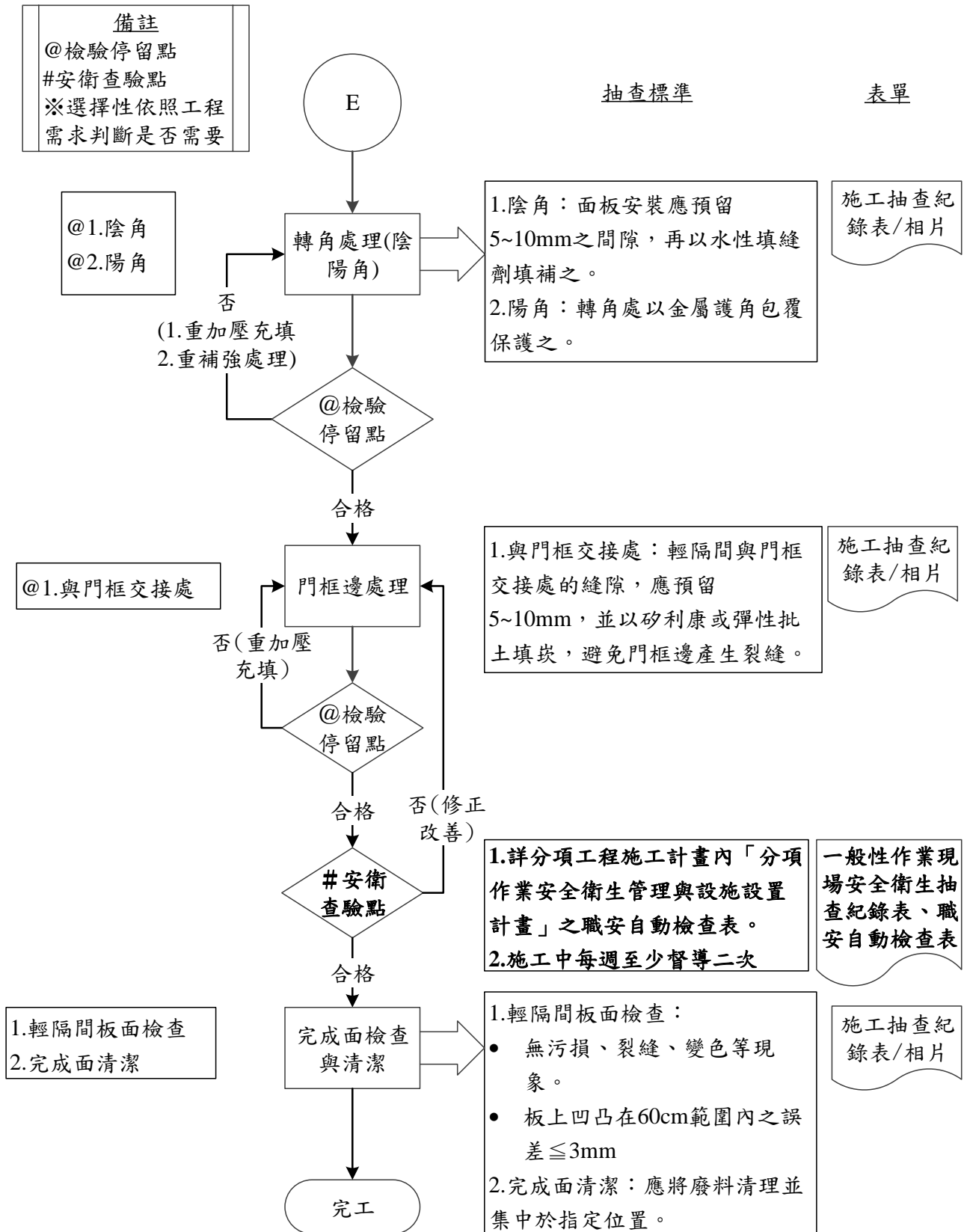
圖 092602-F-1 輕鋼架隔間牆-乾式工程施工抽查流程圖 6/6
