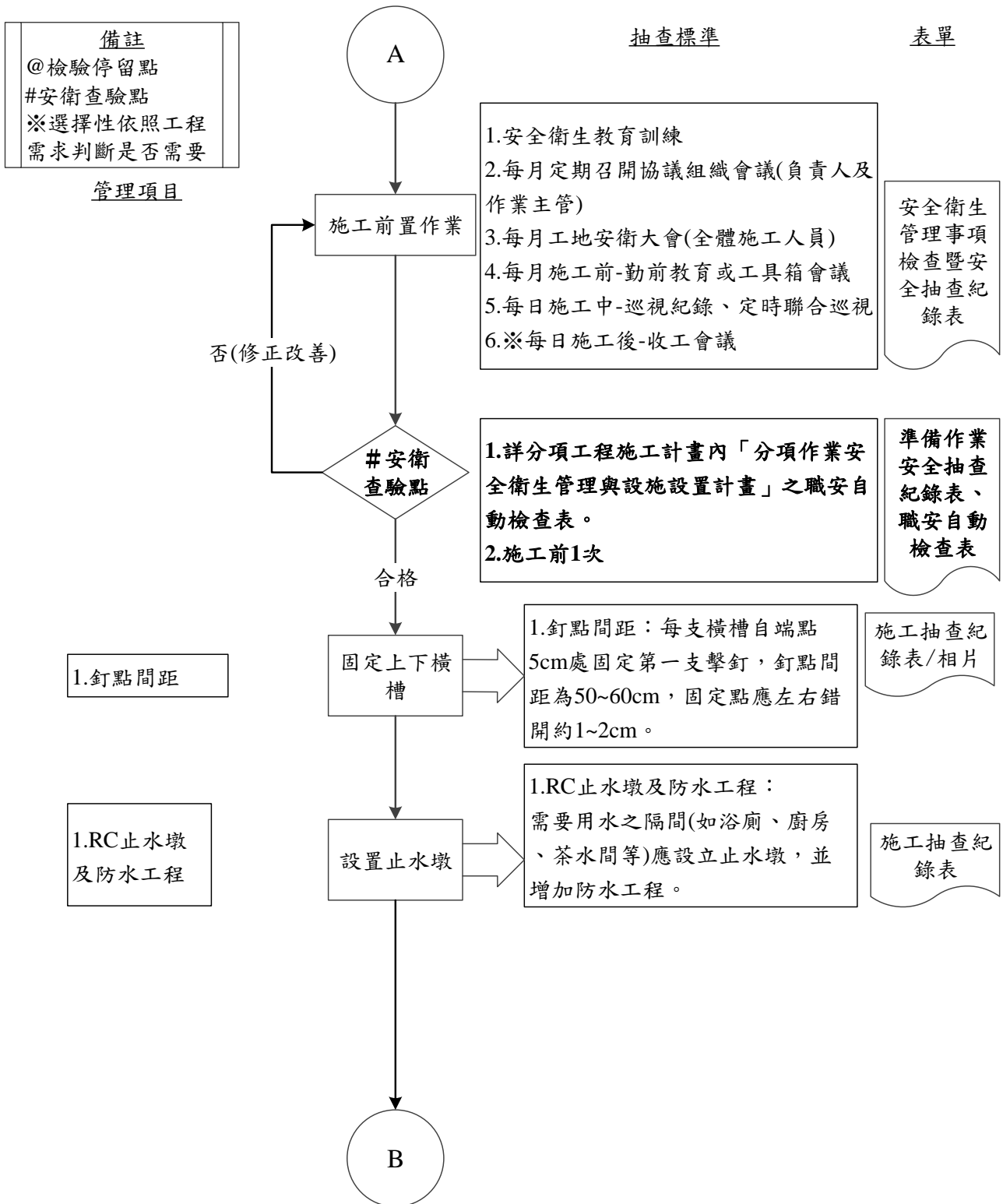
圖 092602-F-1 輕鋼架隔間牆-乾式工程施工抽查流程圖 2/6
