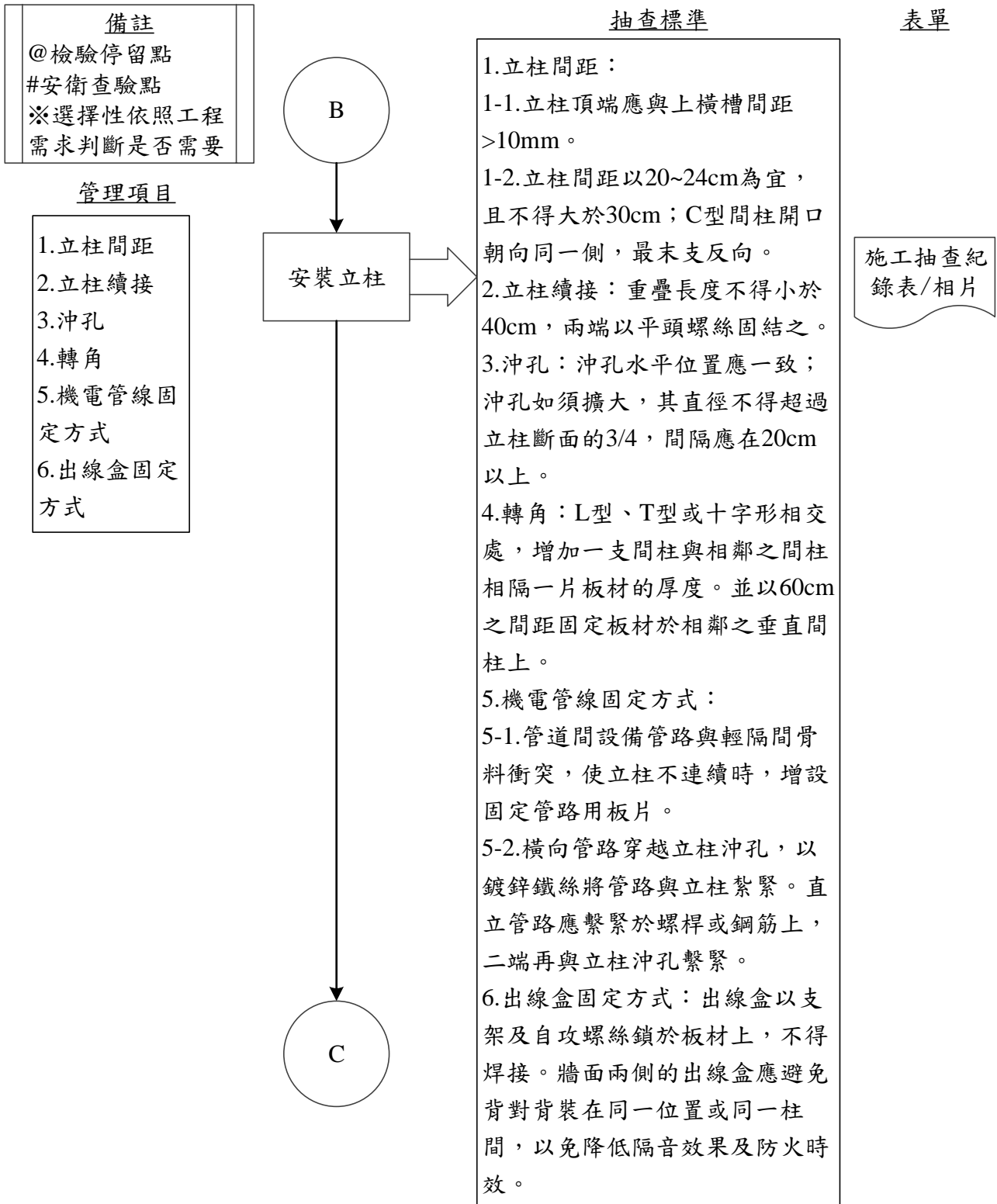
圖 092602-F-1 輕鋼架隔間牆-乾式工程施工抽查流程圖 3/6
