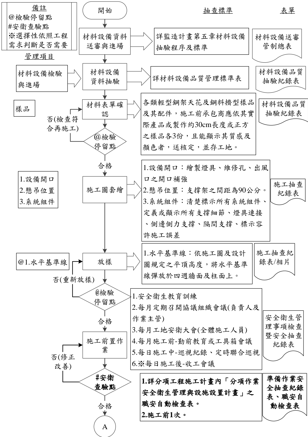
圖 095812-F-1 天花板-明架工程施工抽查流程圖 1/3
