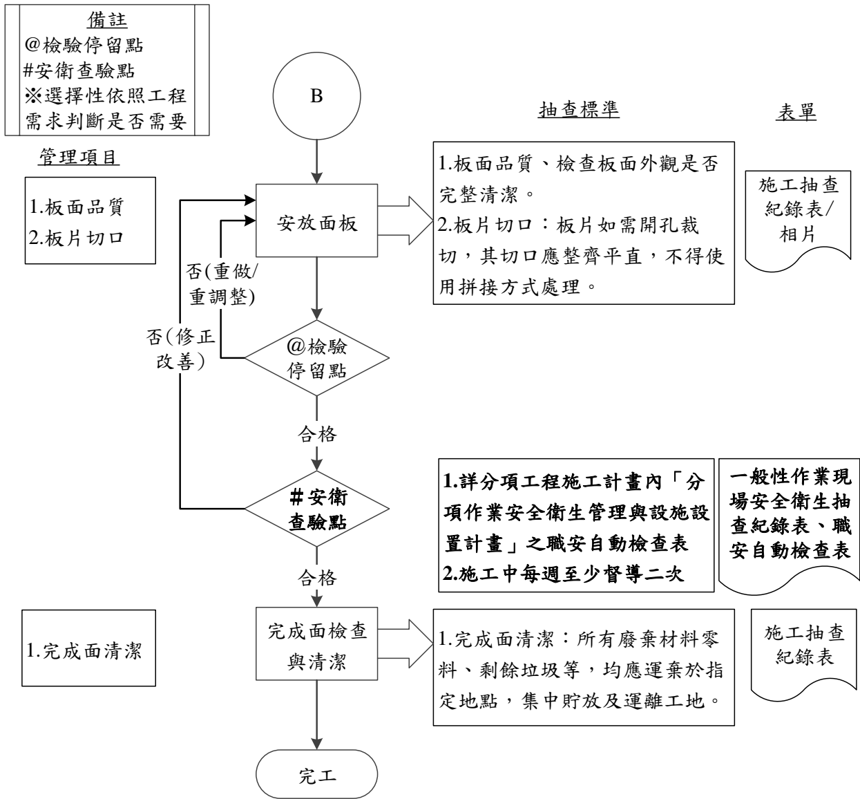
圖 095812-F-1 天花板-明架工程施工抽查流程圖 3/3
