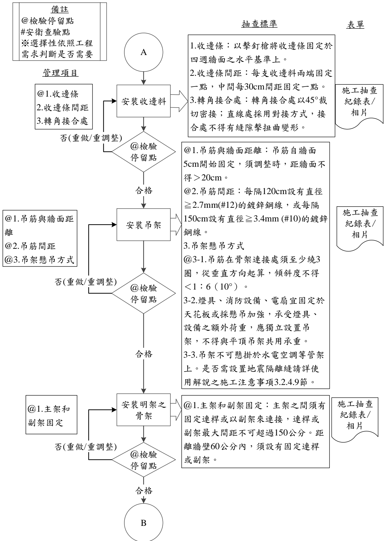
圖 095812-F-1 天花板-明架工程施工抽查流程圖 2/3
