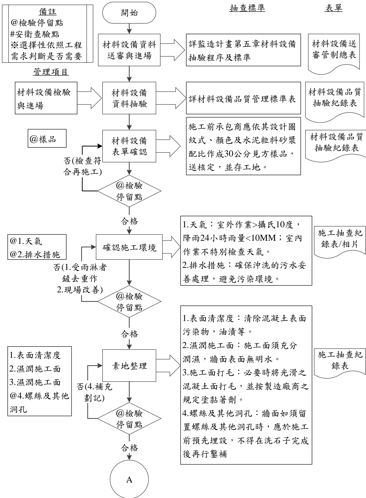
圖 097800-F-1 洗石子工程施工抽查流程圖 1/4
