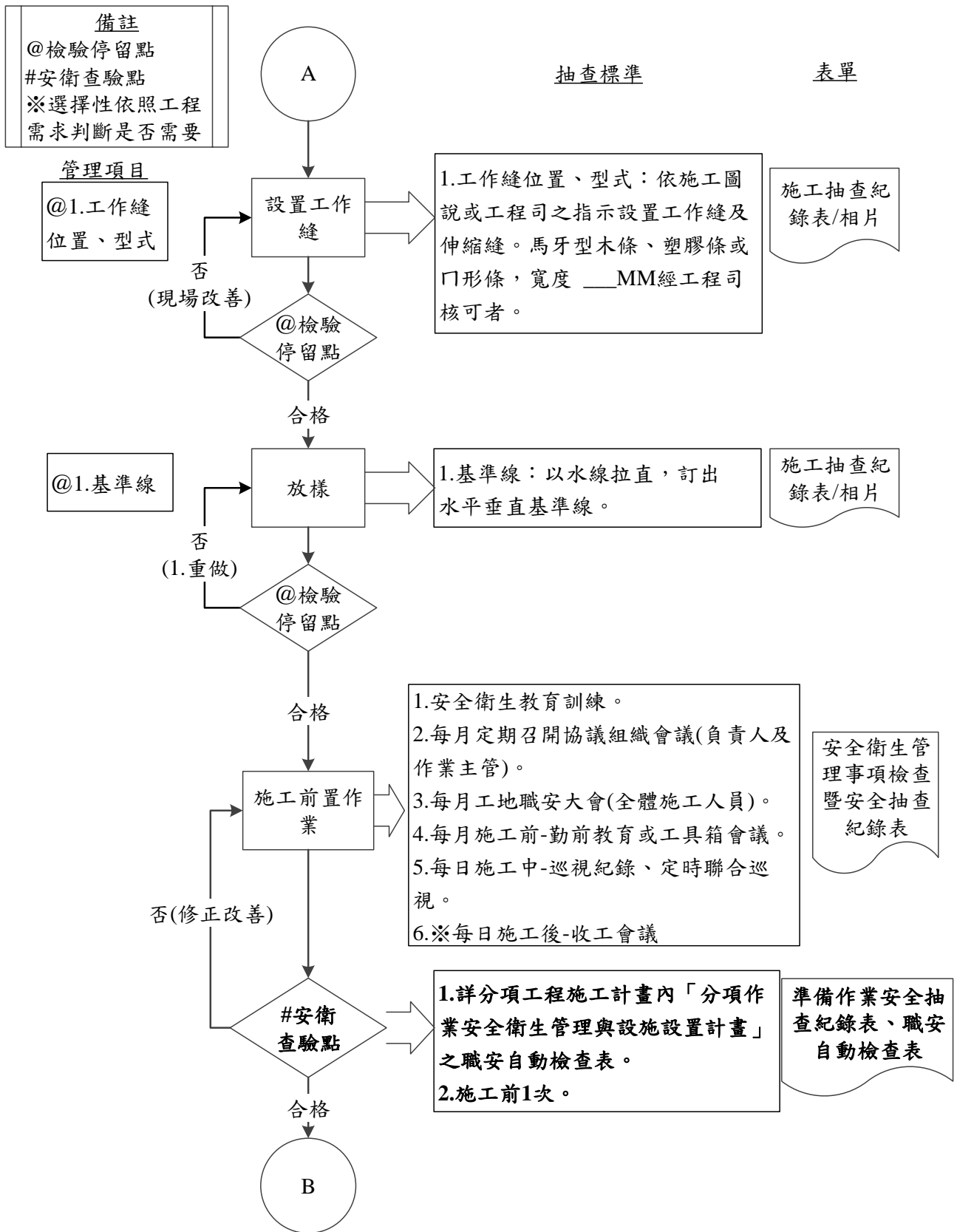
圖 097810-F-1 新石子工程施工抽查流程圖 2/4
