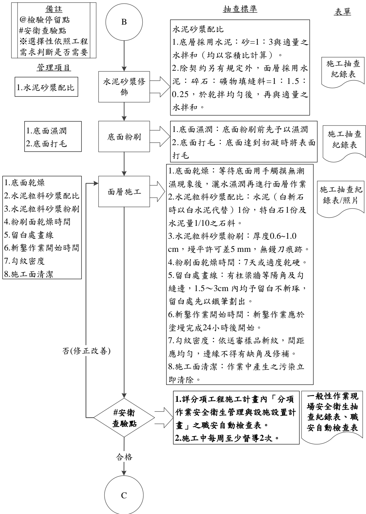
圖 097810-F-1 斬石子工程施工抽查流程圖 3/4
