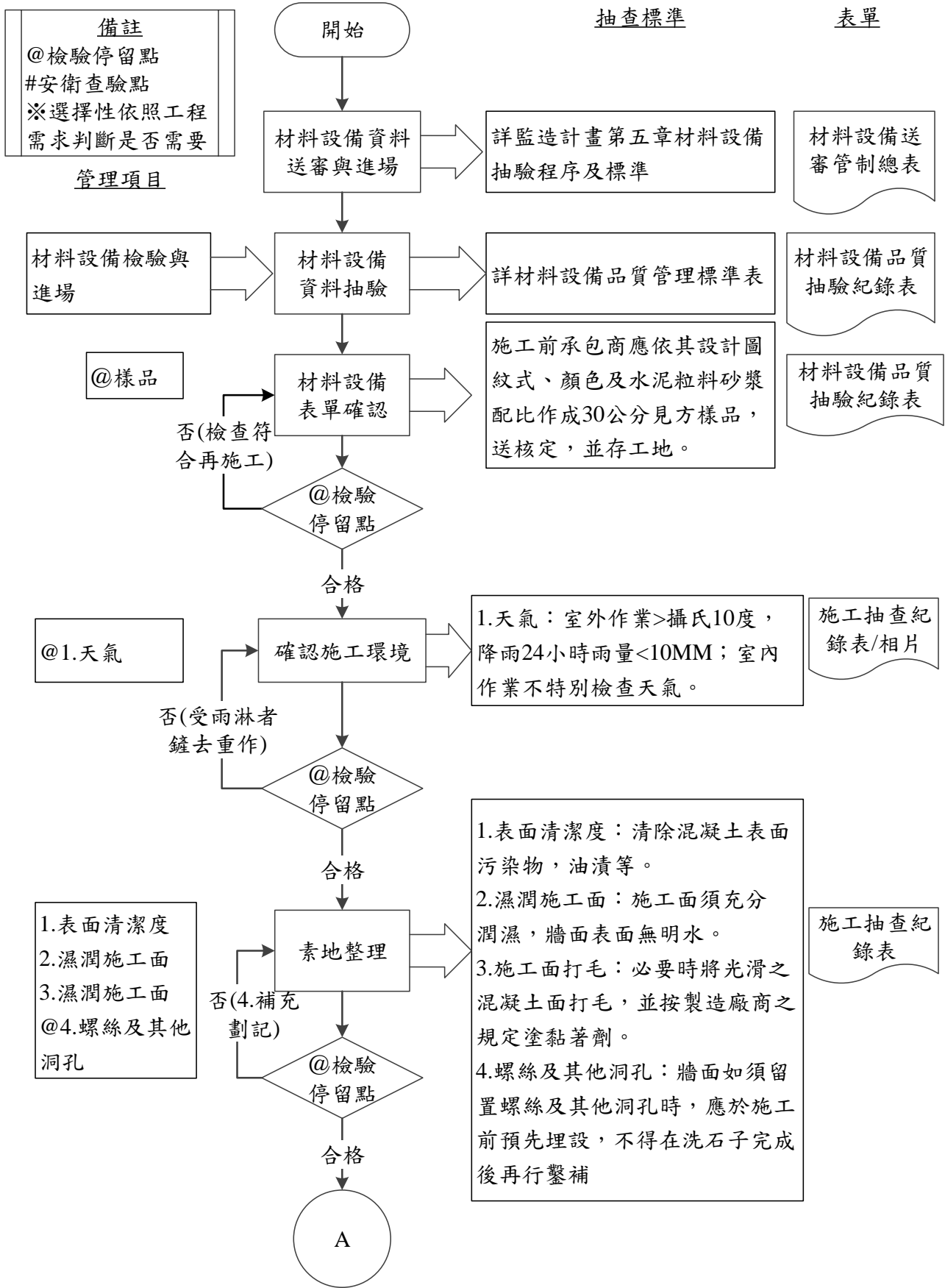
圖 097810-F-1 斬石子工程施工抽查流程圖 1/4
