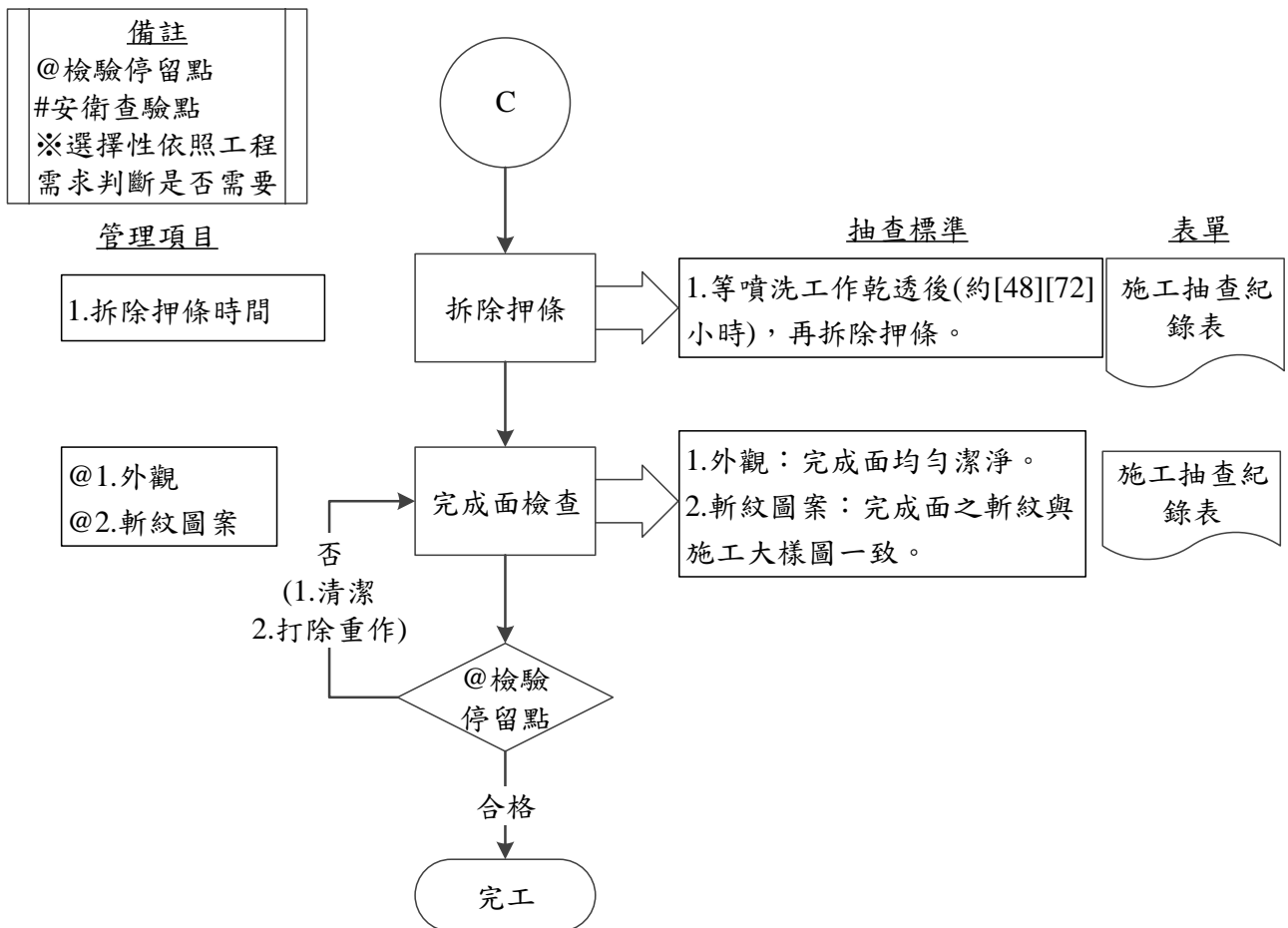
圖 097810-F-1 斬石子工程施工抽查流程圖 4/4
