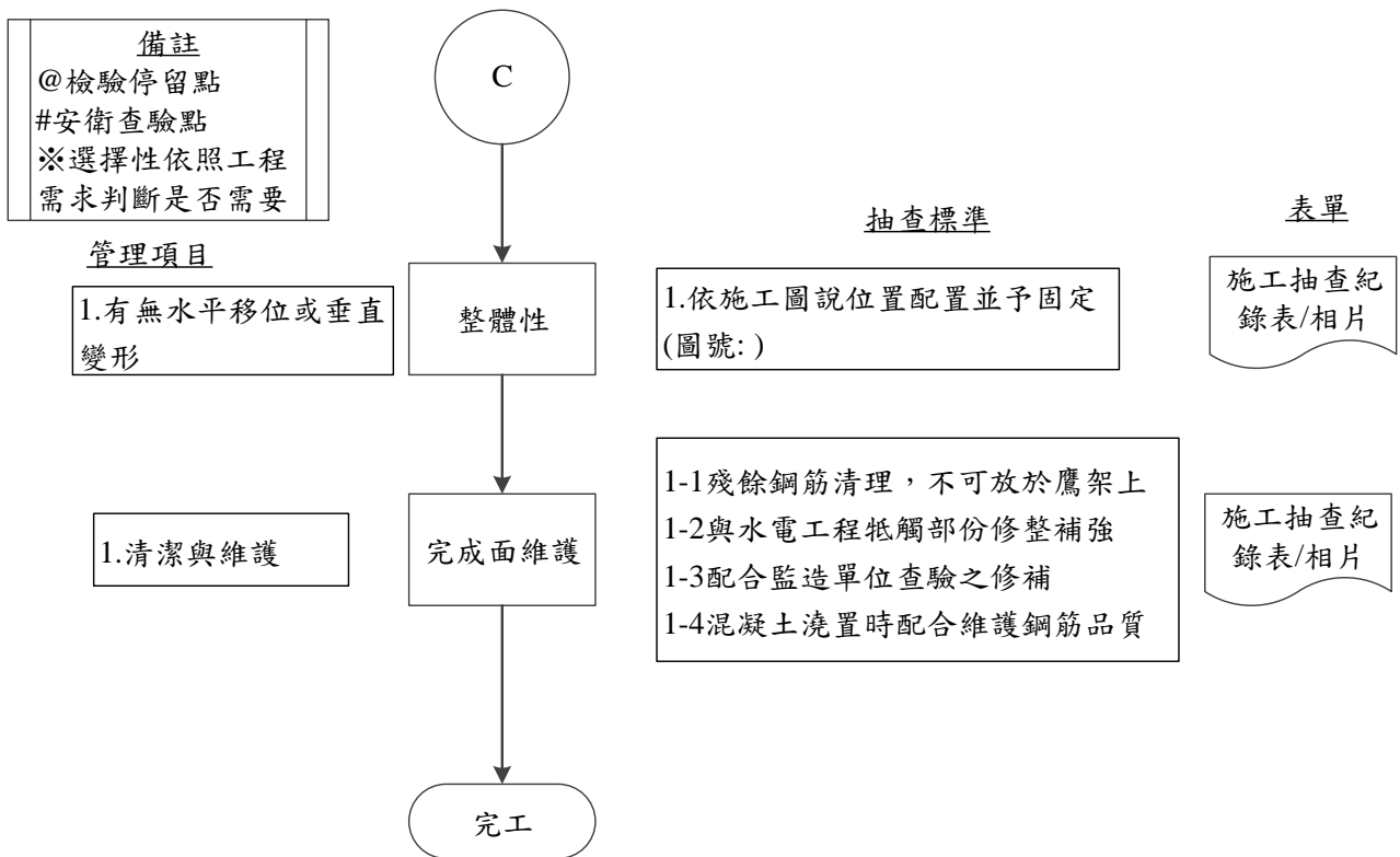
圖 032101-F-1 建築物鋼筋工程施工抽查流程圖 4/4
