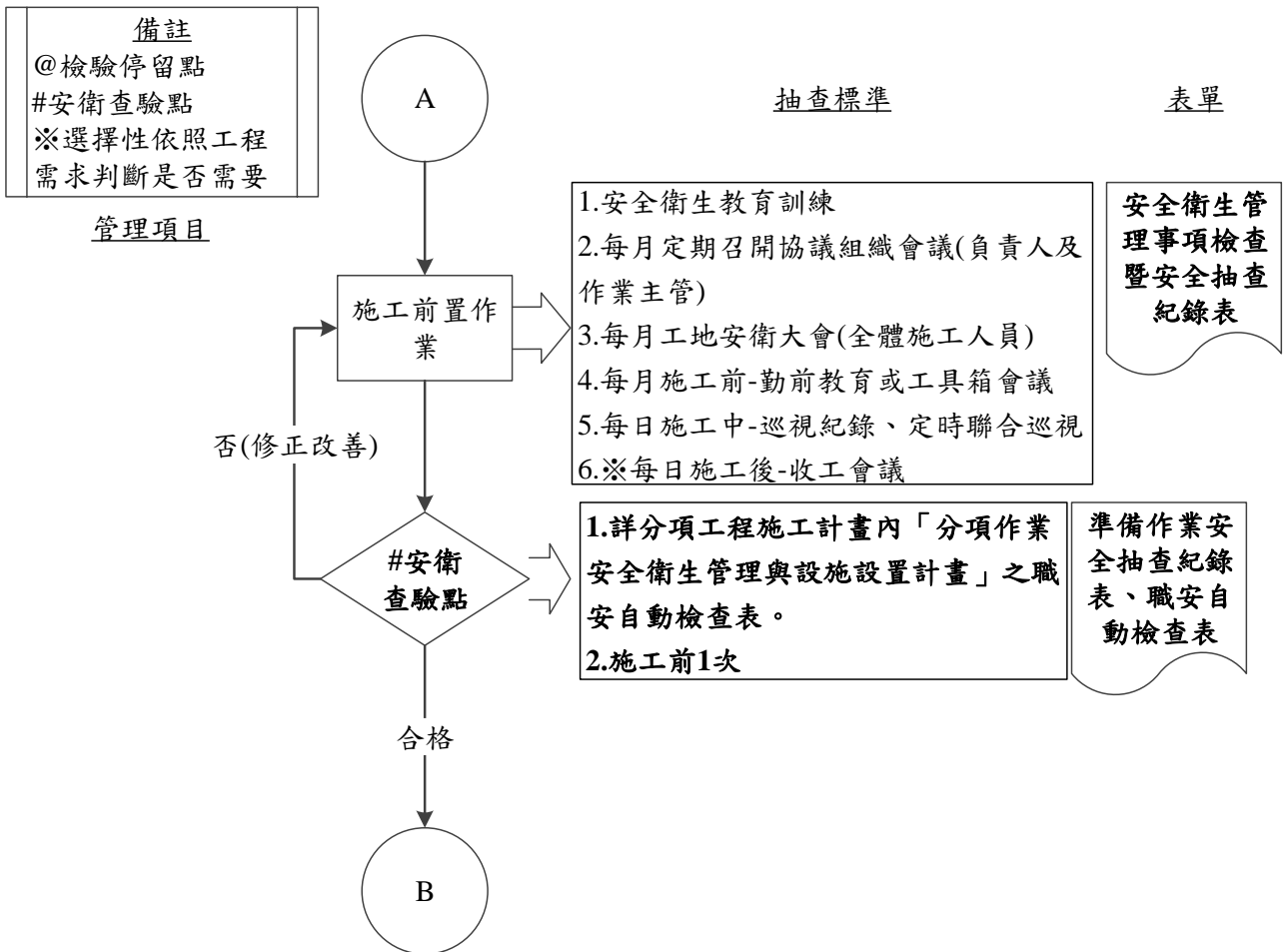
圖 032101-F-1 建築物鋼筋工程施工抽查流程圖 2/4
