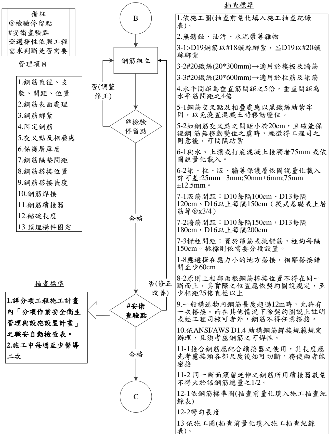
圖 032101-F-1 建築物鋼筋工程施工抽查流程圖 3/4
