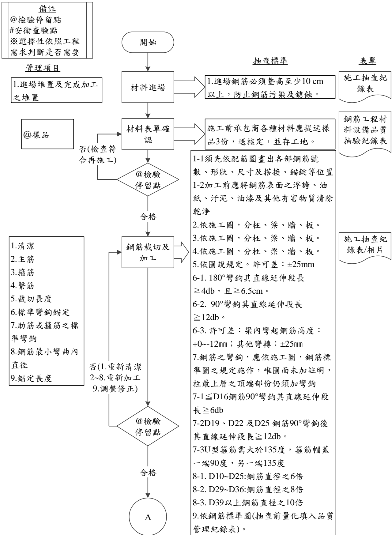
圖 032101-F-1 建築物鋼筋工程施工抽查流程图 1/4
