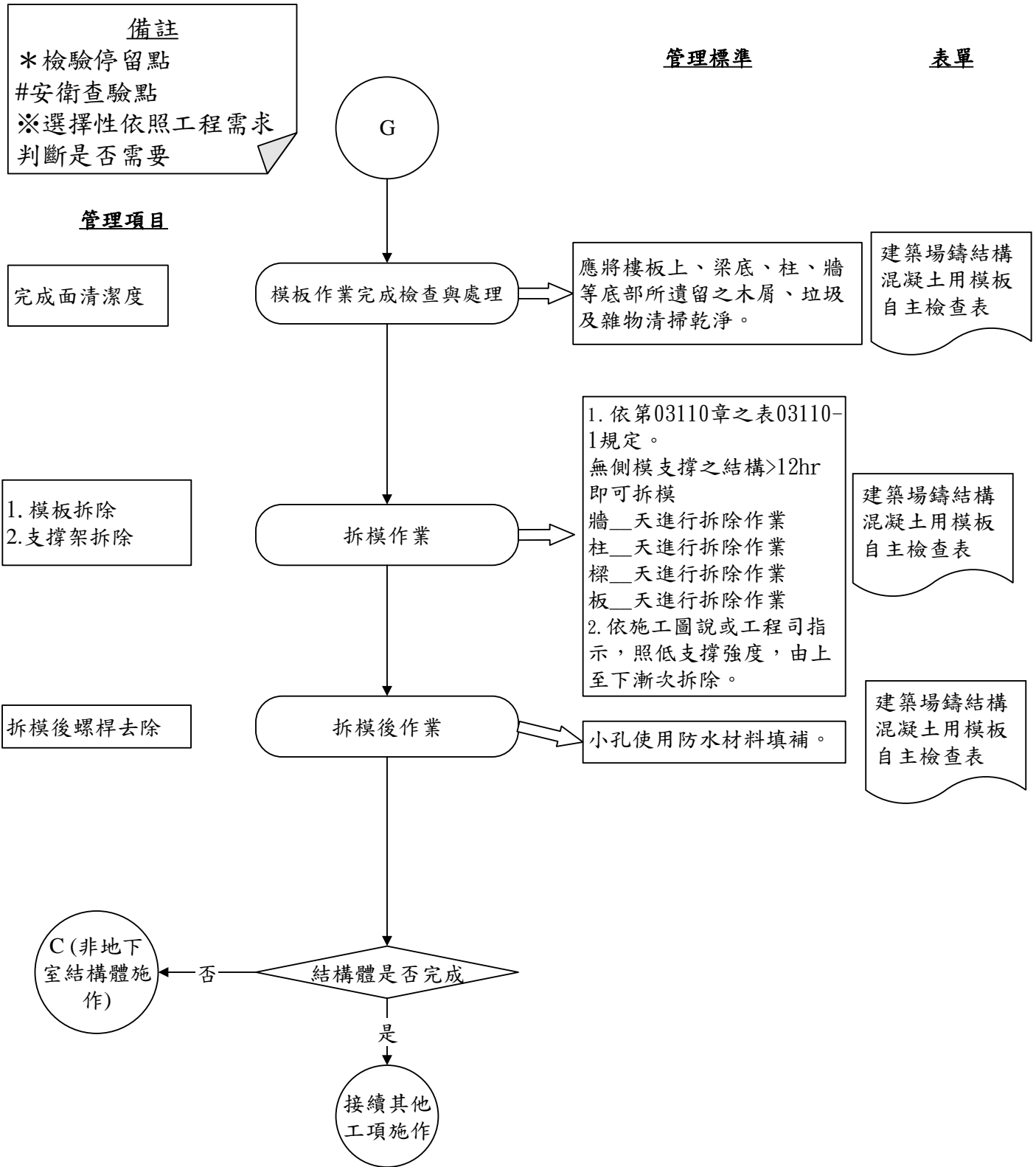
圖 031103-QCF-8 建築場鑄結構混凝土用模板工程施工檢驗流程圖 8/8
