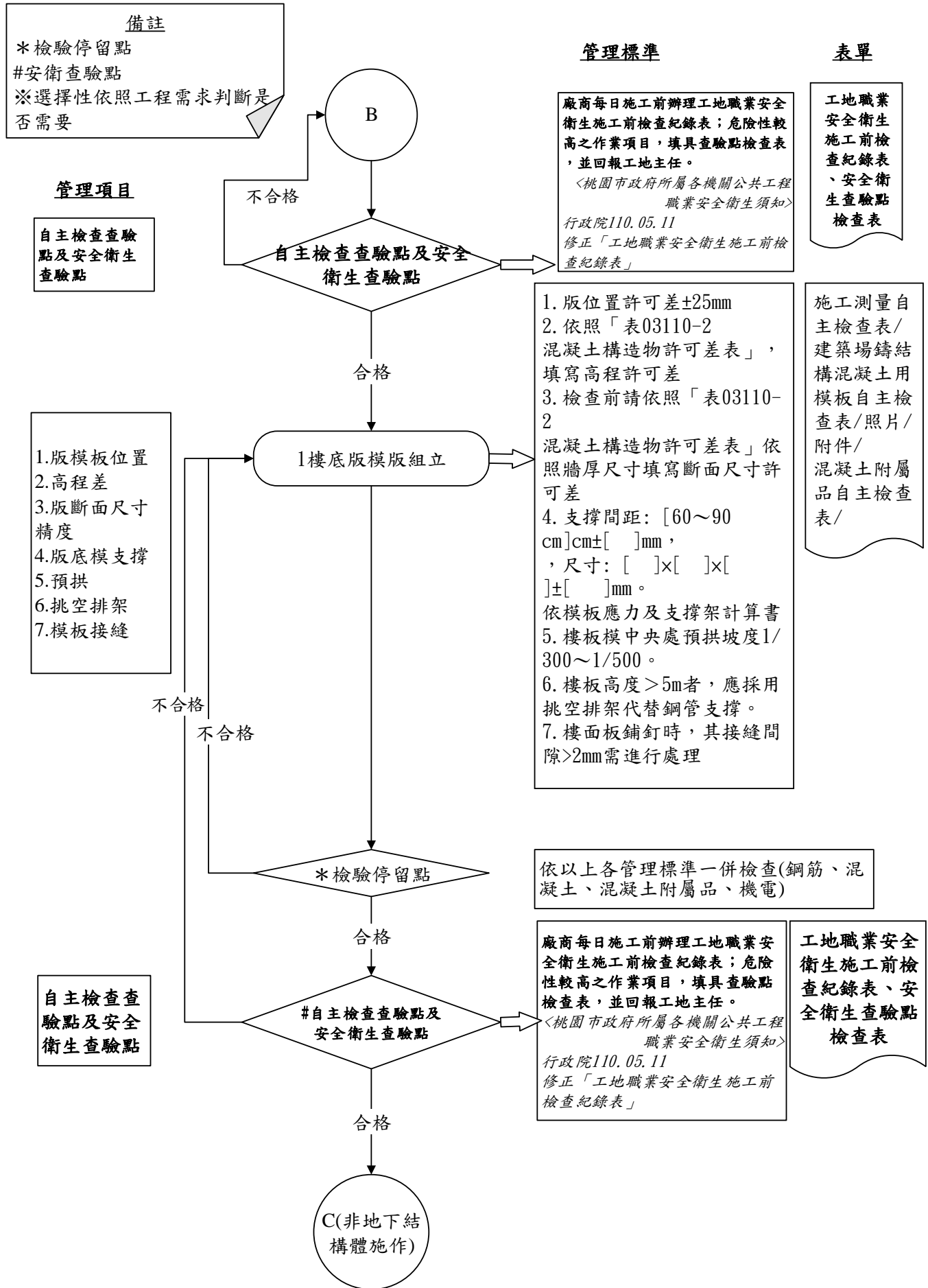
圖 031103-QCF-3 建築場鑄結構混凝土用模板工程施工檢驗流程圖 3/8
