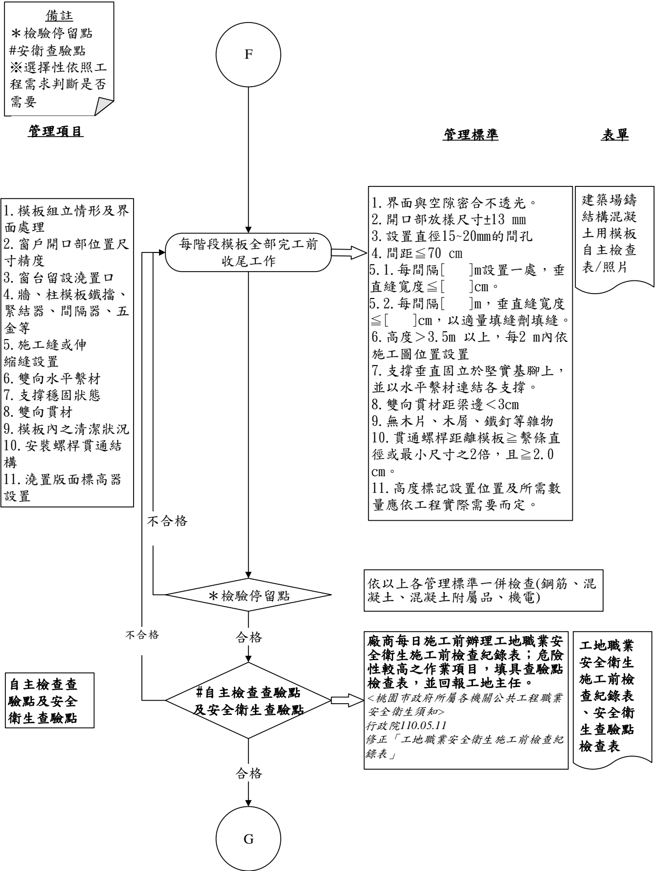
圖 031103-QCF- 7 建築場鑄結構混凝土用模板工程施工檢驗流程圖 7/8
