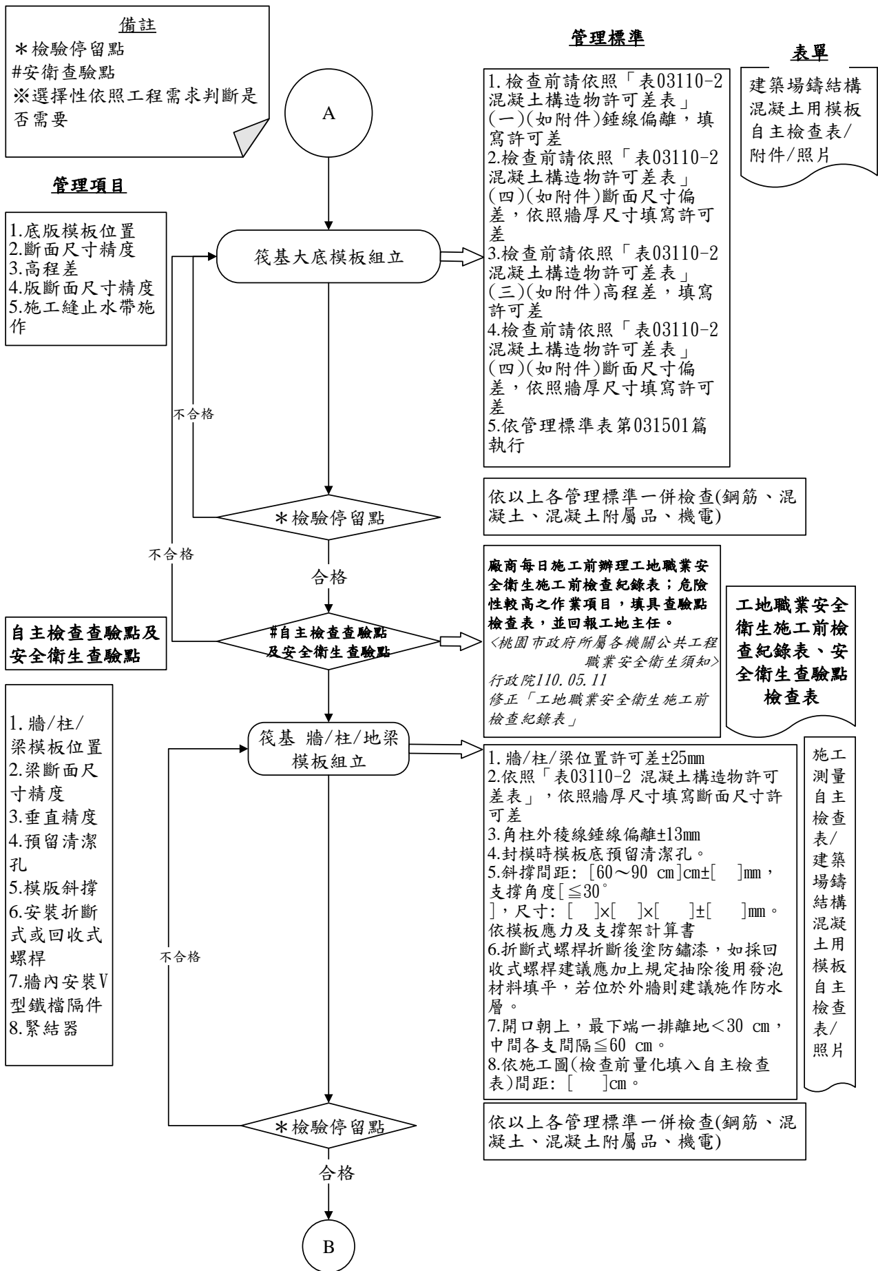
圖 031103-QCF-2 建築場鑄結構混凝土用模板工程施工檢驗流程圖 2/8
