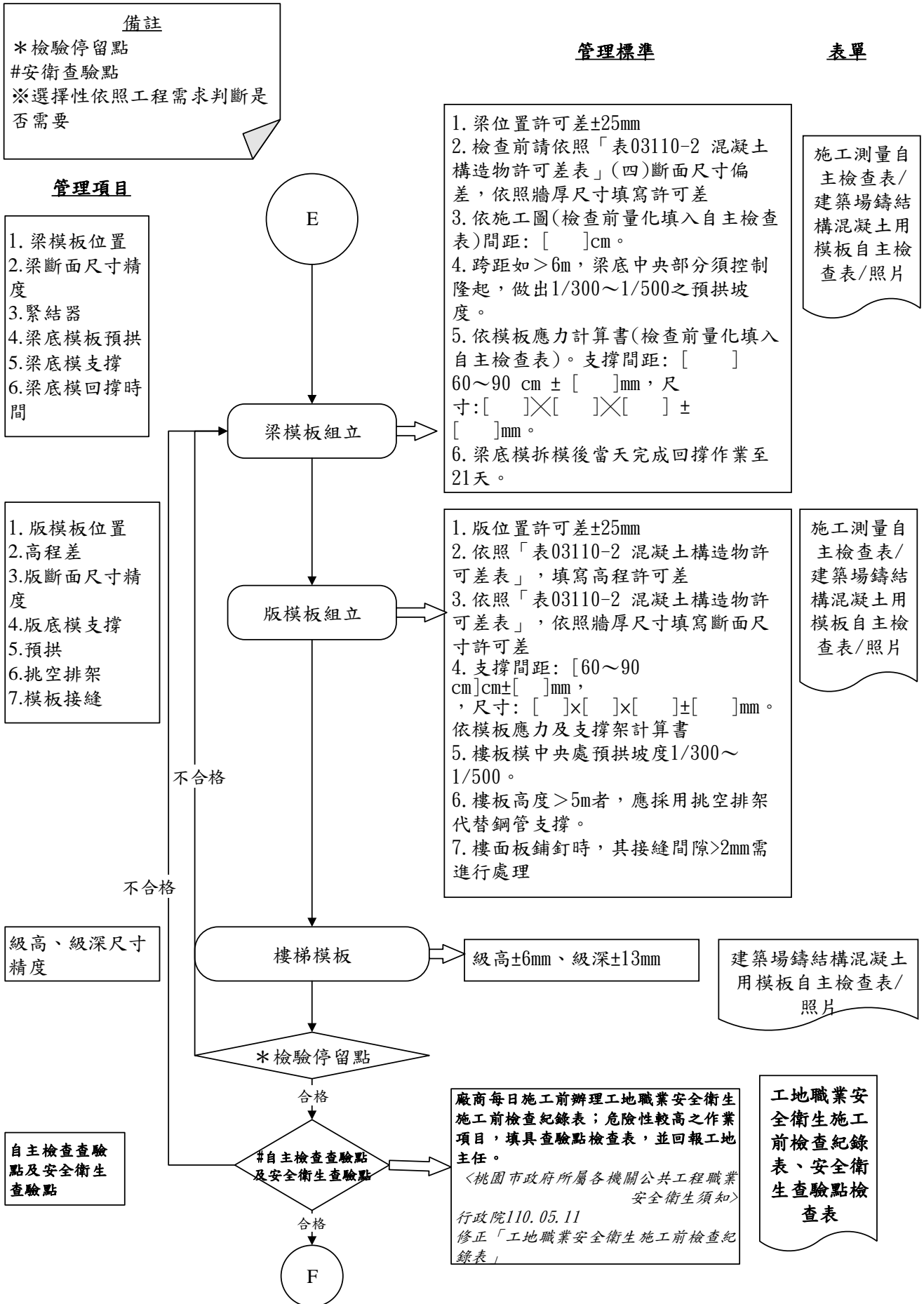
圖 031103-QCF-6 建築場鑄結構混凝土用模板工程施工檢驗流程圖 6/8
