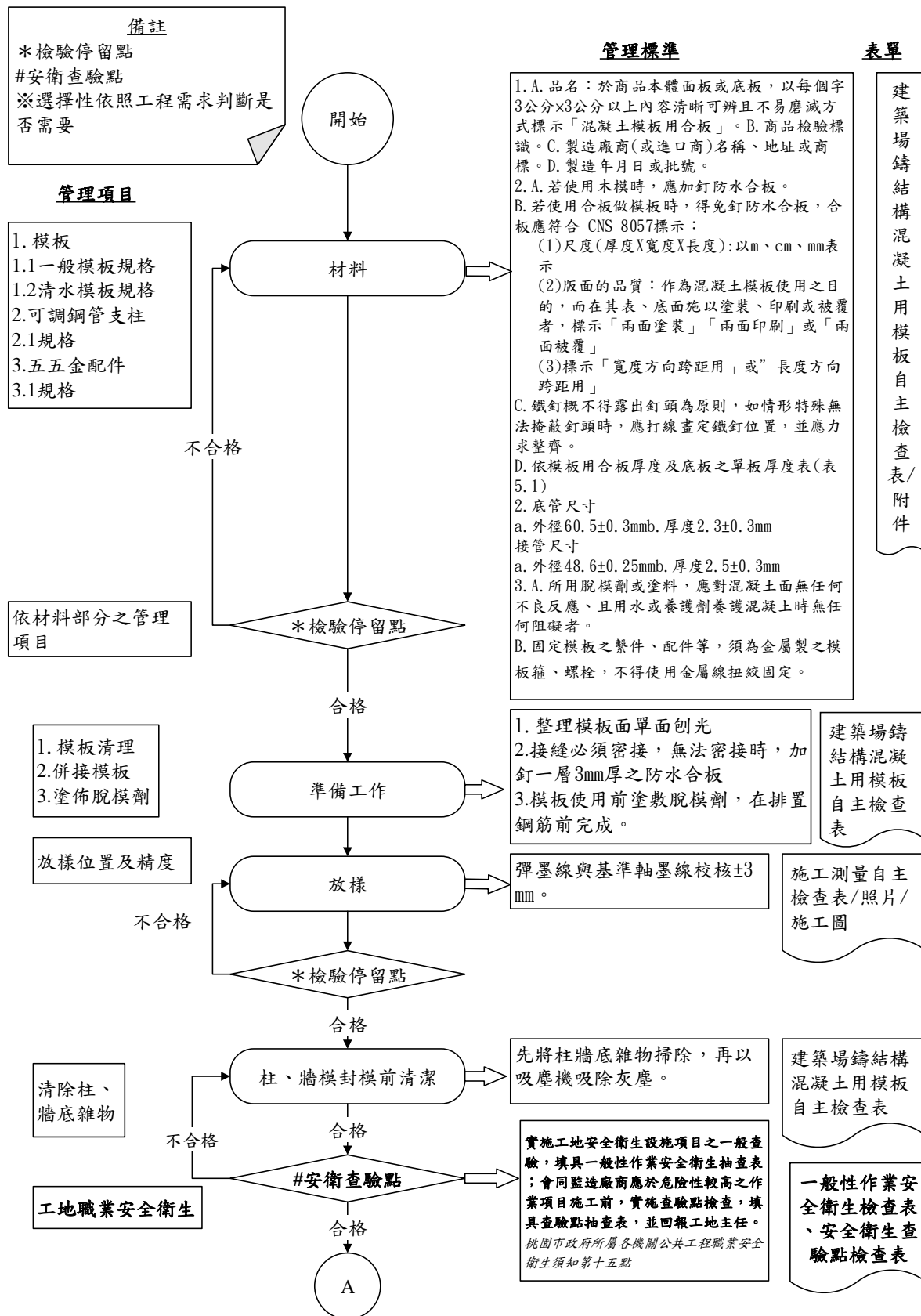
圖 031103-QCF-1 建築場鑄結構混凝土用模板工程施工檢驗流程圖 1/8
