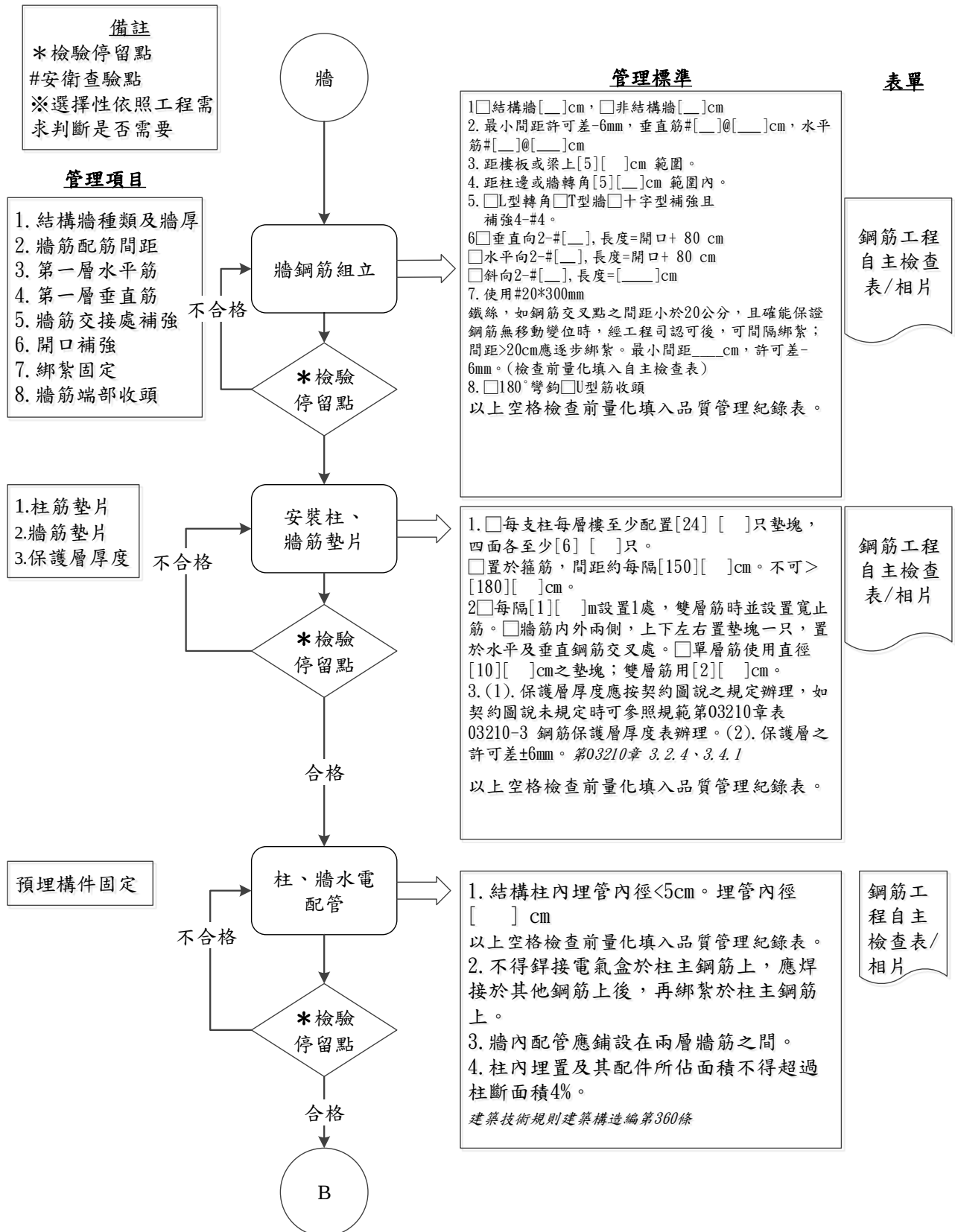
圖 032101-QCF-1 鋼筋工程施工檢驗流程圖 4/7
