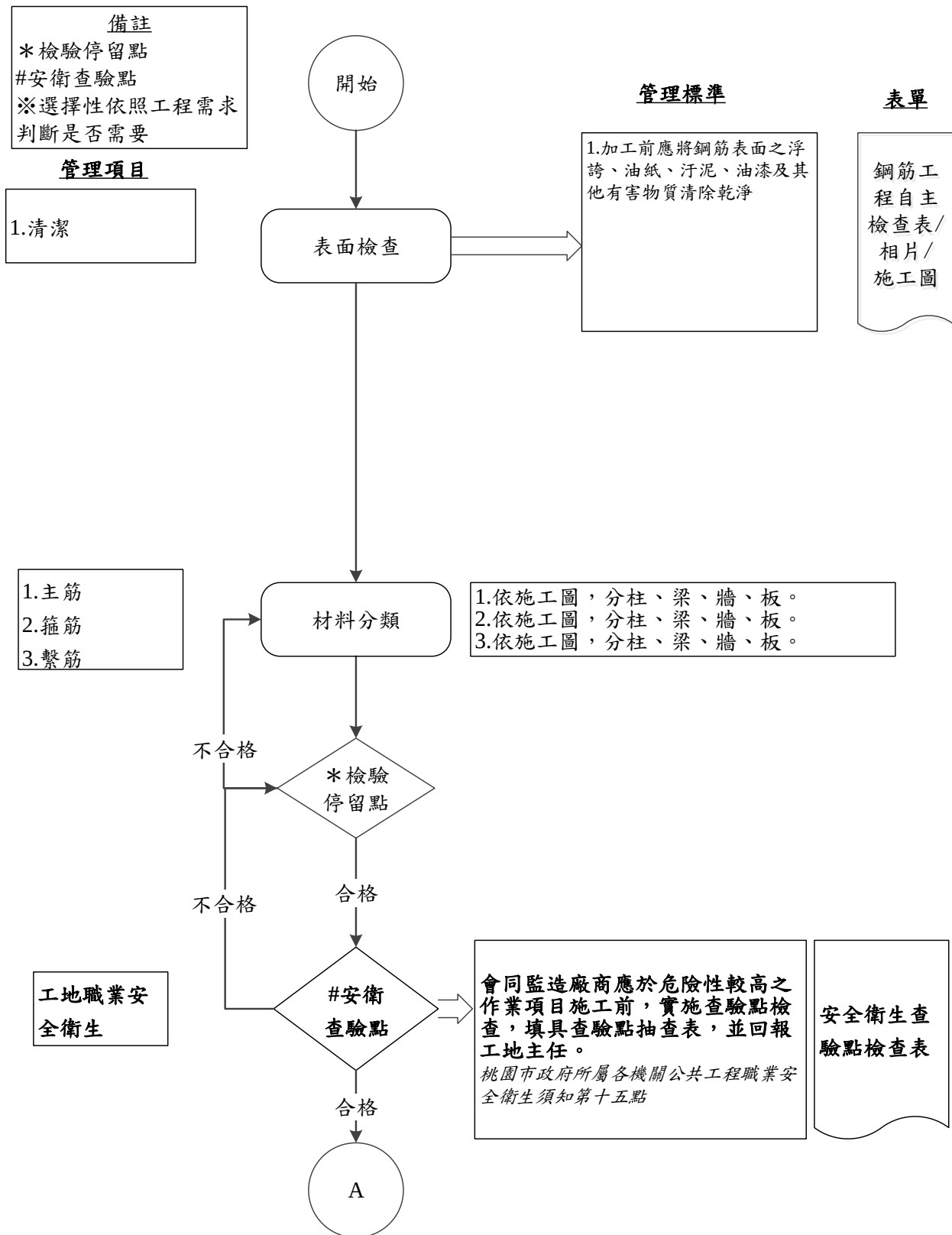
圖 032101-QCF-1 鋼筋工程施工檢驗流程圖 1/7
