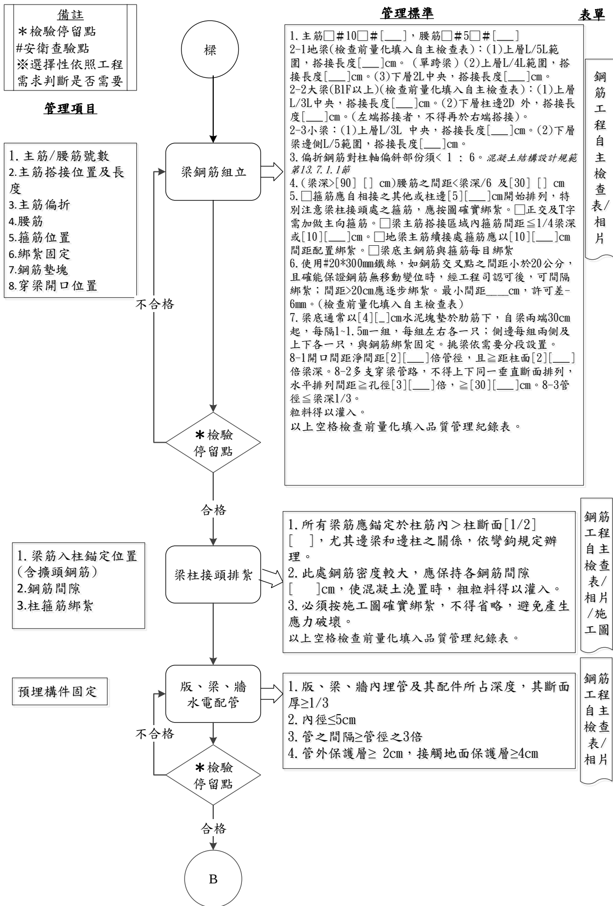
圖 032101-QCF- 1 鋼筋工程施工檢驗流程圖 5/7
