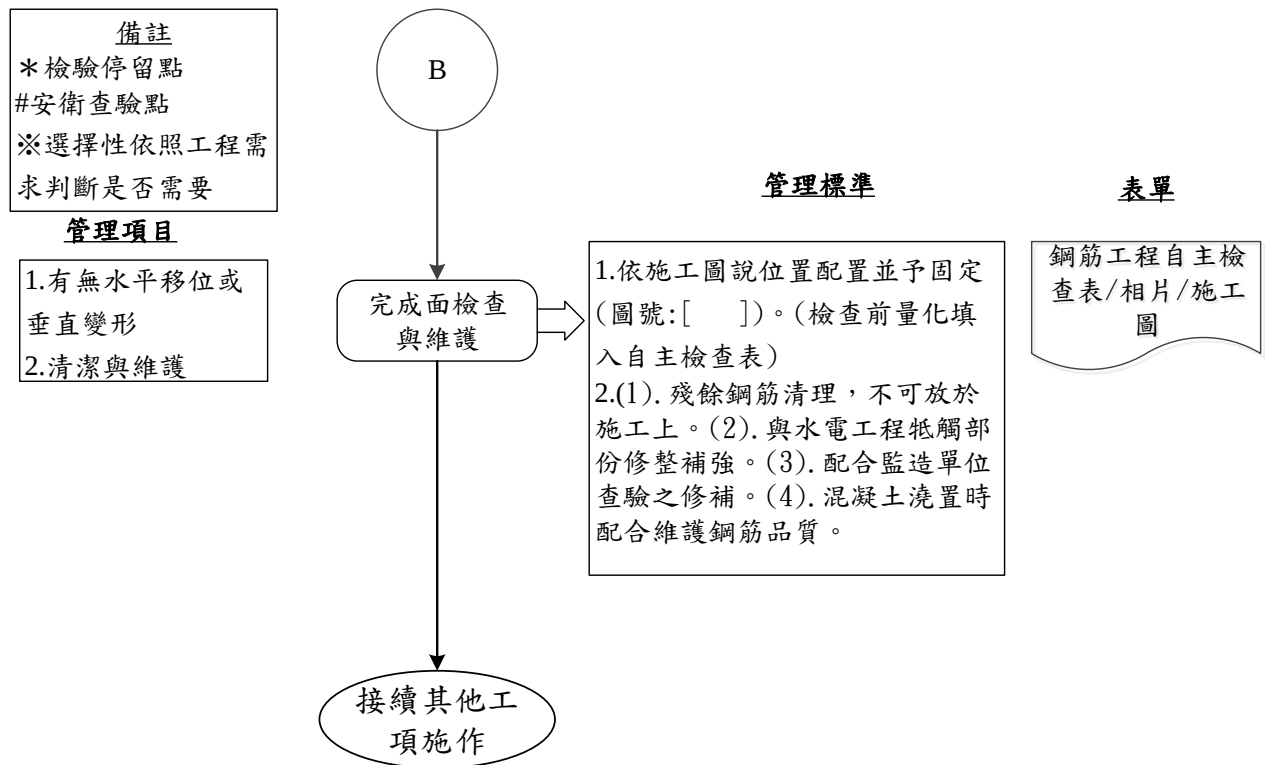
圖 032101-QCF- 1 鋼筋工程施工檢驗流程圖 7/7
