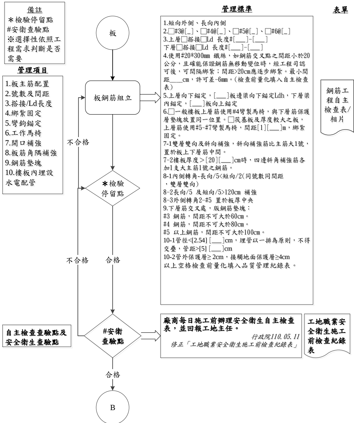
圖 032101-QCF-1 鋼筋工程施工檢驗流程圖 6/7
