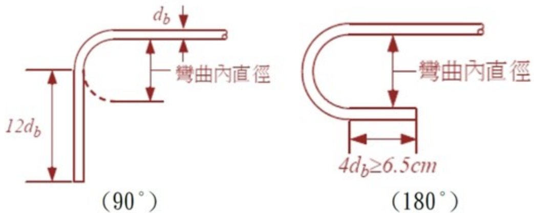
圖 03210- 主鋼筋之標準彎鉤
