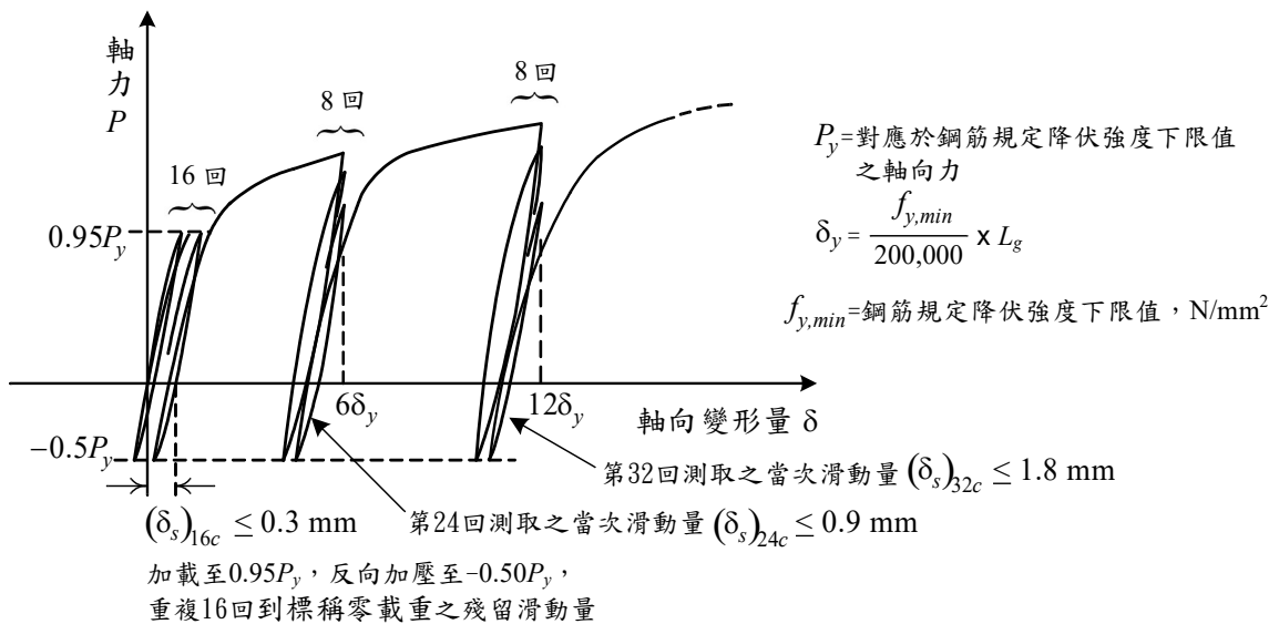
圖四 續接試體高塑性反復負載試驗加載程式示意圖
