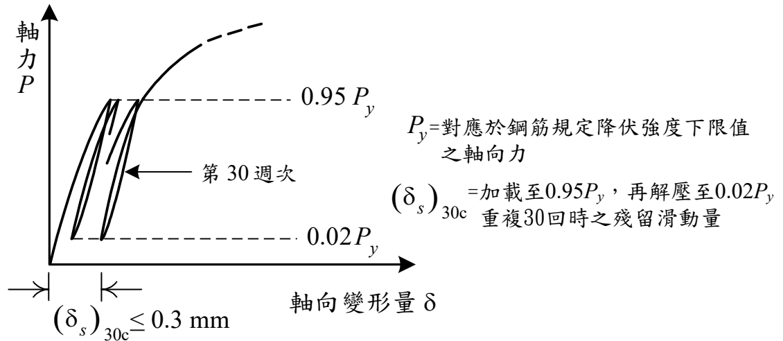
圖三 續接試體重復負載及滑動試驗加載程式示意圖
