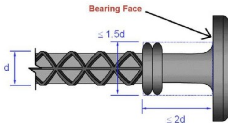
圖 03210- 主鋼筋之擴頭竹節鋼筋
