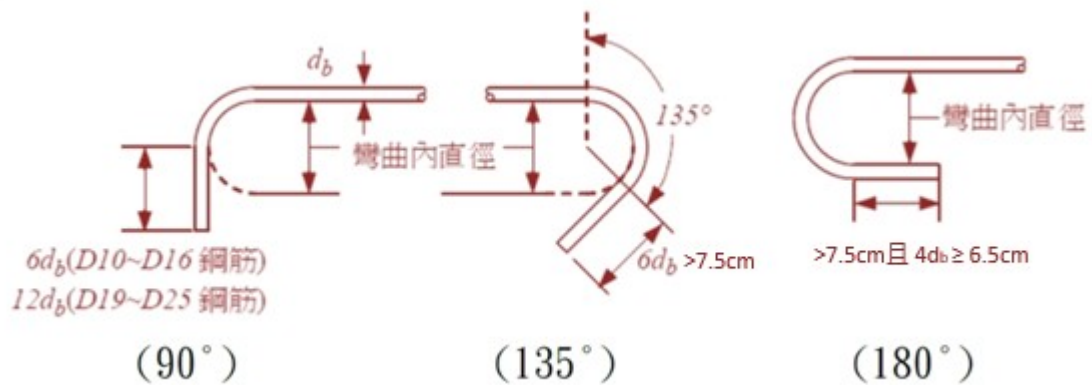
圖 03210- 肋筋及箍筋標準彎鉤
